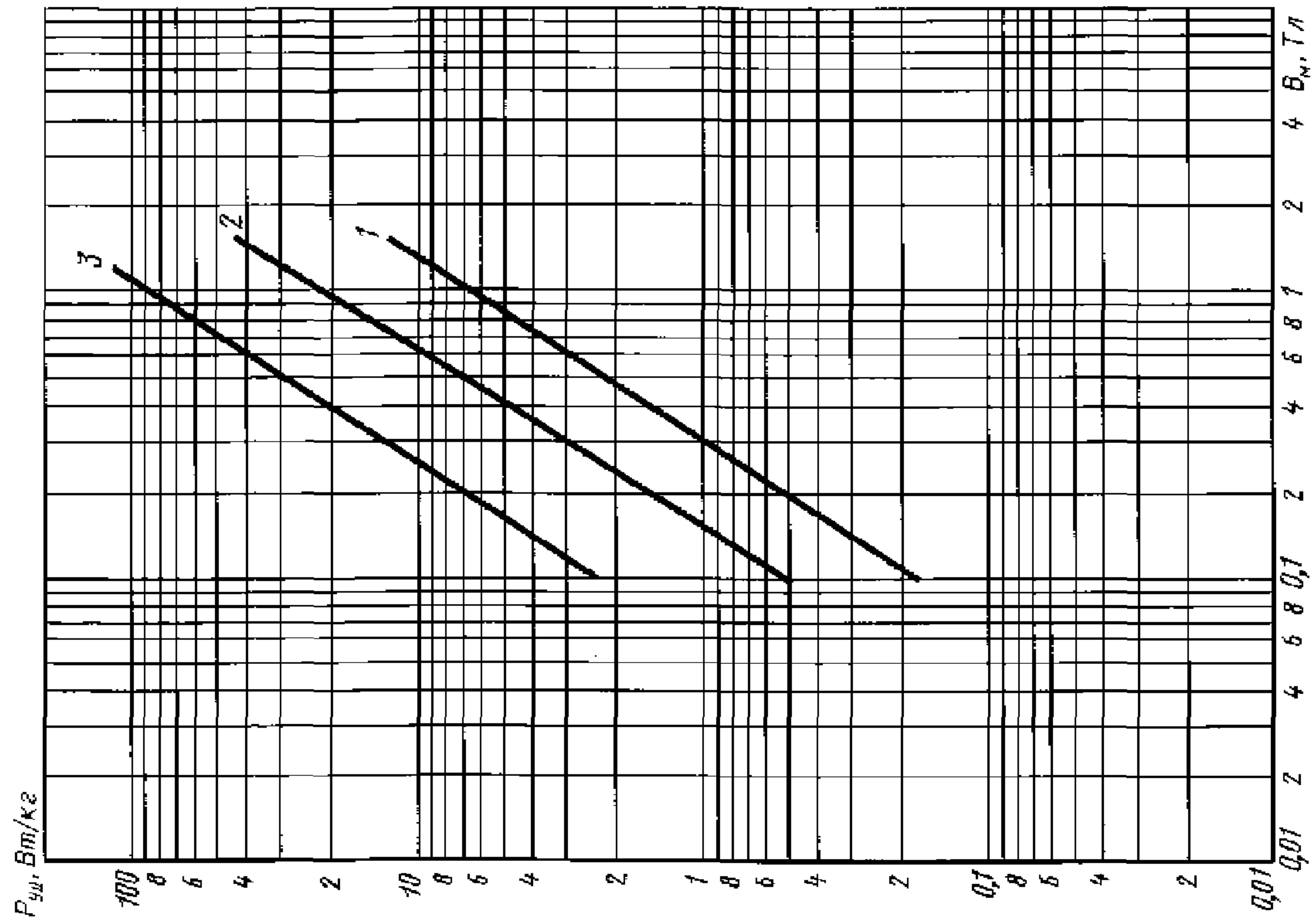
Зависимость удельных потерь от индукции для стали марки 3425 (Э360АА) при частоте: 1 — 400 Гц, 2 — 1000 Гц, 3 — 3000 Гц
