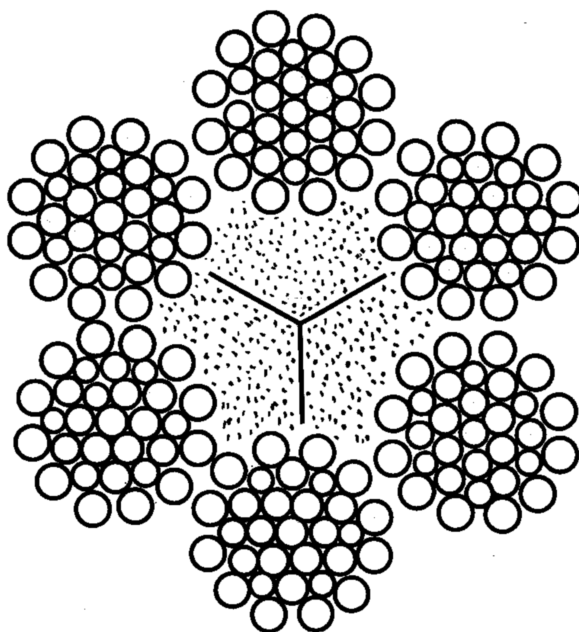
Шестипрядный канат 6×31+1 о. с.; 6×31=186 проволок с органическим сердечником (прясть каната 1+6+6/6+12).
