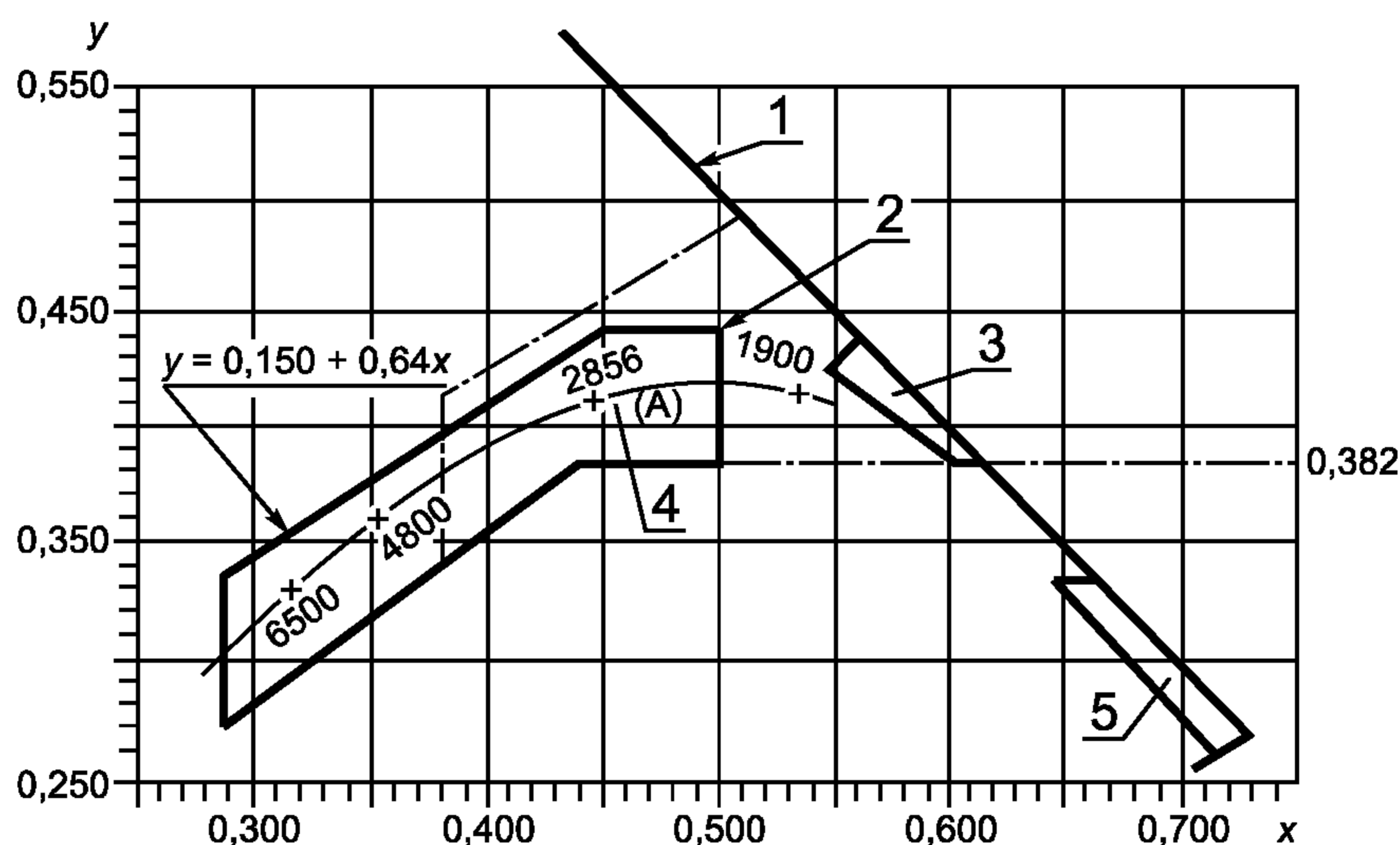
Границы световых участков для световозвращающих устройств
