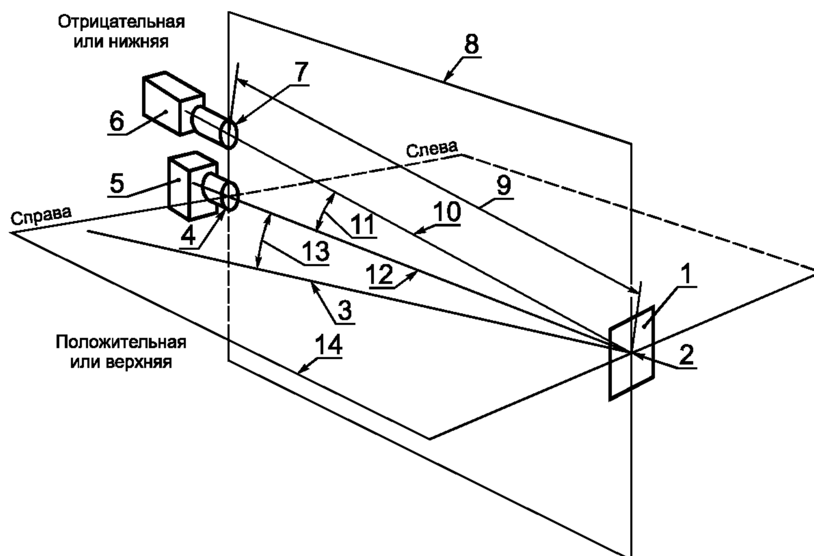
Установка оборудования для испытания световозвращателя
