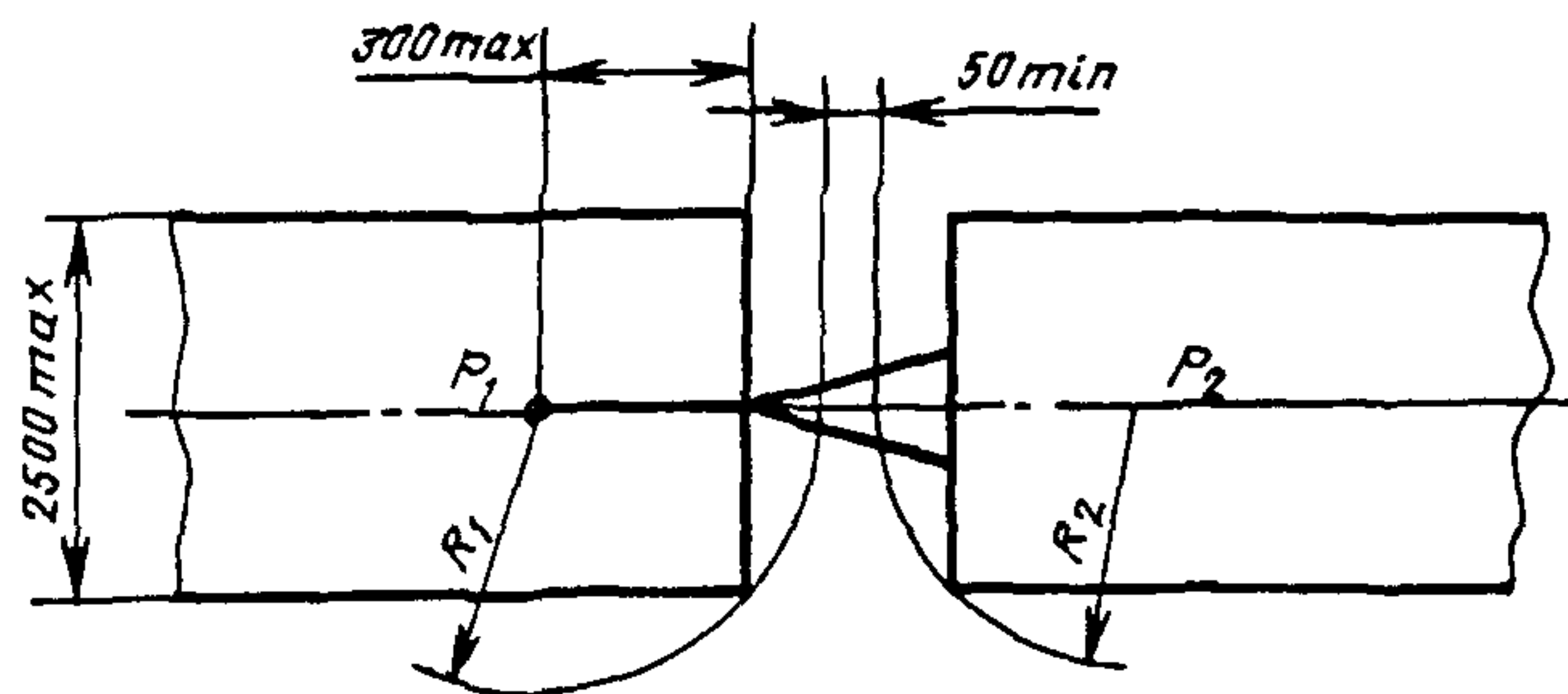
R_1 — радиус габарита задней части тягача (прицепа или полуприцепа для многозвенного автопоезда); R_2 — радиус габарита передней части прицепа; P_1 — центр тягово-сцепного устройства; P_2 — центр поворотного устройства
