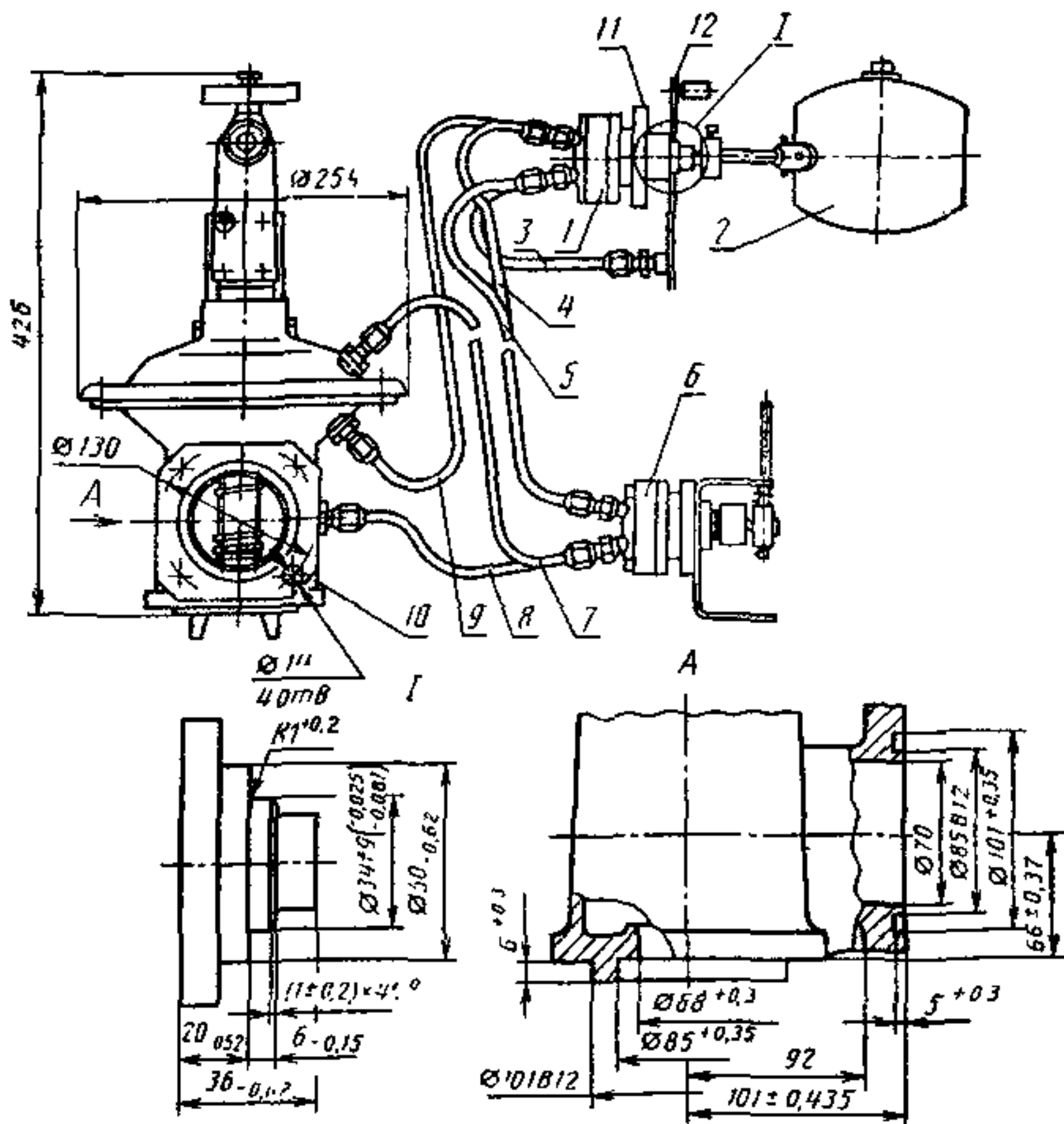
1 — кран золотниковый; 2 — цистерма; 3, 4, 5, 7, 8, 9 — соединительные магистрали; 6 — кран управления; 10 — гидроклапан; 11 — фланец; 12 — горловина цистермы
