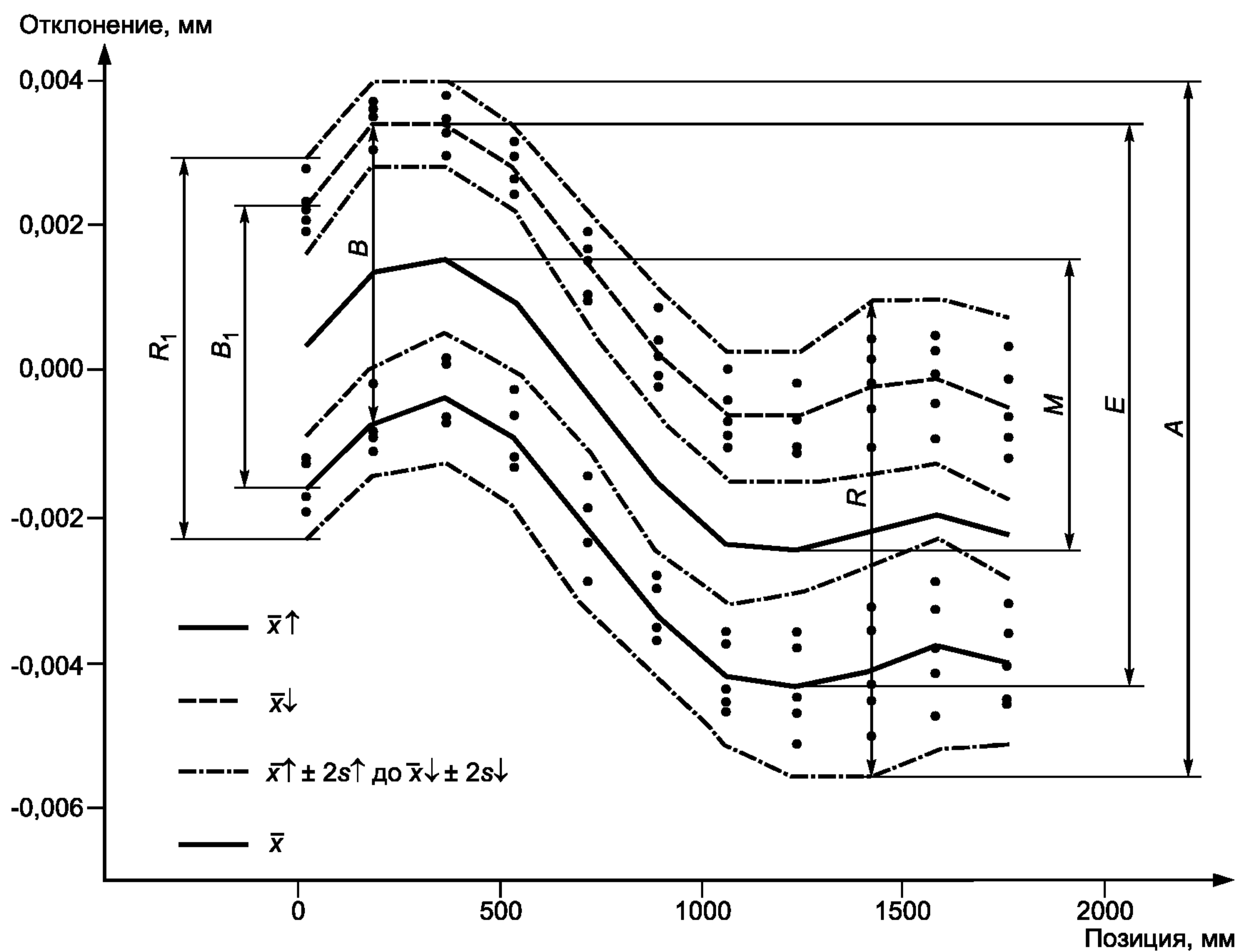
Рисунок А.1 — Точность и повторяемость двустороннего позиционирования
