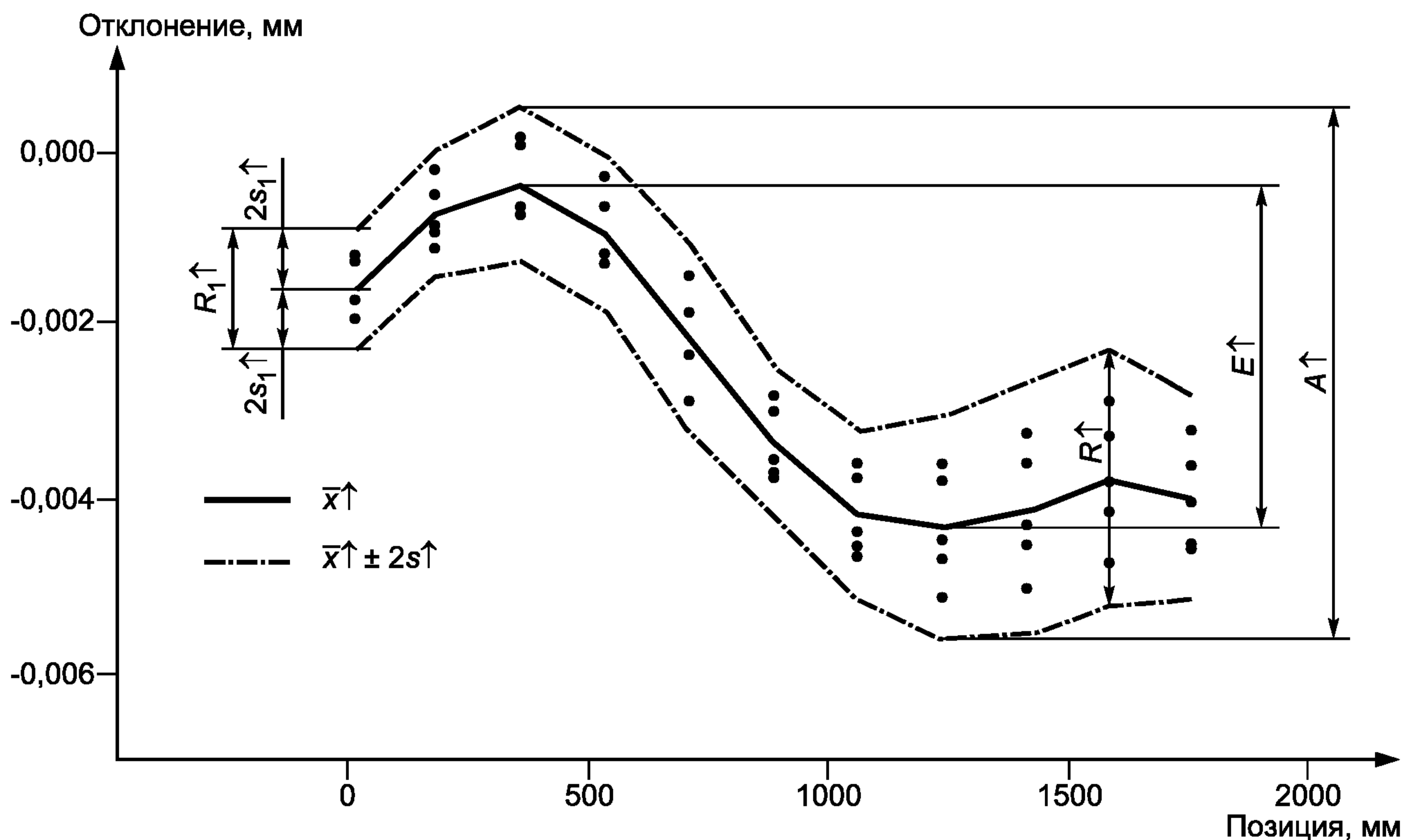
Рисунок А.2 — Точность и повторяемость одностороннего позиционирования
