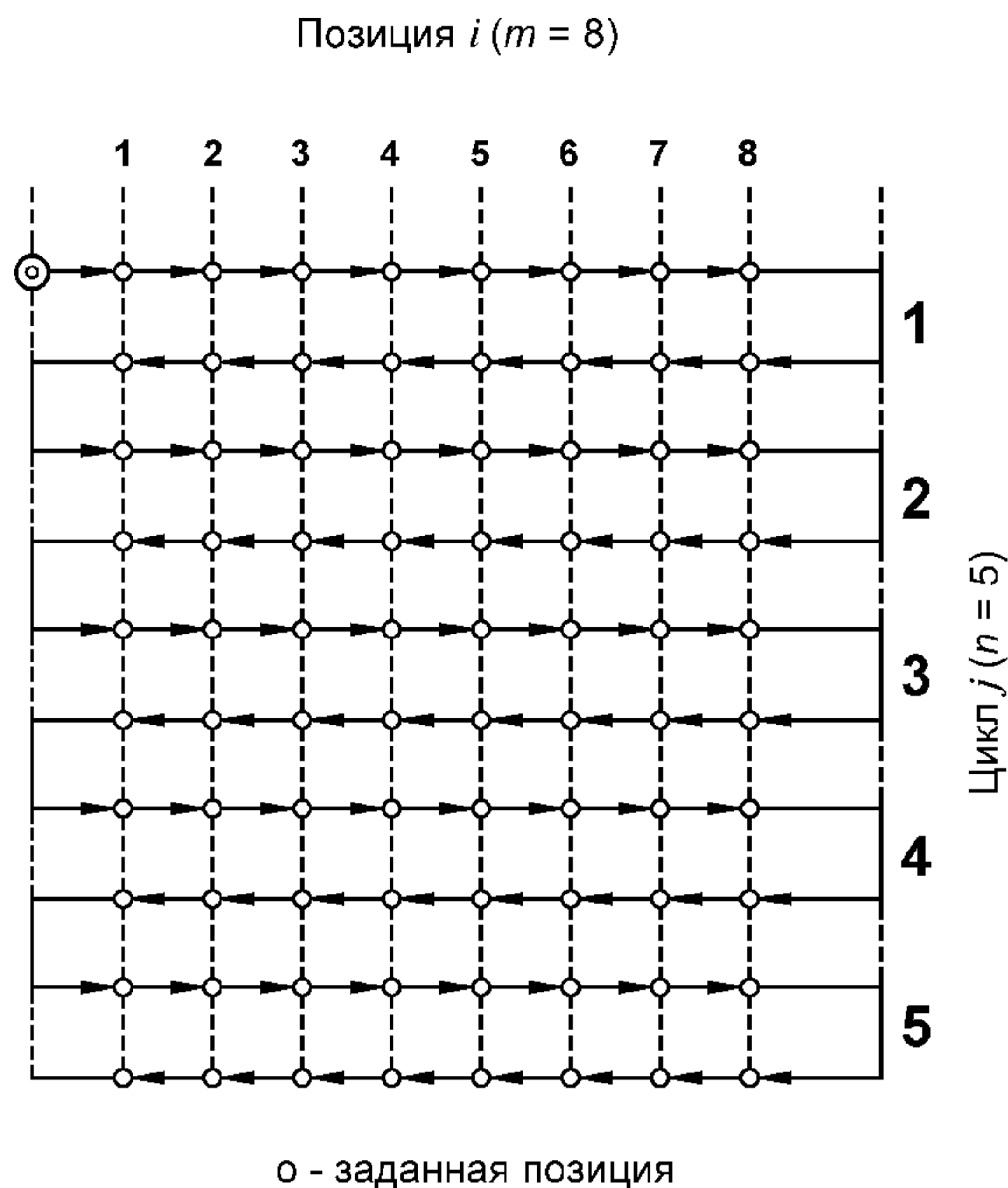
Рисунок 1 — Стандартный цикл измерений
