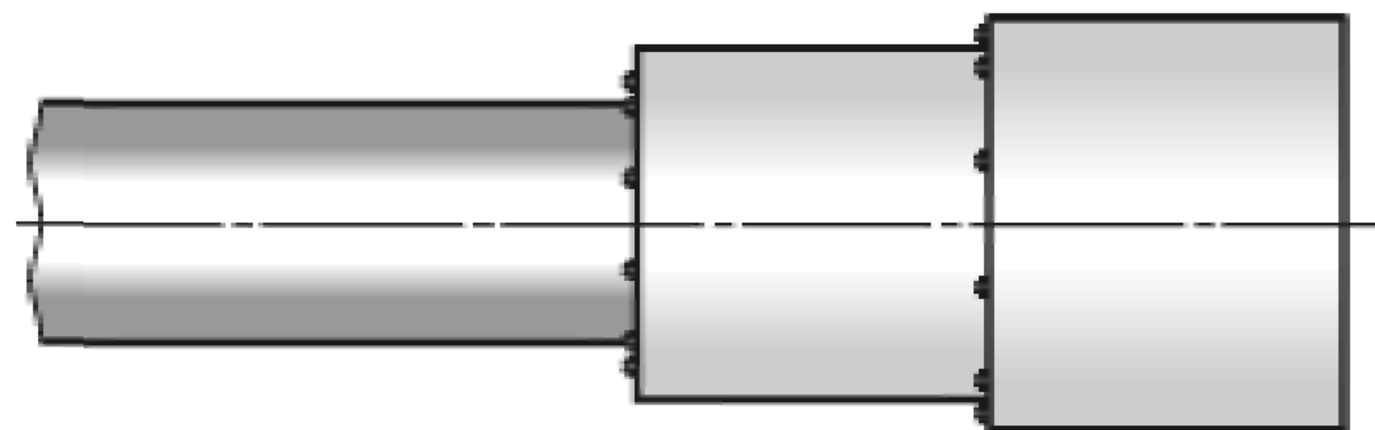
Рисунок D.2 — Двойной канальный глушитель
