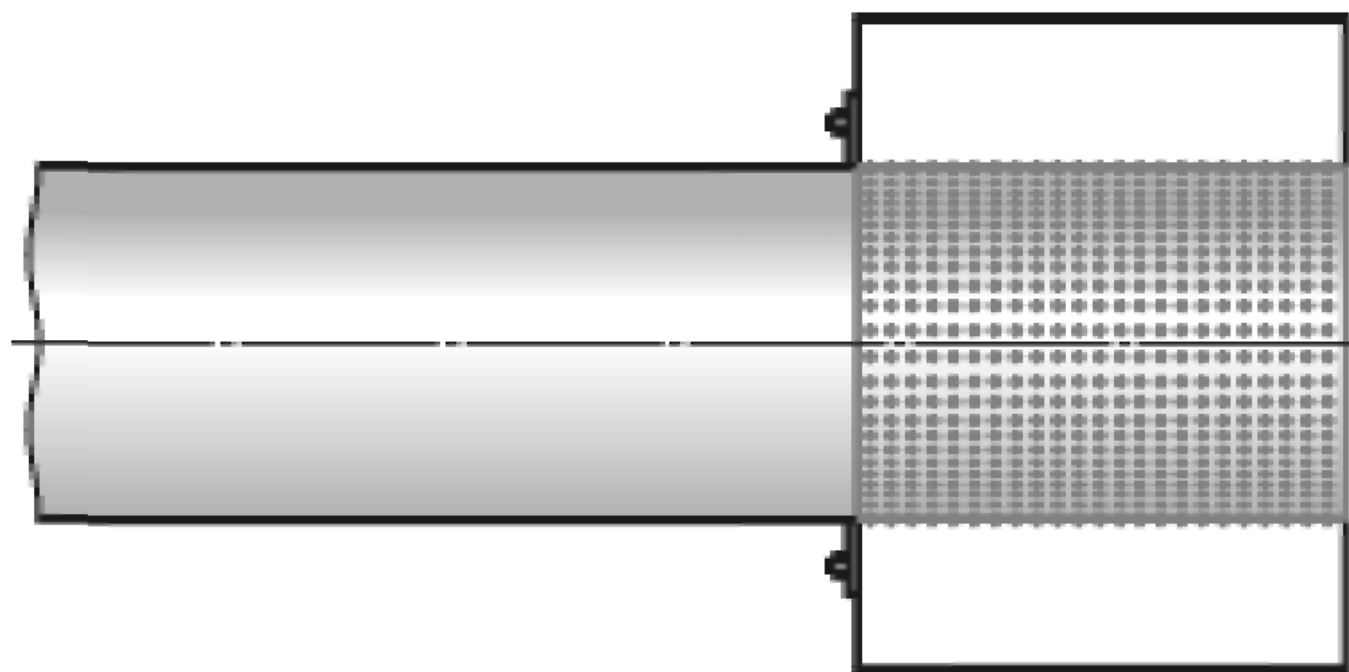
Рисунок D.1 — Канальный глушитель (разрез)
