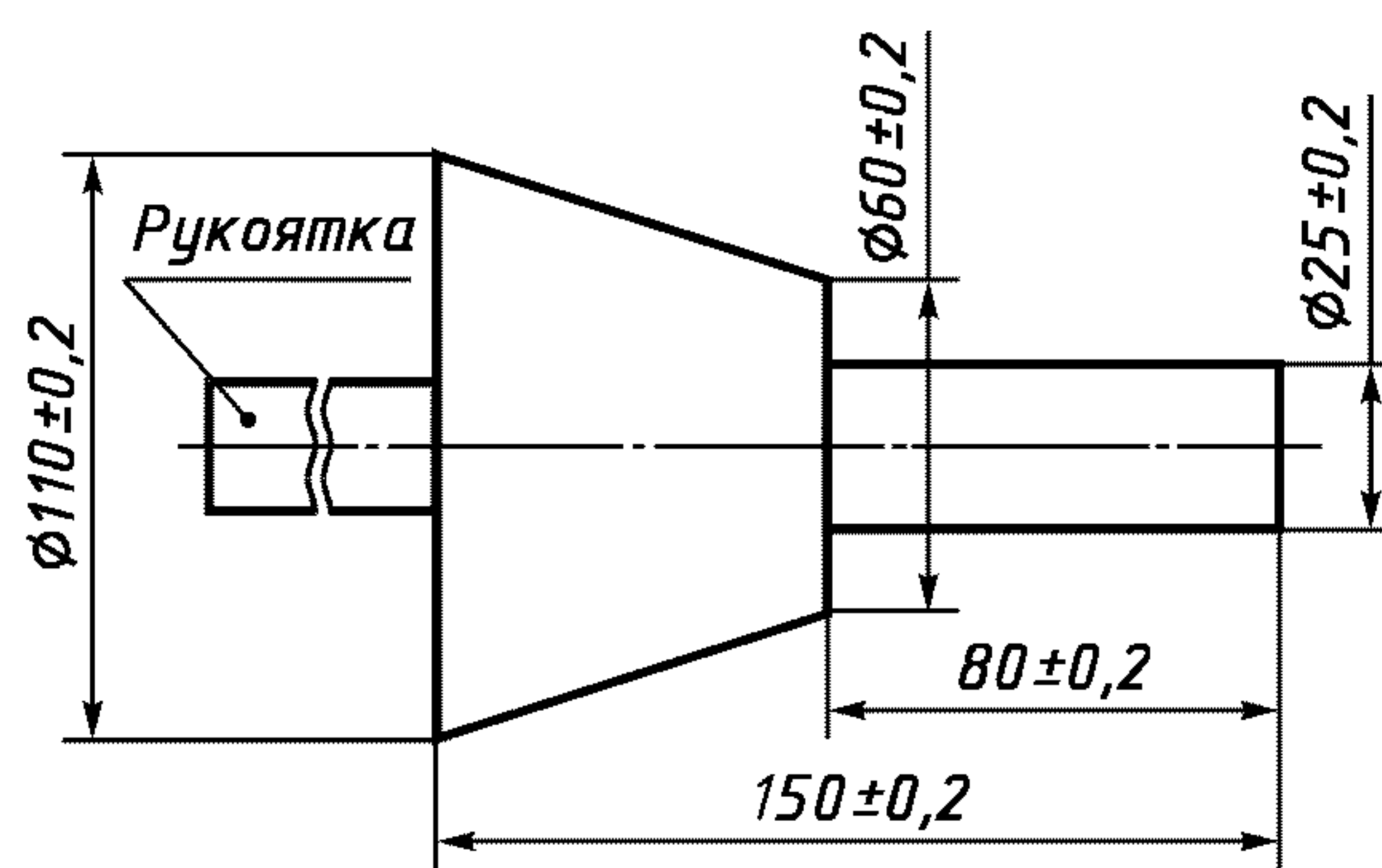
Рисунок 101 — Испытательный калибр
