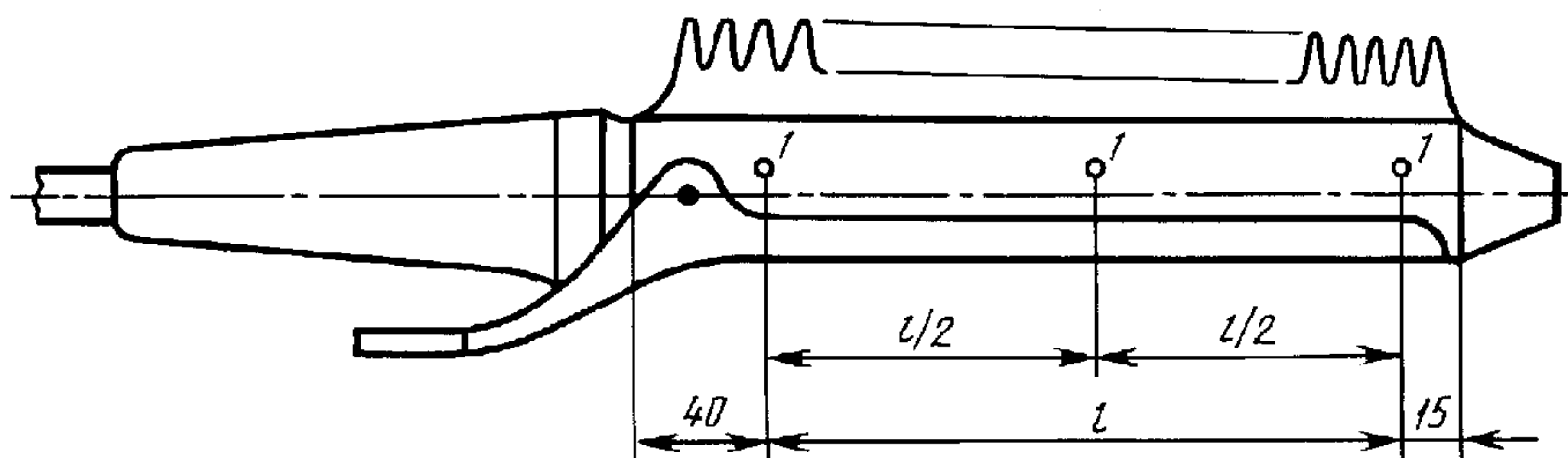
Схема прикрепления термопар на электрощипцах и электрорасческах
