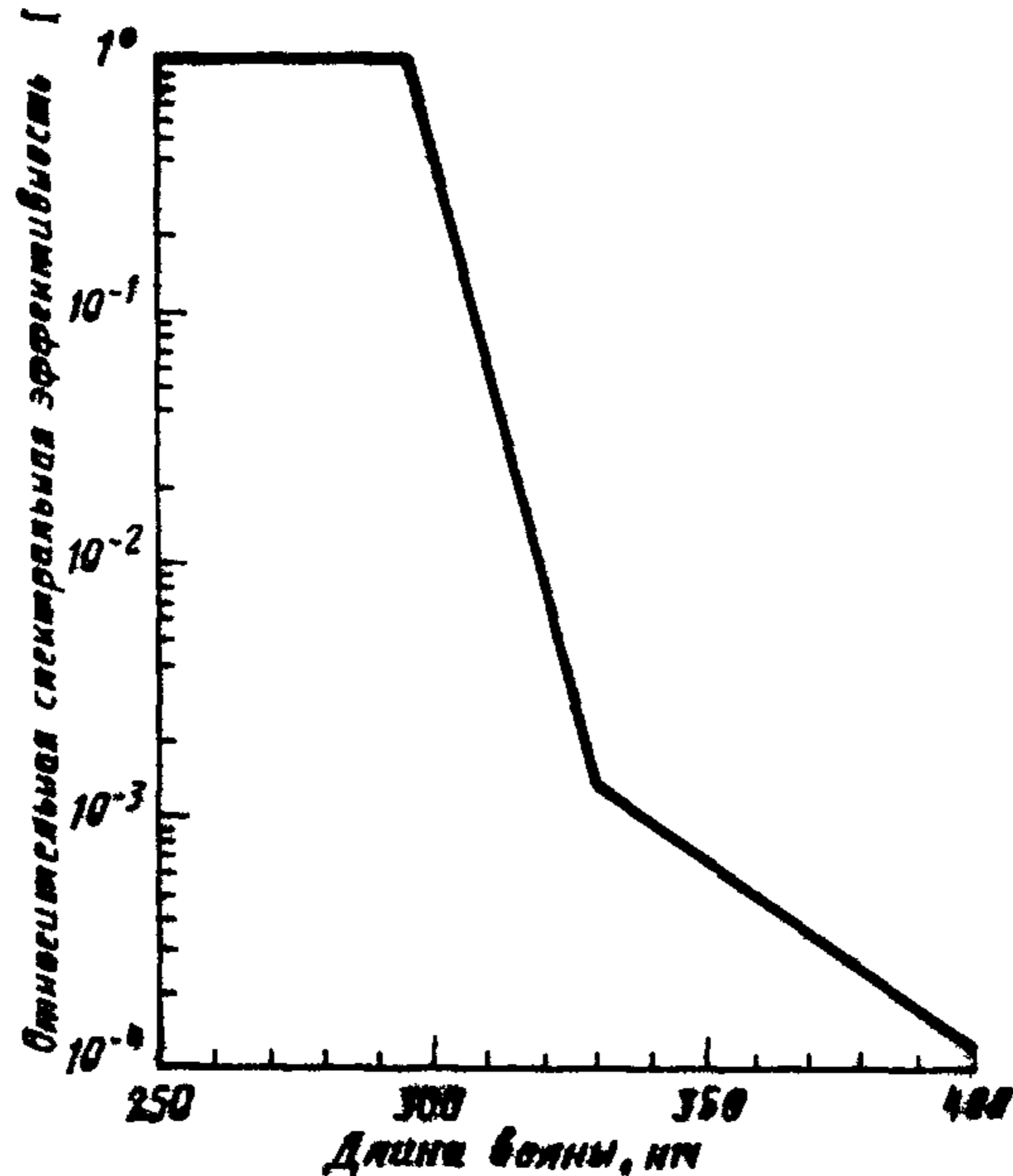
Некоторые значения кривой УФ-воздействия
