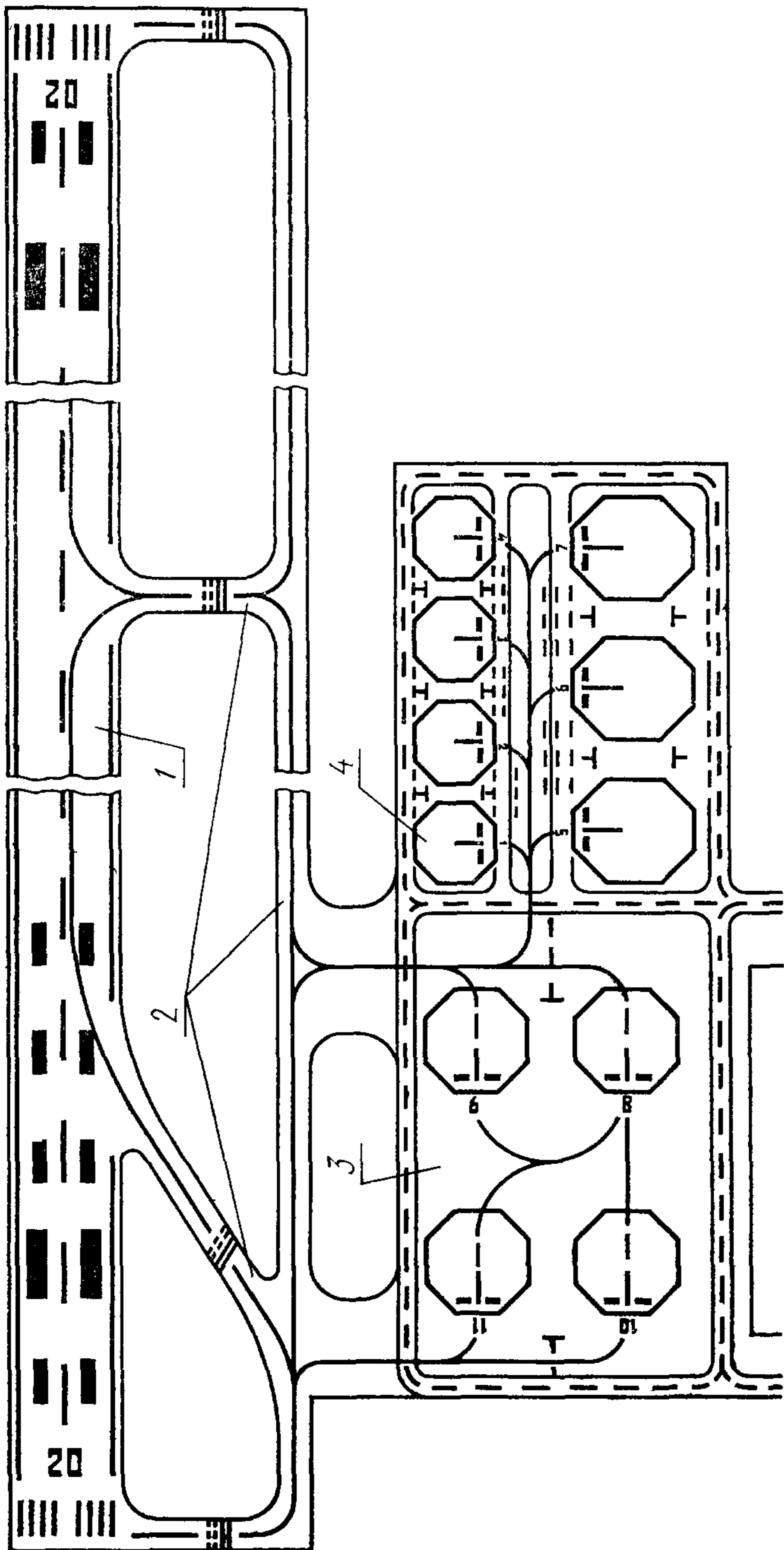
1—искусственная взлетно-посадочная полоса; 2—рулежные дорожки; 3—перрон; 4—места стоянки Черт. 1
