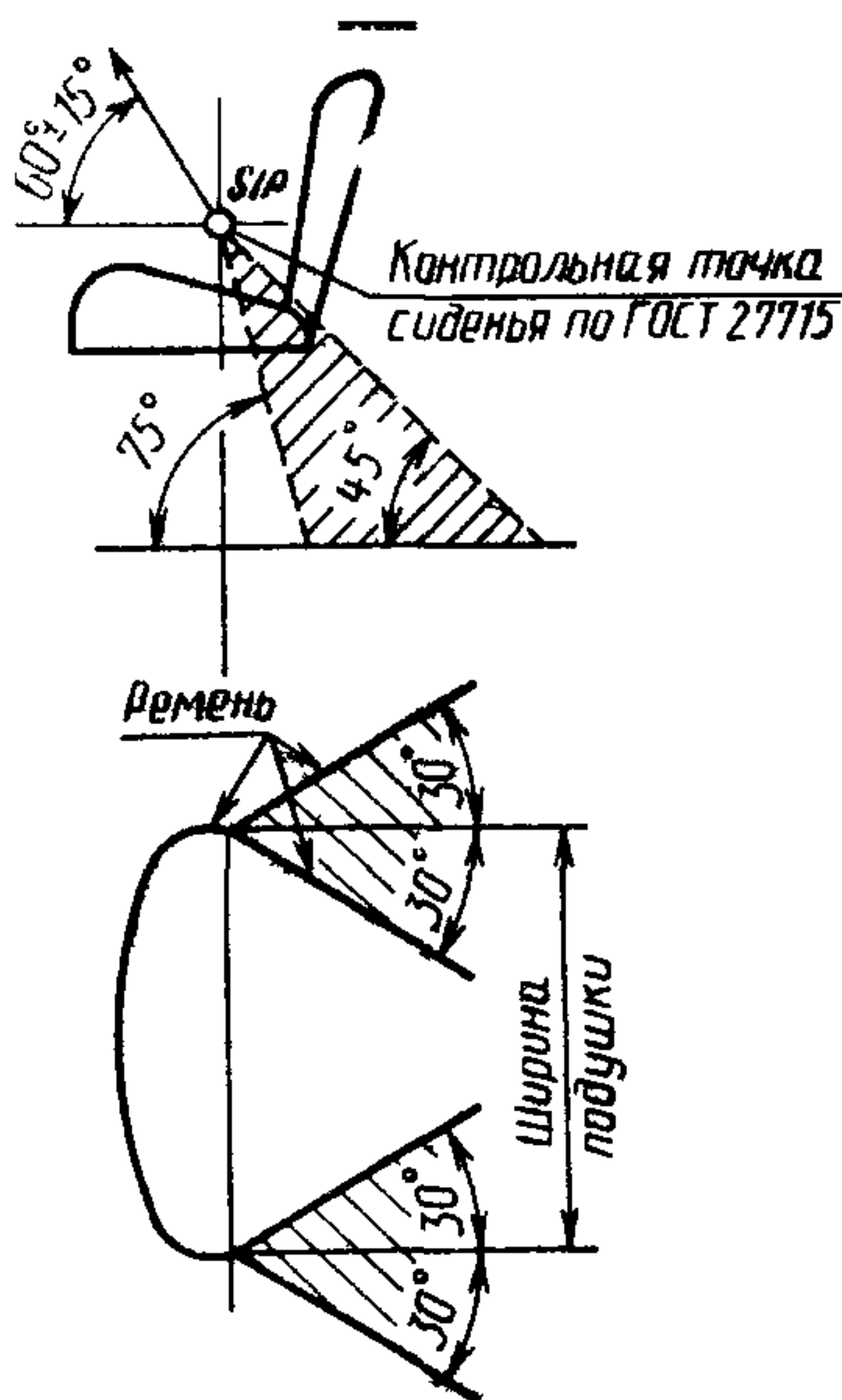
Места крепления ремней безопасности
