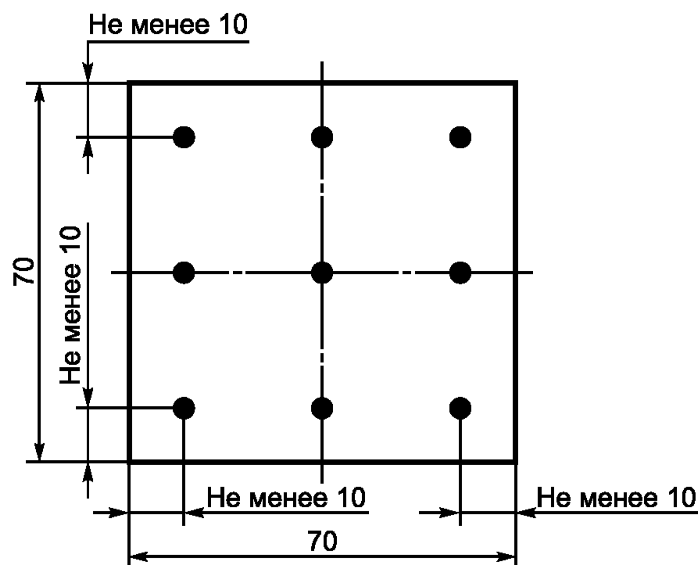
Рисунок 1 — Точки измерения толщины образца
