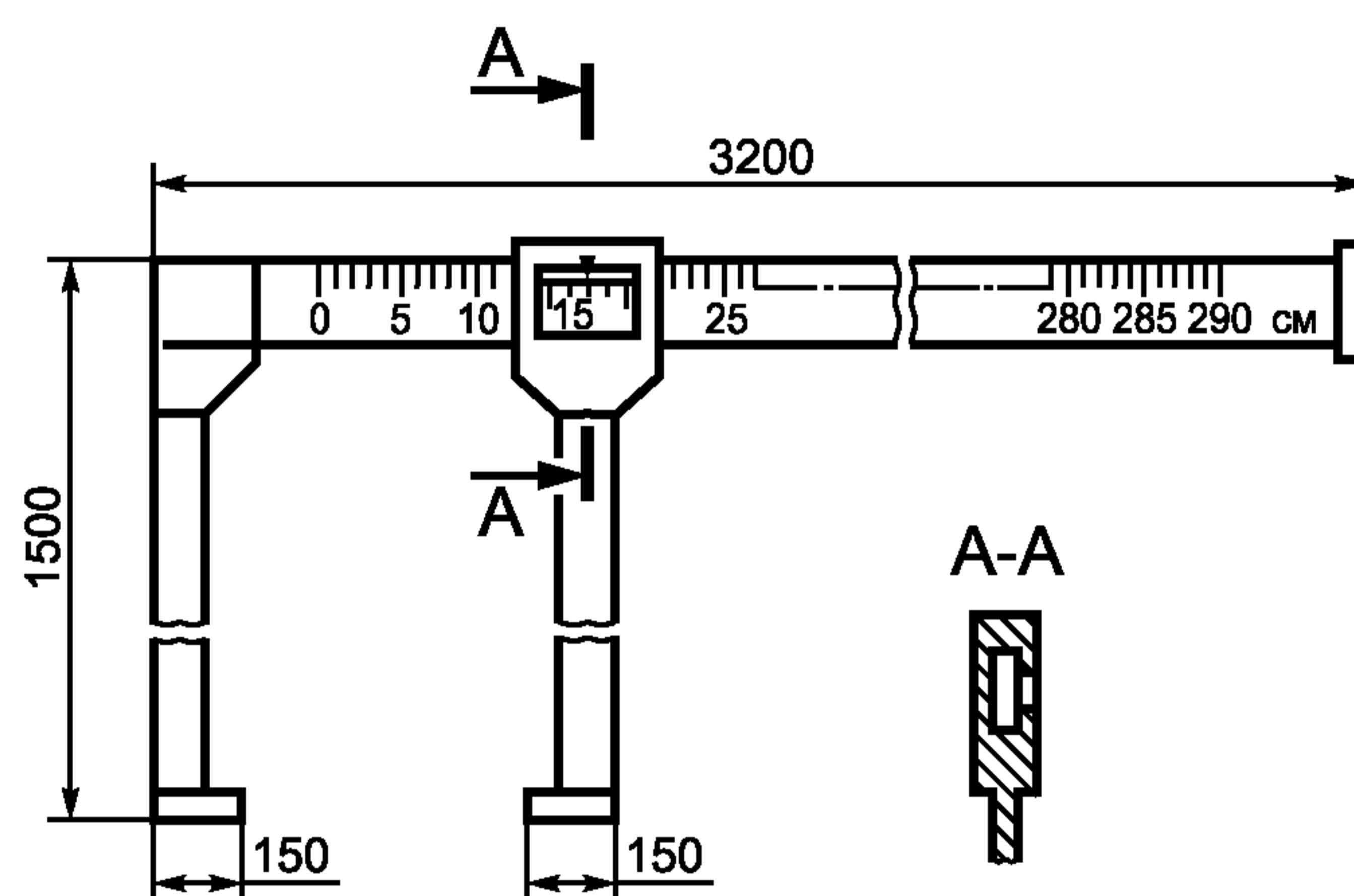
Рисунок 6 — Измерительный шаблон
