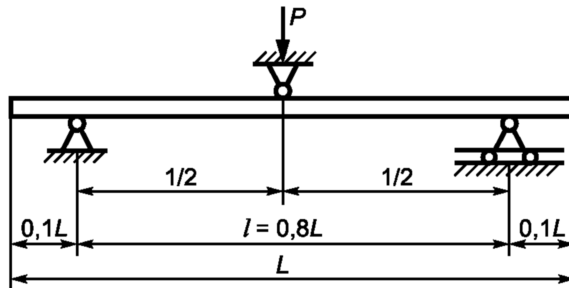
Рисунок 2 — Схема испытания при определении прочности на растяжение при изгибе
