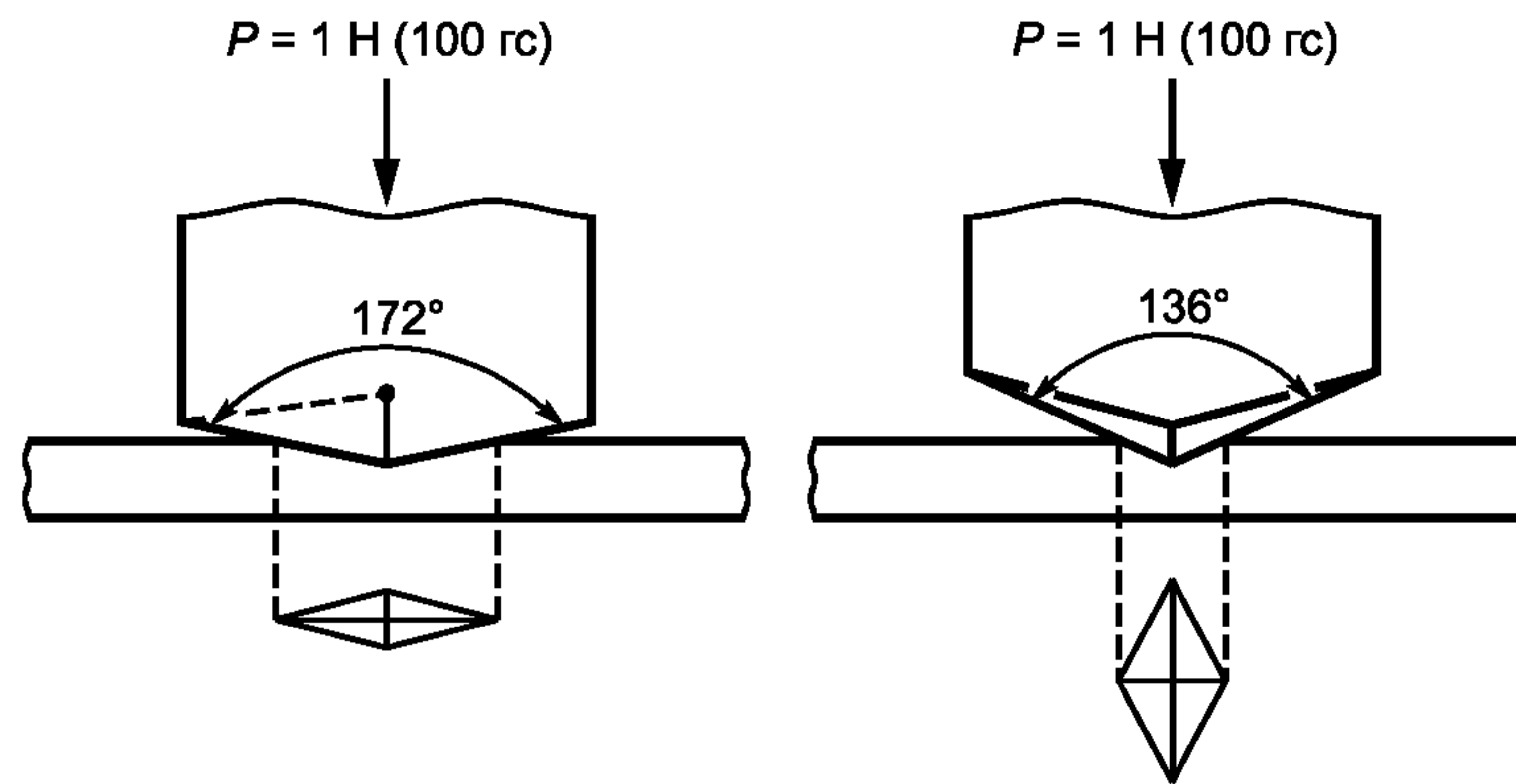
Рисунок 5 — Алмазный наконечник (пирамида) твердометра
