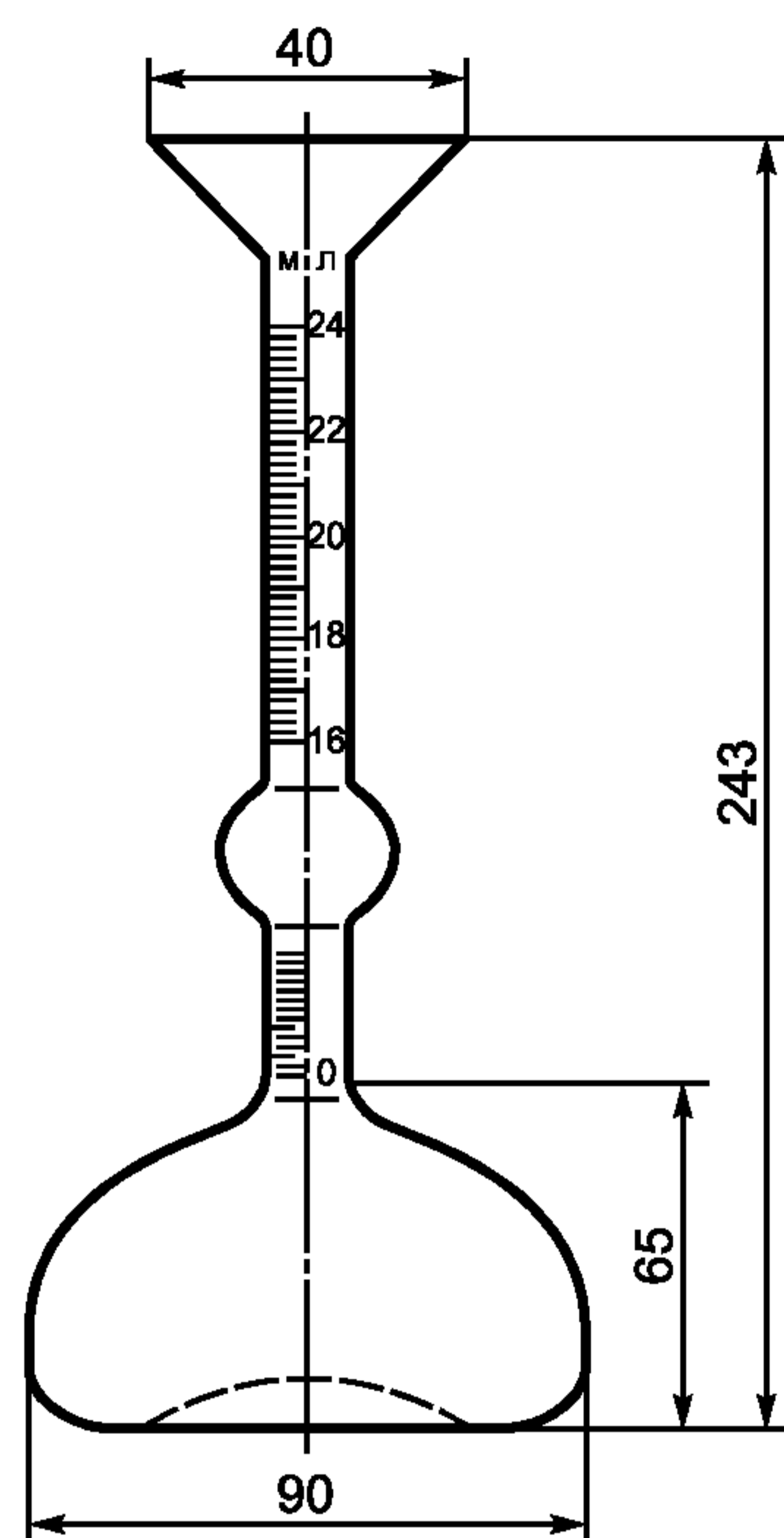
Рисунок 1 — Прибор Ле-Шателье
