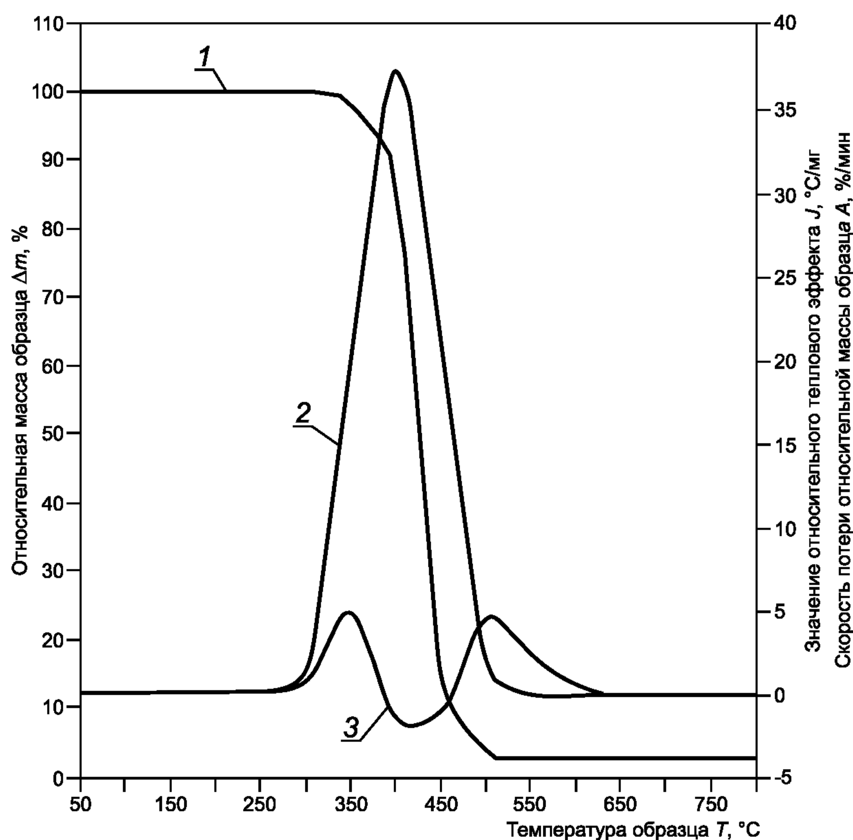
1 — ТГ-зависимость; 2 — ДТГ-зависимость; 3 — ДТА-зависимость
