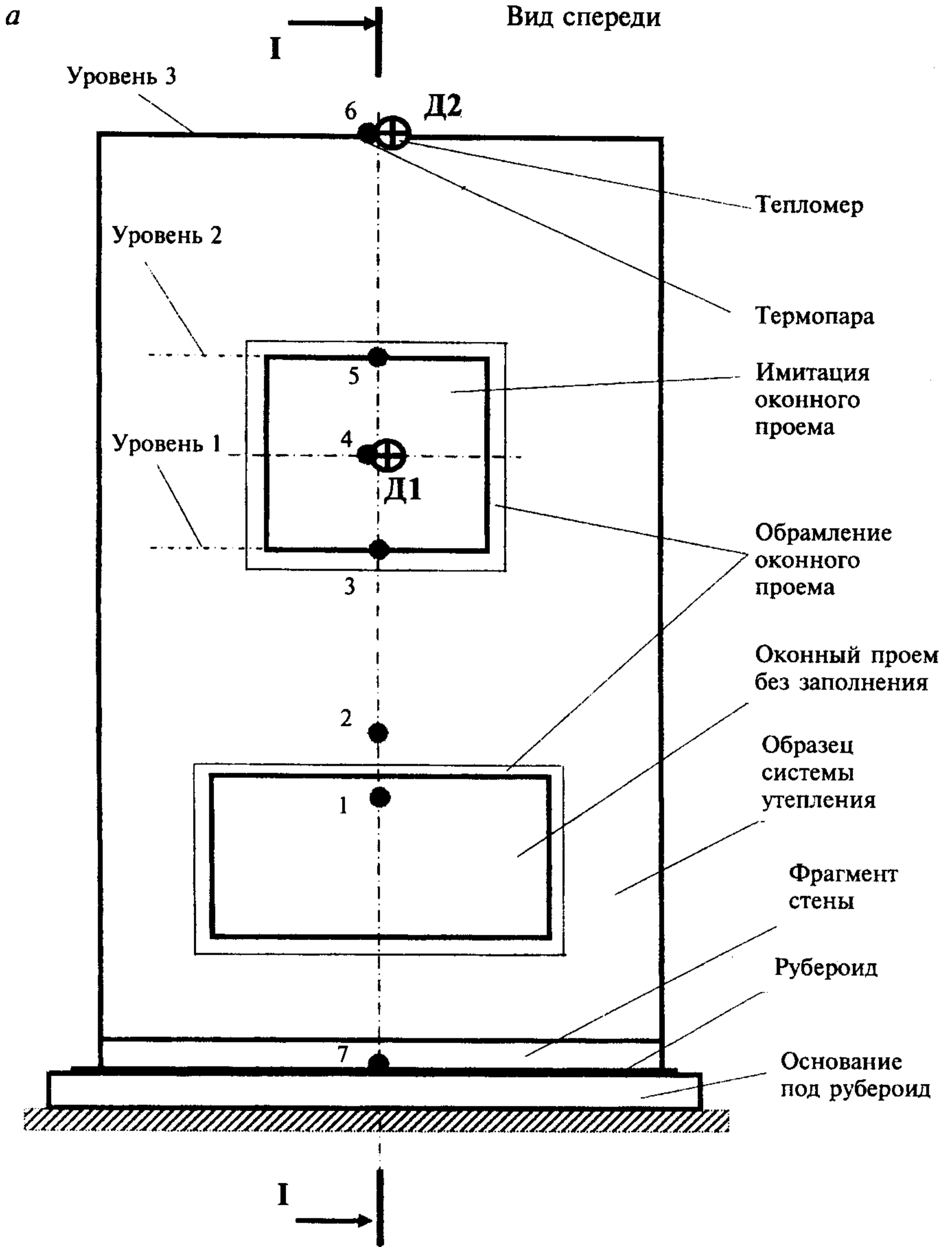
Рисунок 2 — Схема установки с образцом системы утепления
