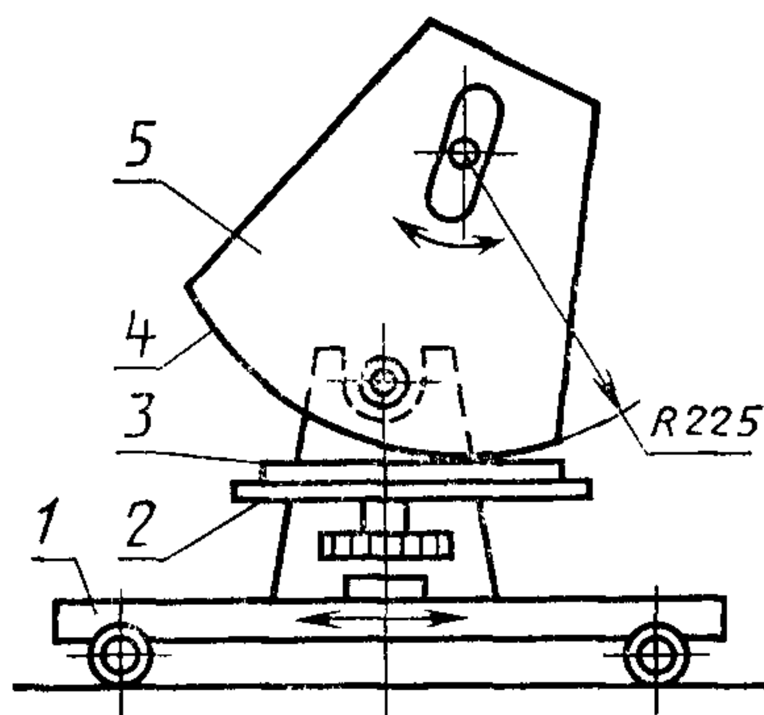
1—площадка; 2—стол, 3—образец; 4—шлифовальная шкурка, 5—рабочий элемент
