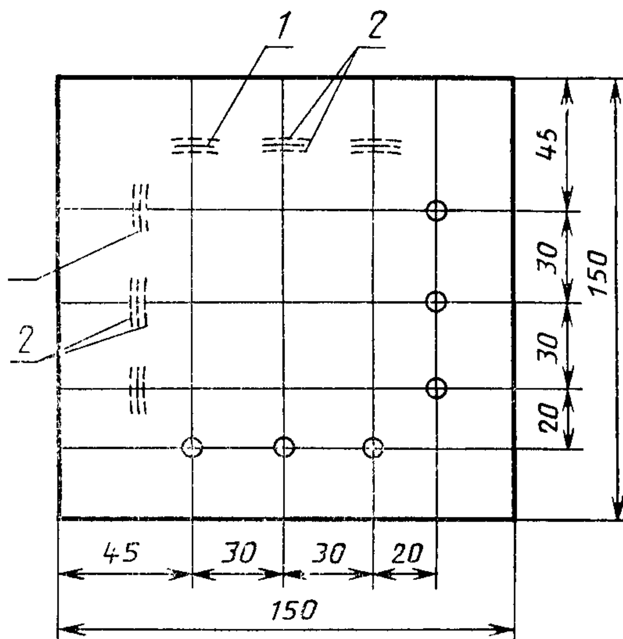
1—риски до испытания; 2—риски после испытания
