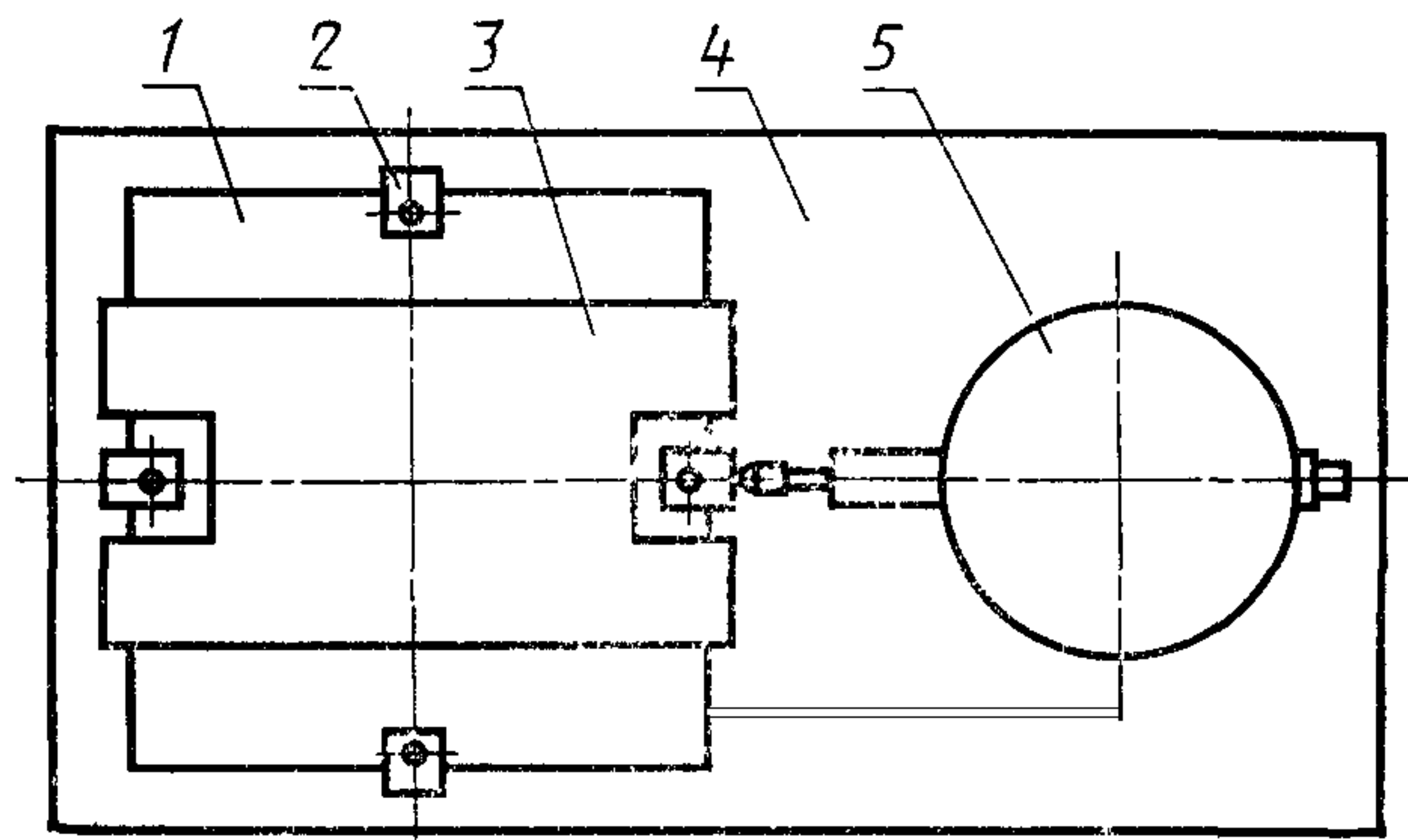
1—образец; 2—зажим; 3—прижим; 4—основание; 5—индикатор часового типа
