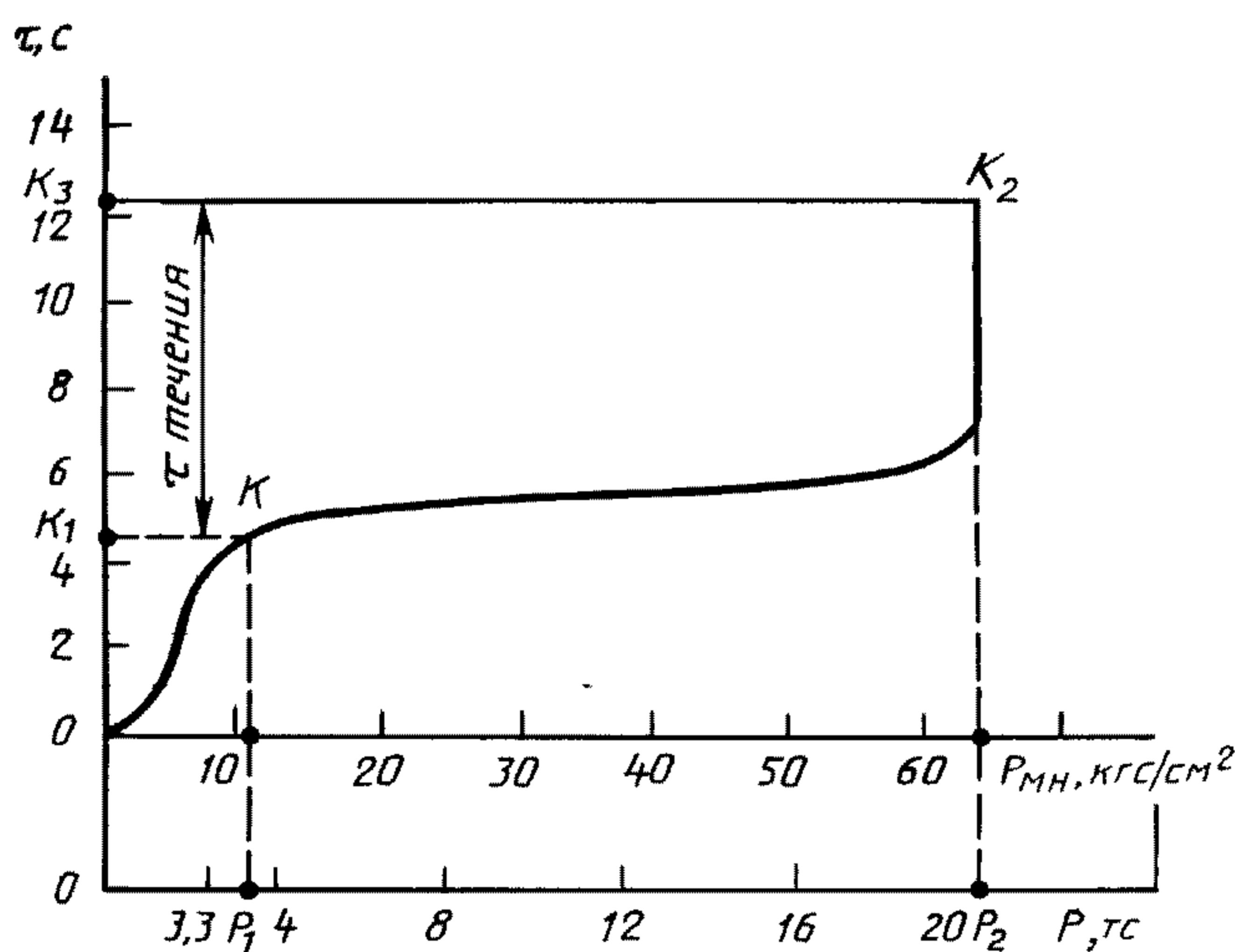
График определения времени течения по кривой диаграммы “время — давление”
