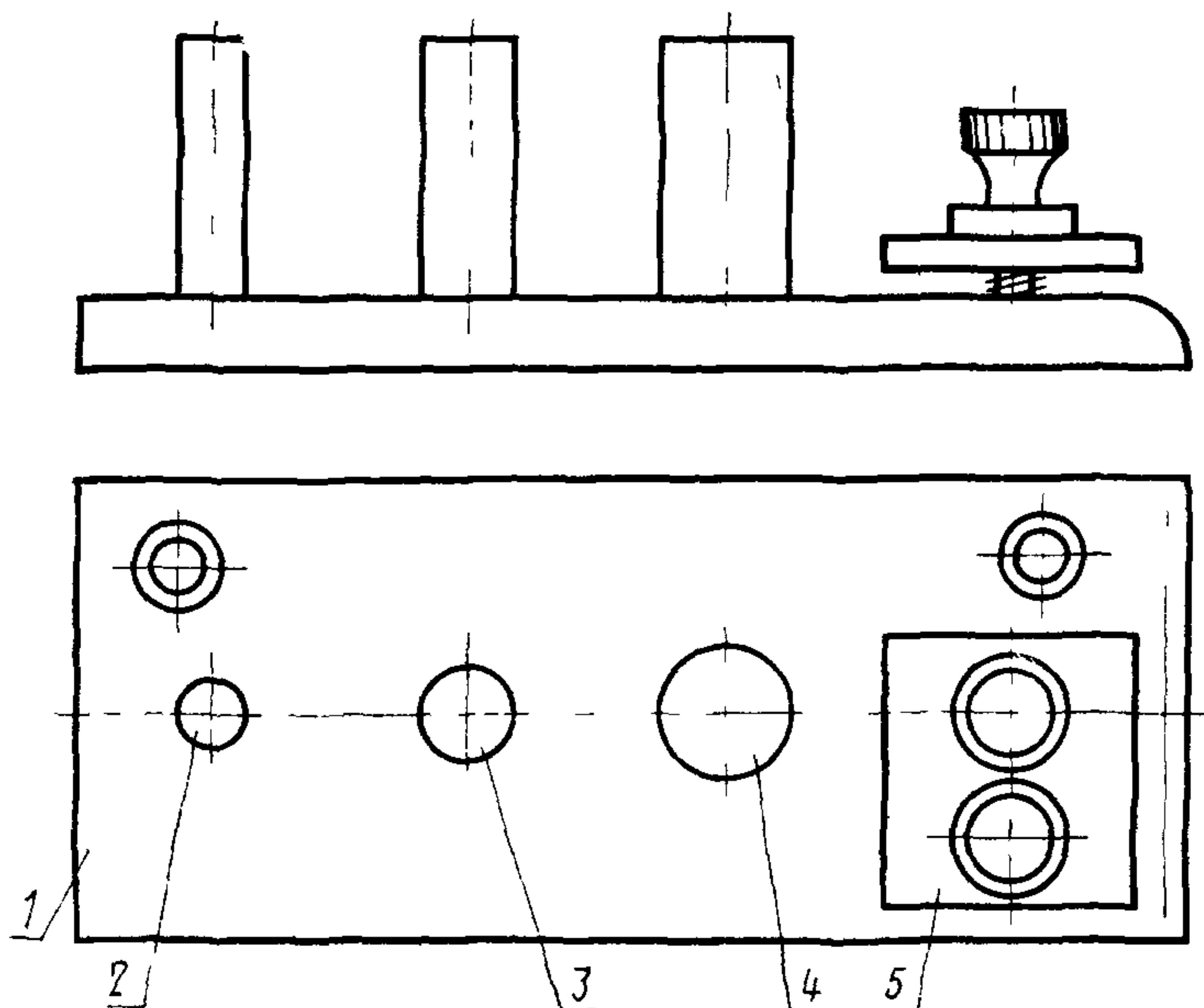
1 — плита; 2, 3, 4 — стержни; 5 — пластина для закрепления образцов
