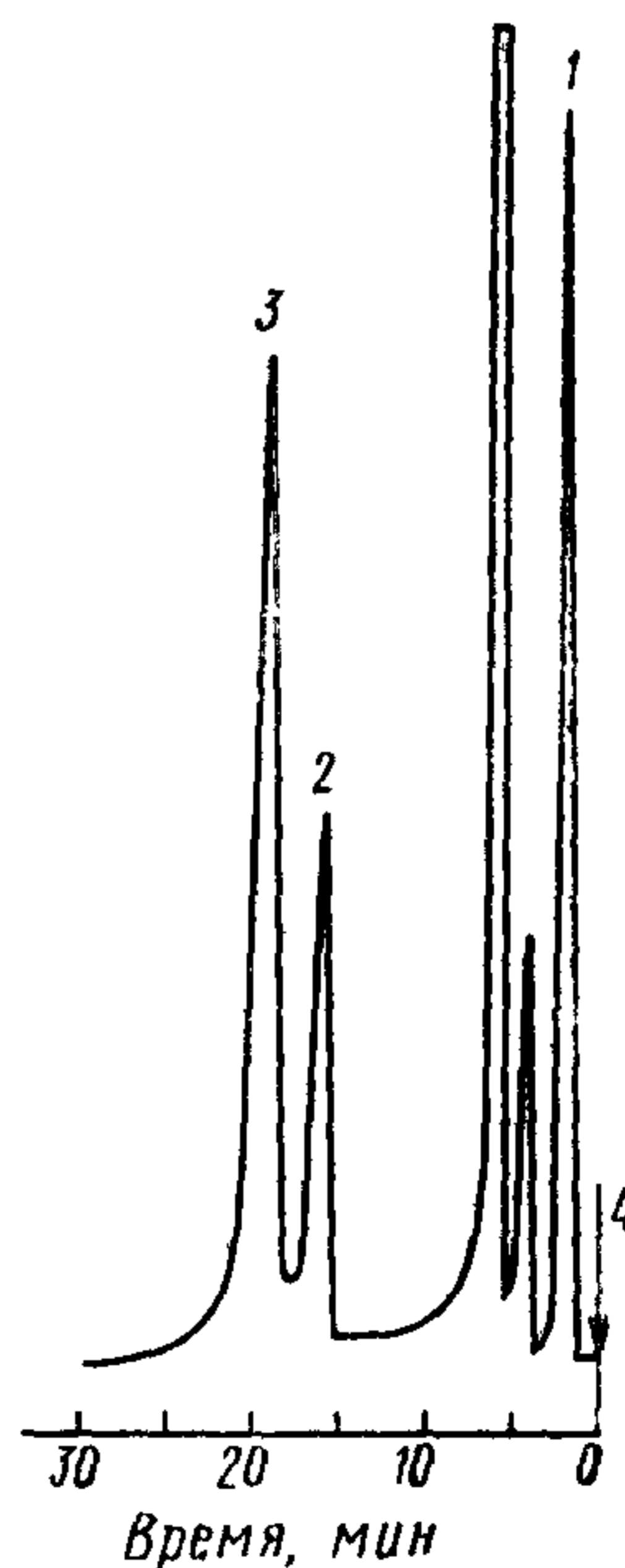
Хроматограмма фенолоформальдегидных смол, содержащих ацетон
