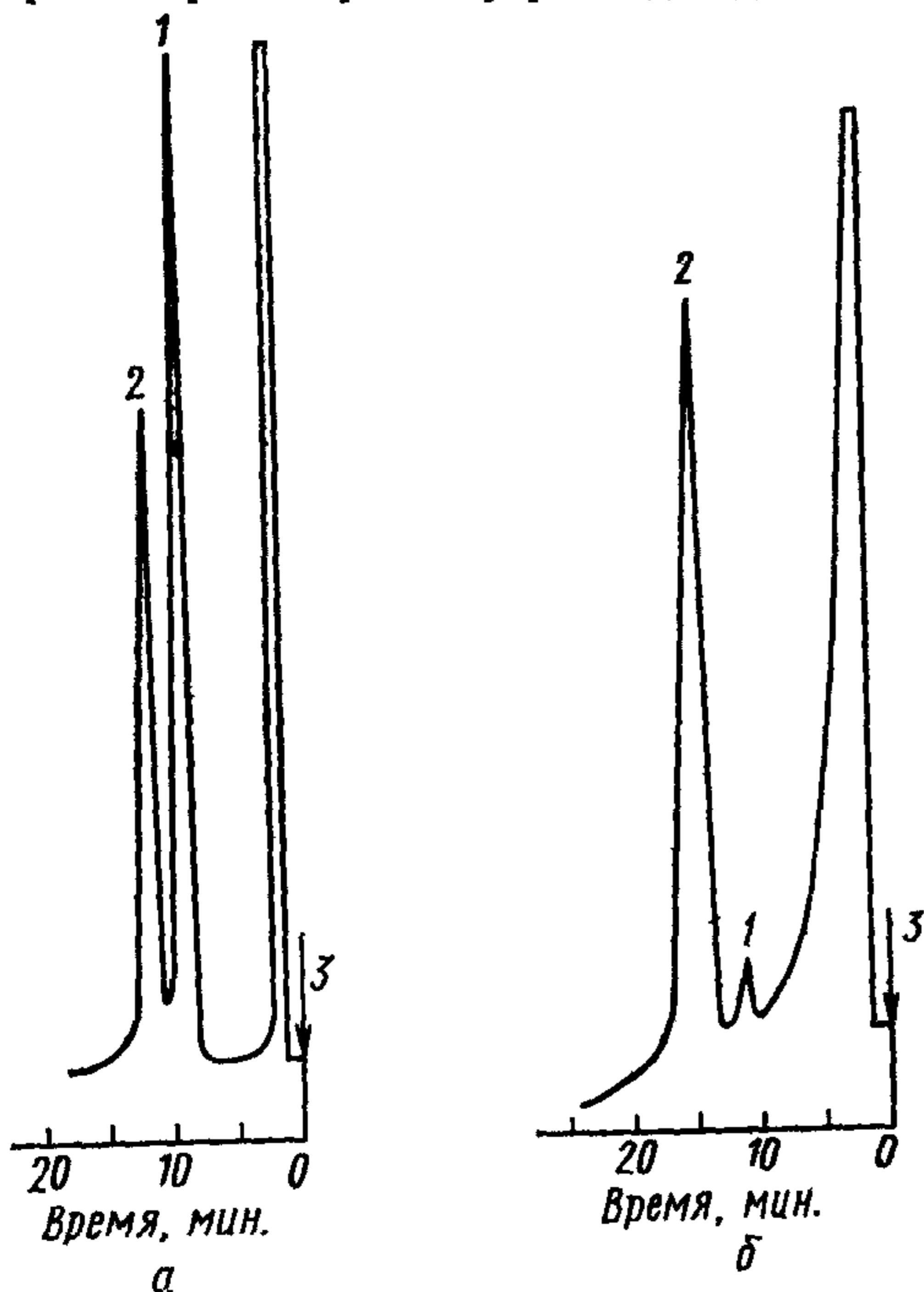
Хроматограмма фенолоформальдегидных смол
