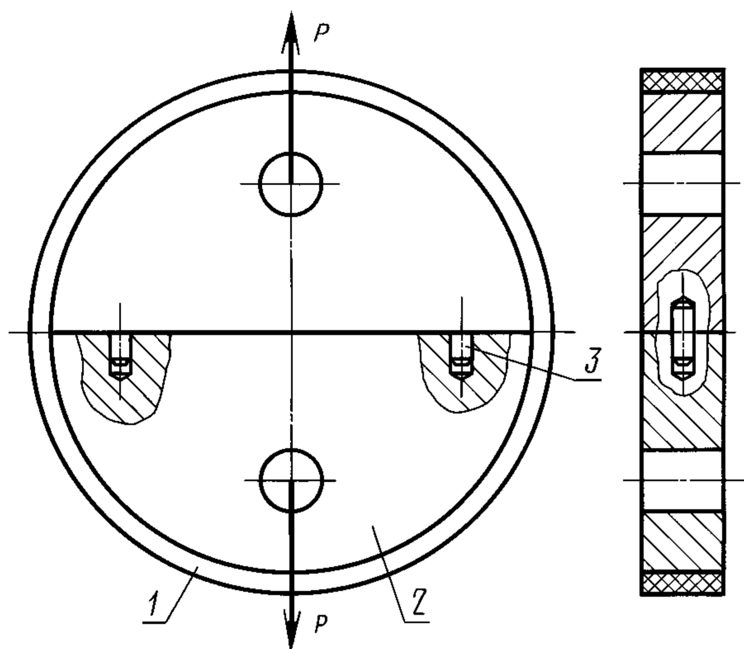
1 — образец; 2 — полудиск; 3 — штифт
