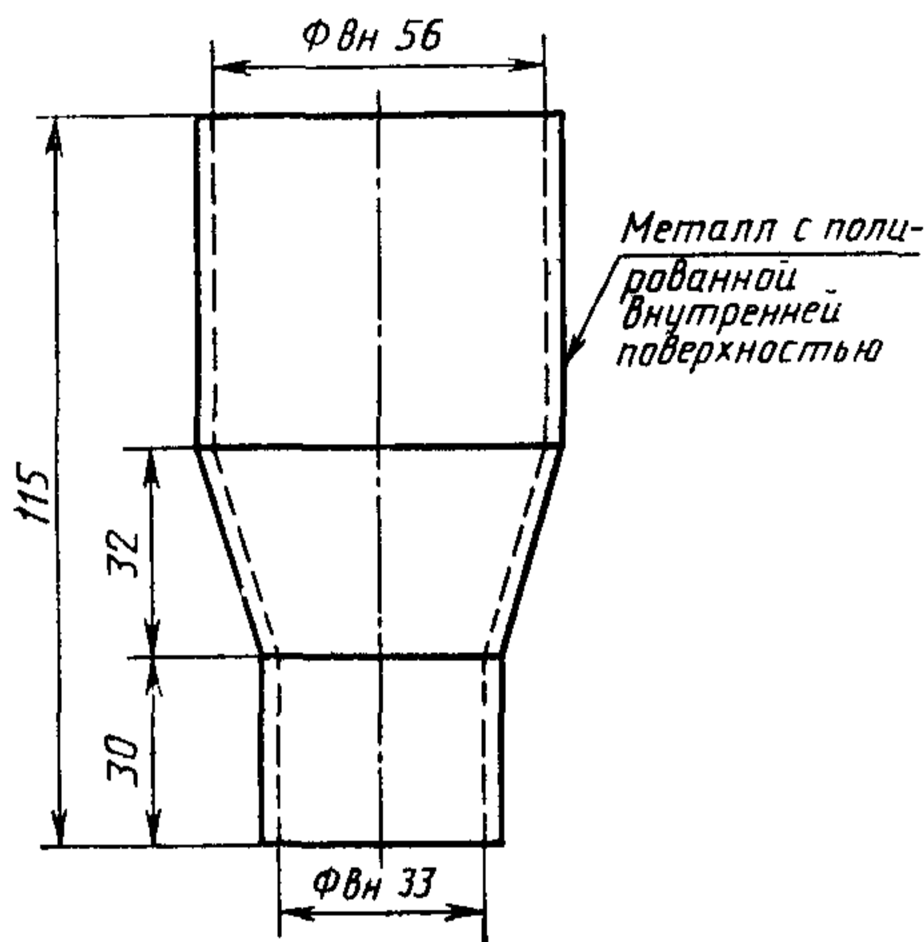
Воронка для определения насыпной плотности
