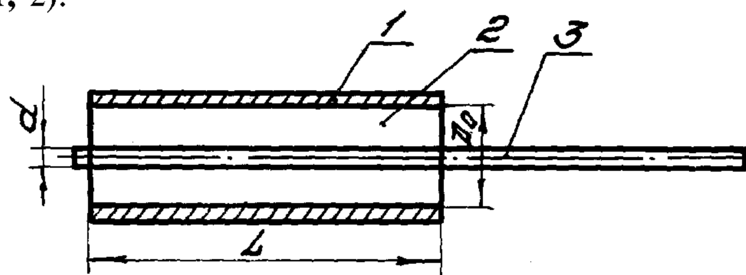
1 — оболочка; 2 — уплотненный порошок; 3 — стержень
