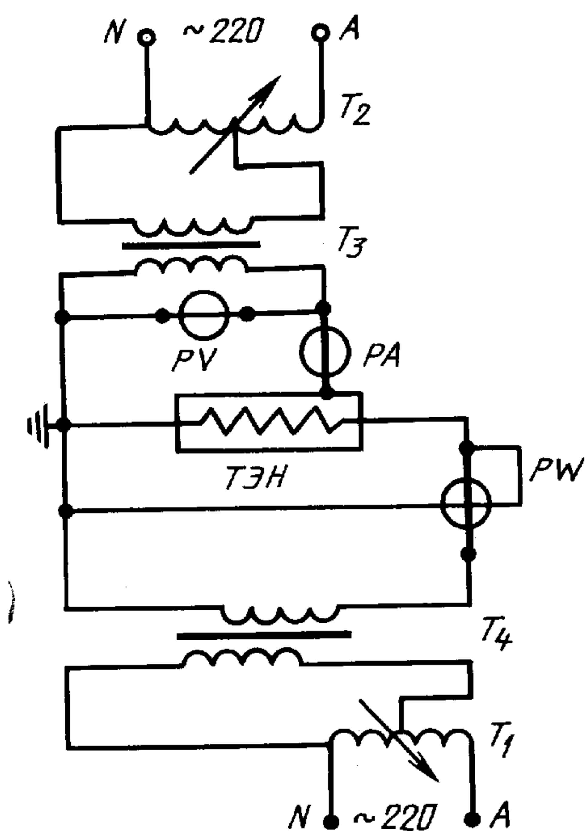
Электрическая схема
