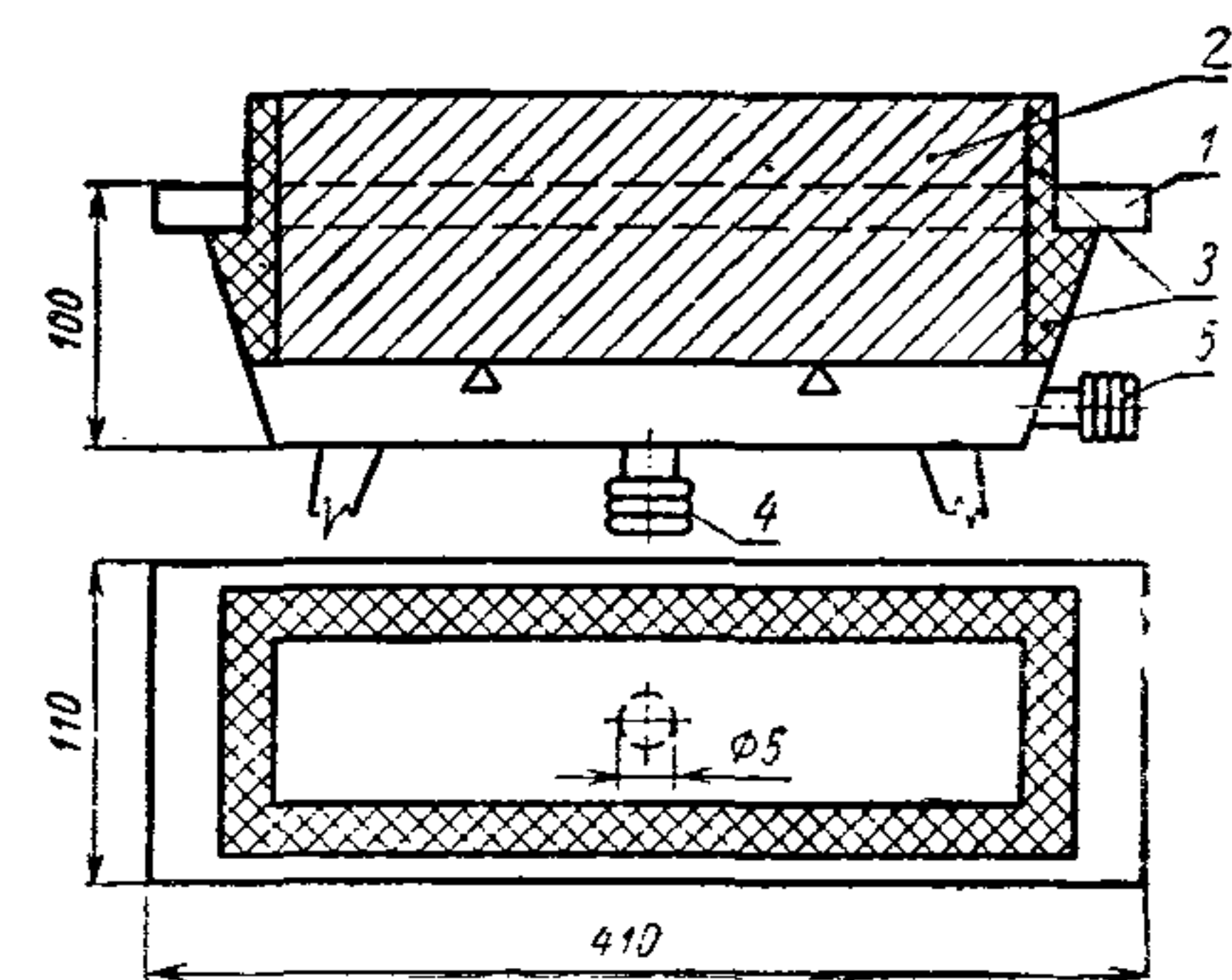
1 — держатель; 2 — кирпич; 3 — замазка; 4 — патрубок для подвода воздуха; 5 — па- трубок для присоединения манометра
