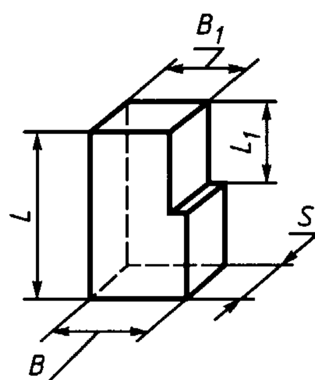
Рисунок 6 — Кирпич фасонный опорный
