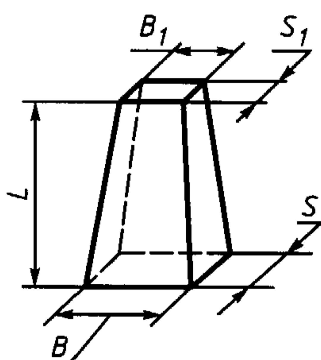
Рисунок 5 — Клин пирамидальный двухсторонний
