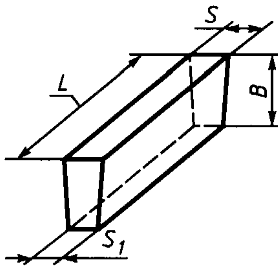
Рисунок 3 — Клин ребровый двухсторонний
