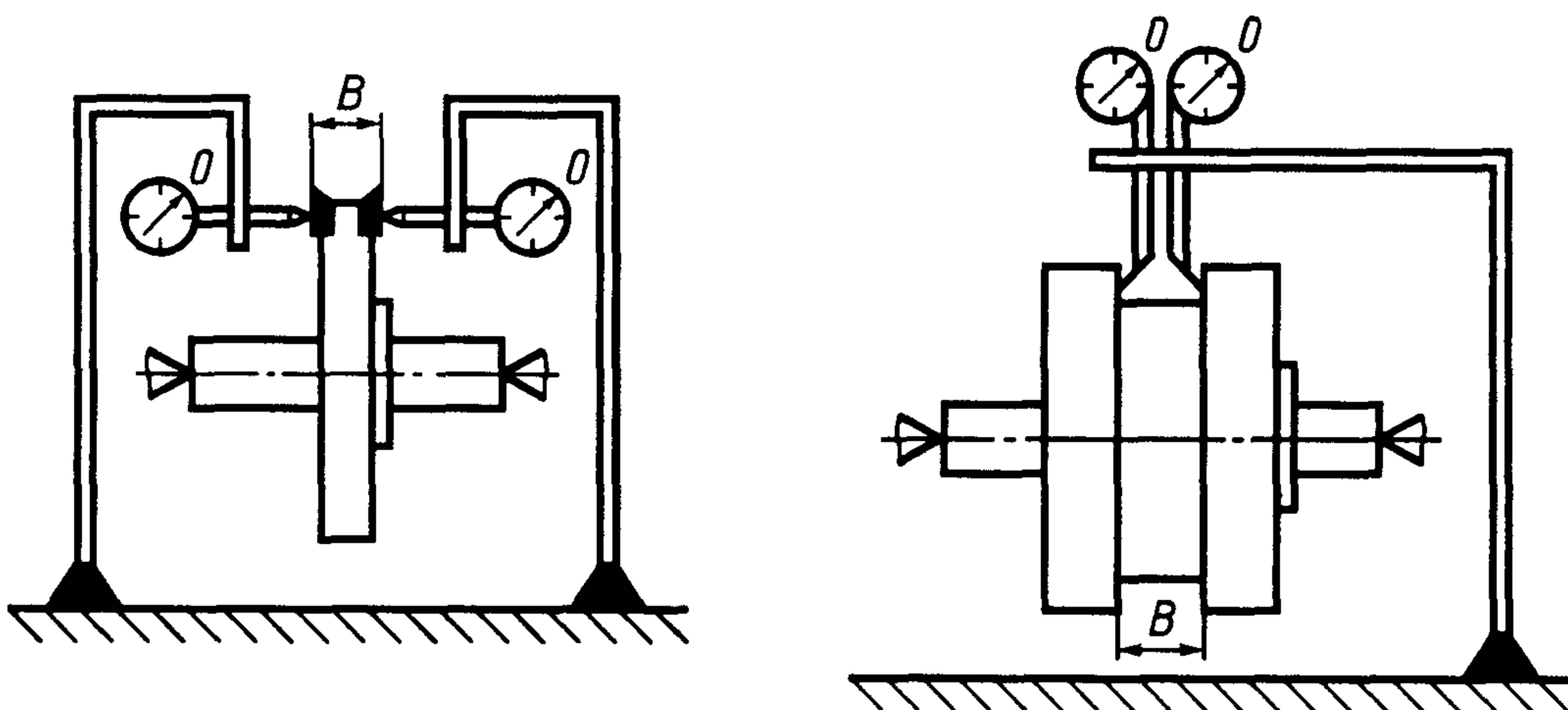
Схема измерения ширины фрез
