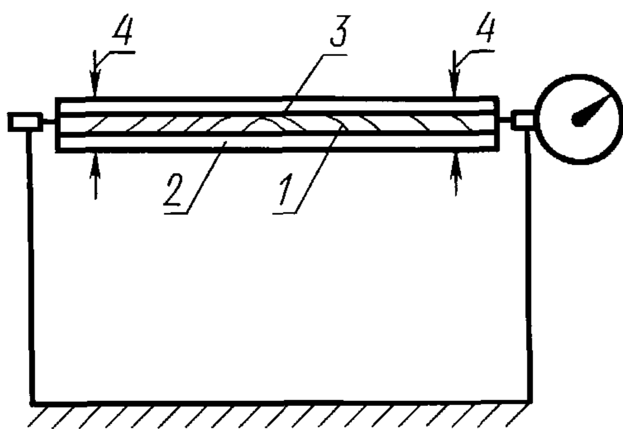
1 — слой секции D ; 2 — основание; 3 — подкладка; 4 — усилия винтовых зажимов
