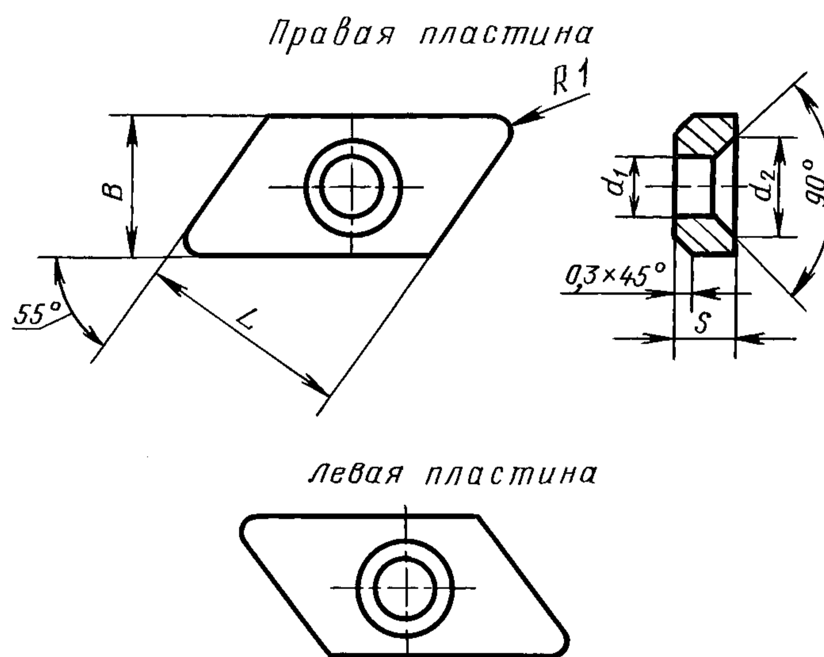
Размеры, мм
