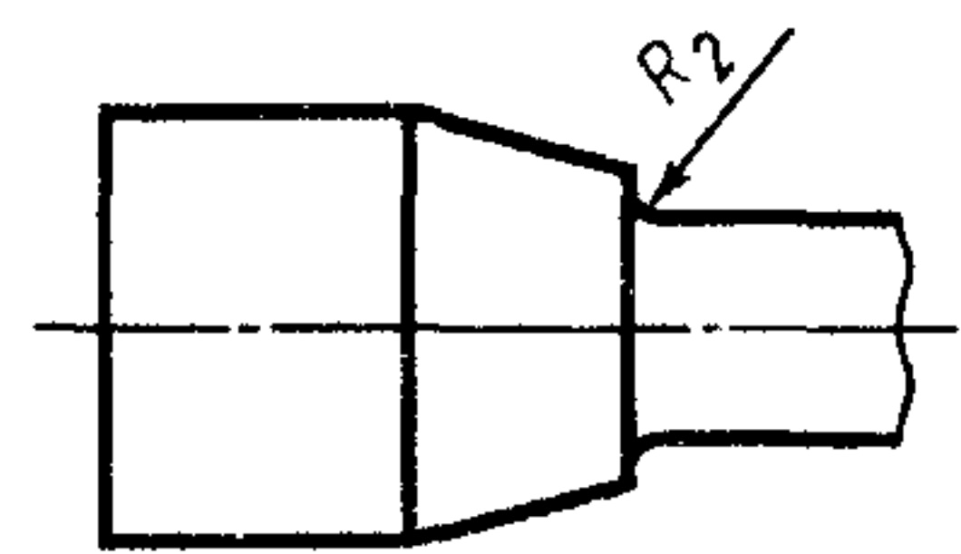
Рисунок 2 — Головка образца с переходным участком
