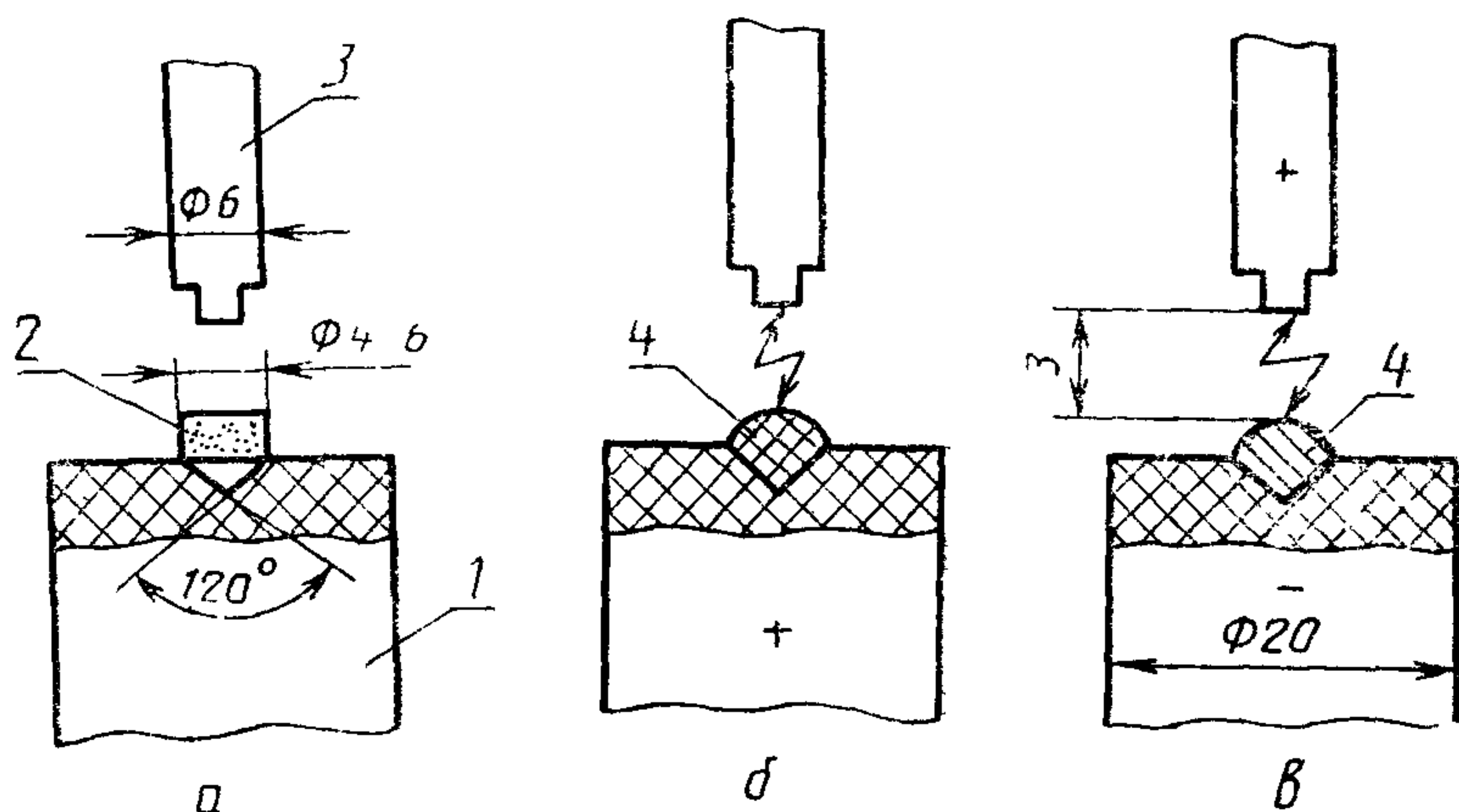
1 — графитовый электрод-подставка; 2 — таблетка пробы или стандартного образца; 3 — графитовый электрод; 4 — капля расплава а — до экспонирования, б — при анодной полярности таблетки, в — при катодной полярности таблетки.
