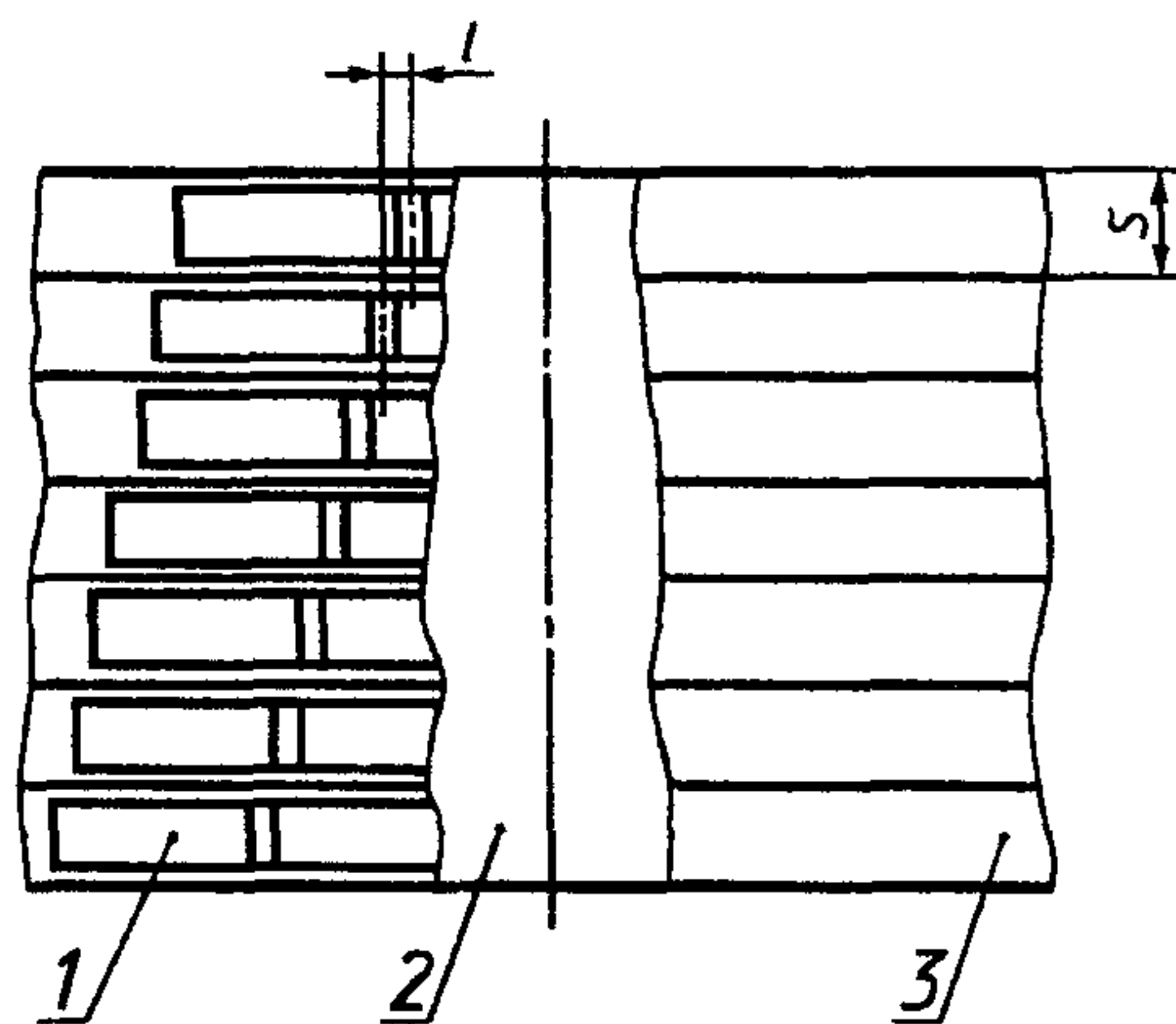
1 — образец; 2 — наплавленный валик; 3 — брусок
