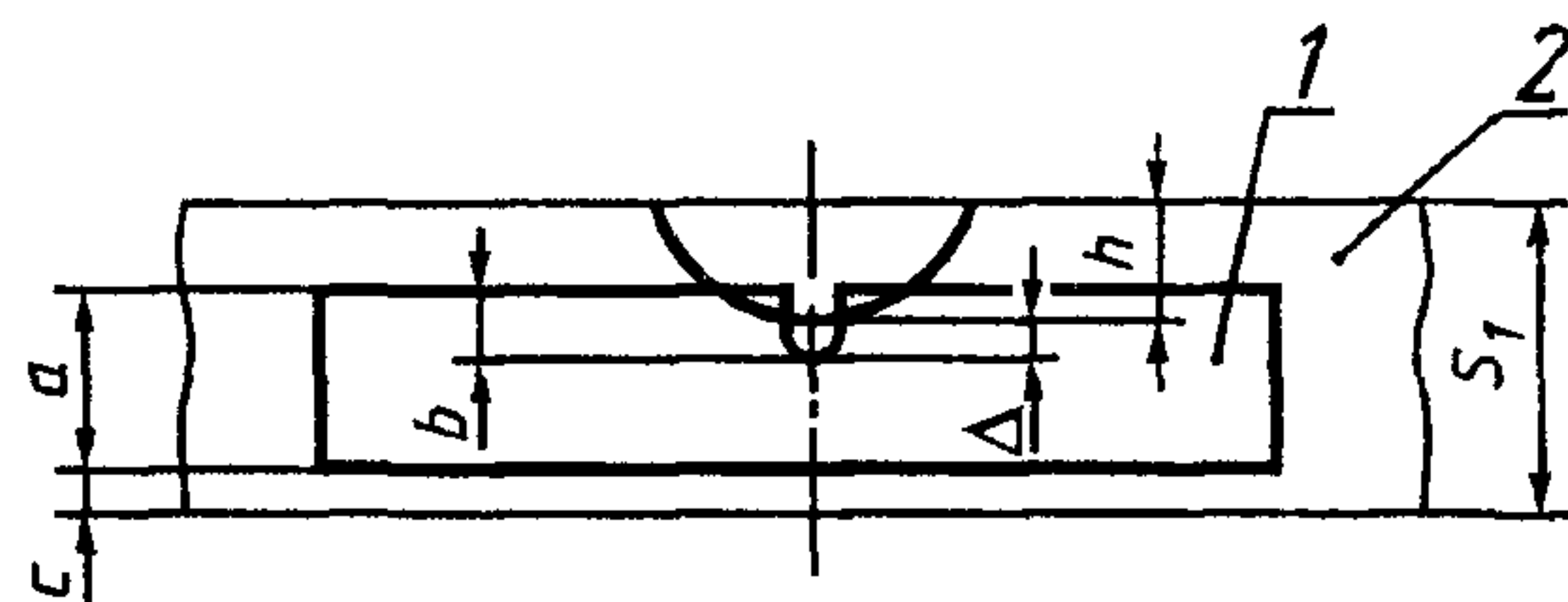
1 — образец; 2 — составная пластина
