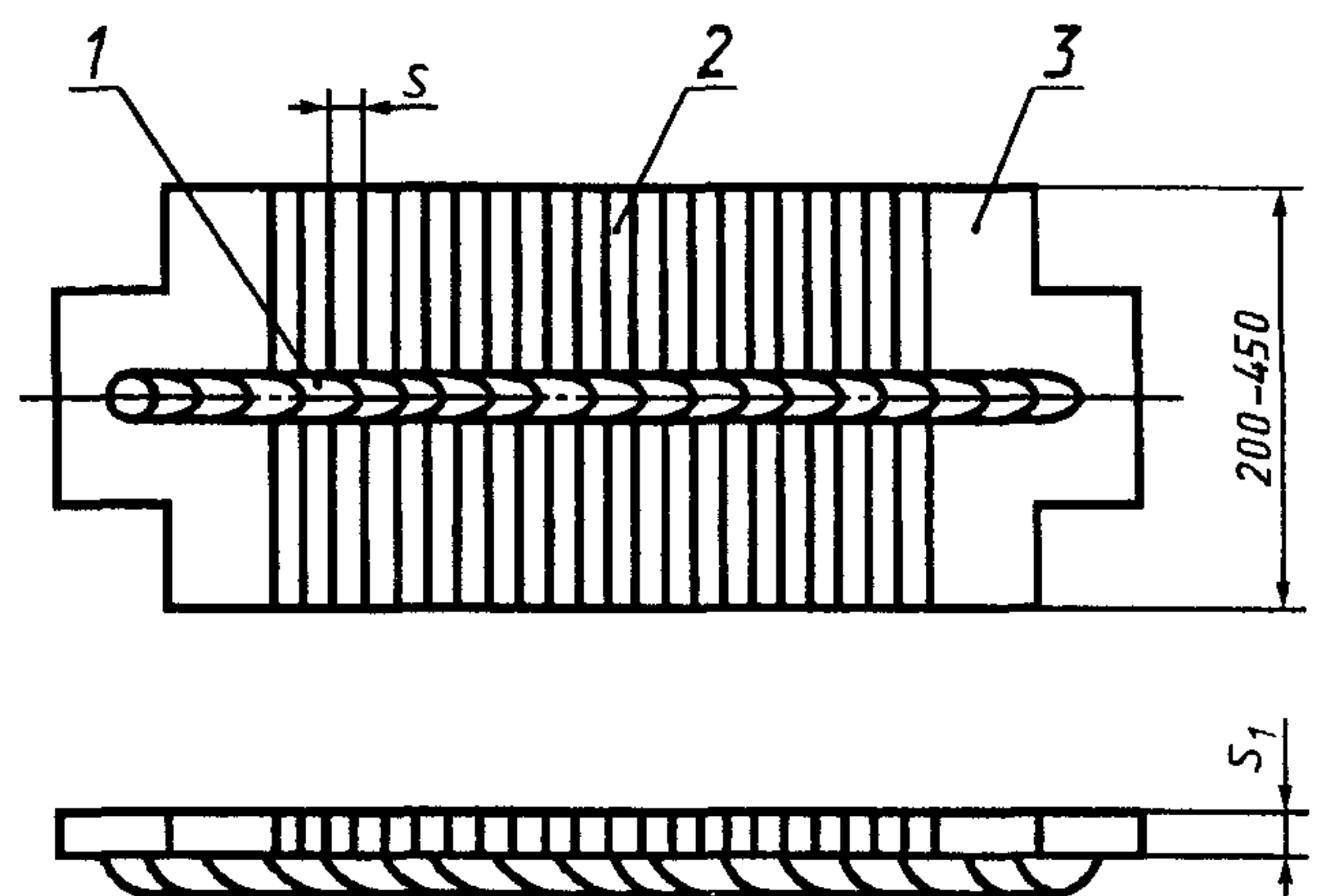
1 — валик; 2 — брусок; 3 — планка приставная
