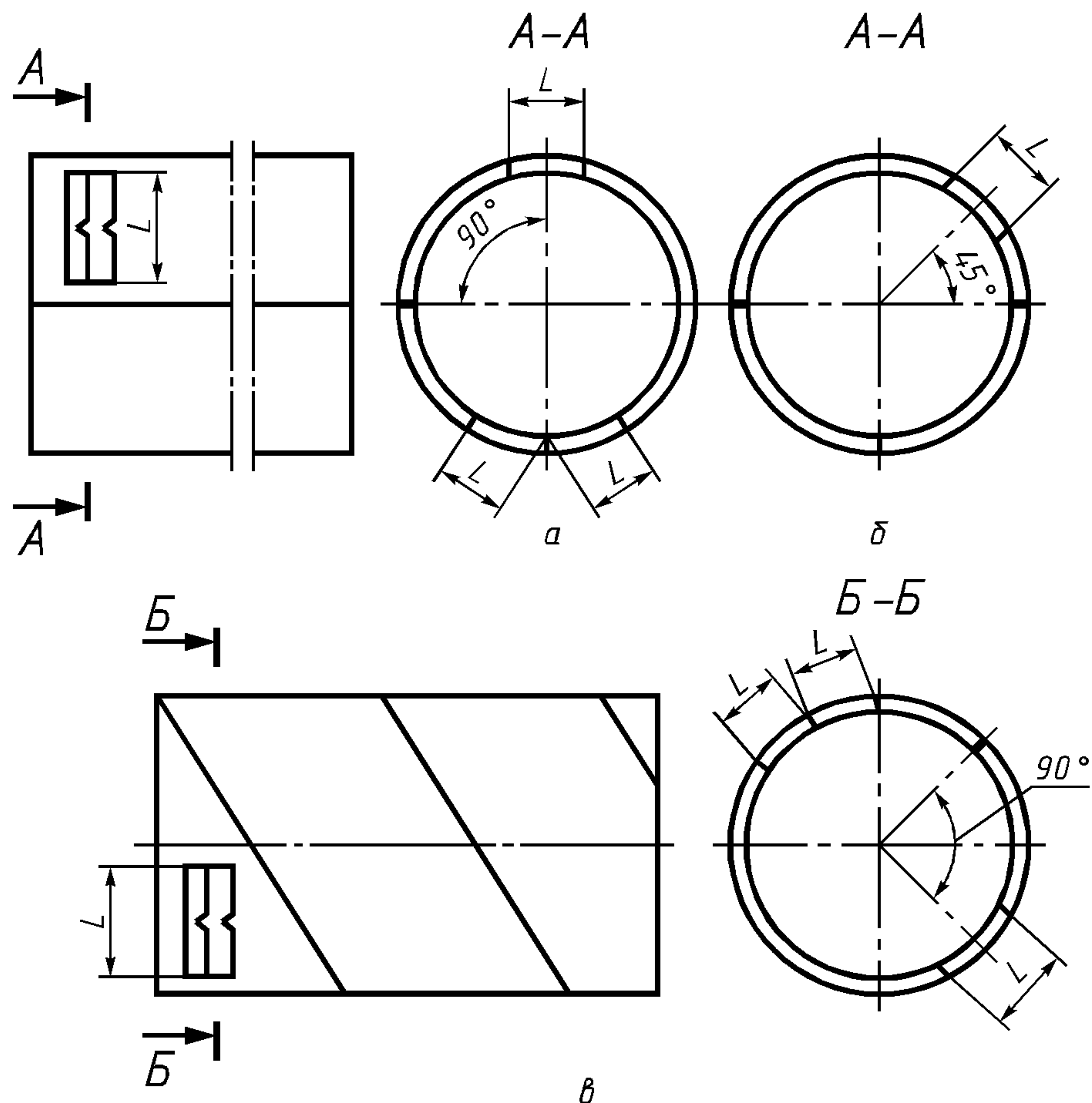
a — прямошовная труба с одним швом; b — прямошовная труба с двумя швами; v — спирально-шовная труба; L — длина образца
