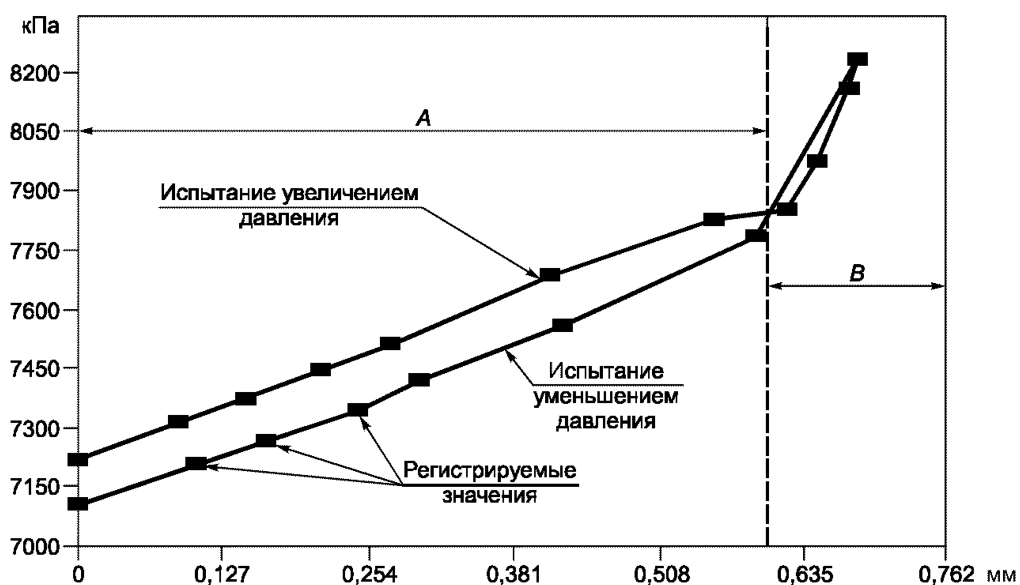
Рисунок 11 — Диаграммы перемещения штока по результатам испытаний
