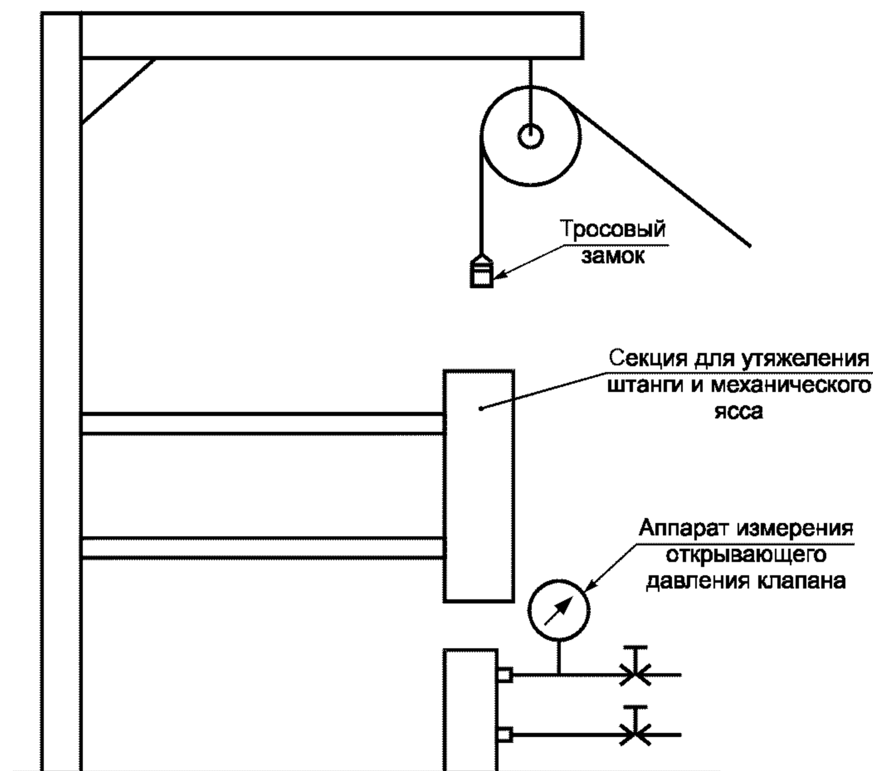
Рисунок 13 — Стенд для испытания установки клапана
