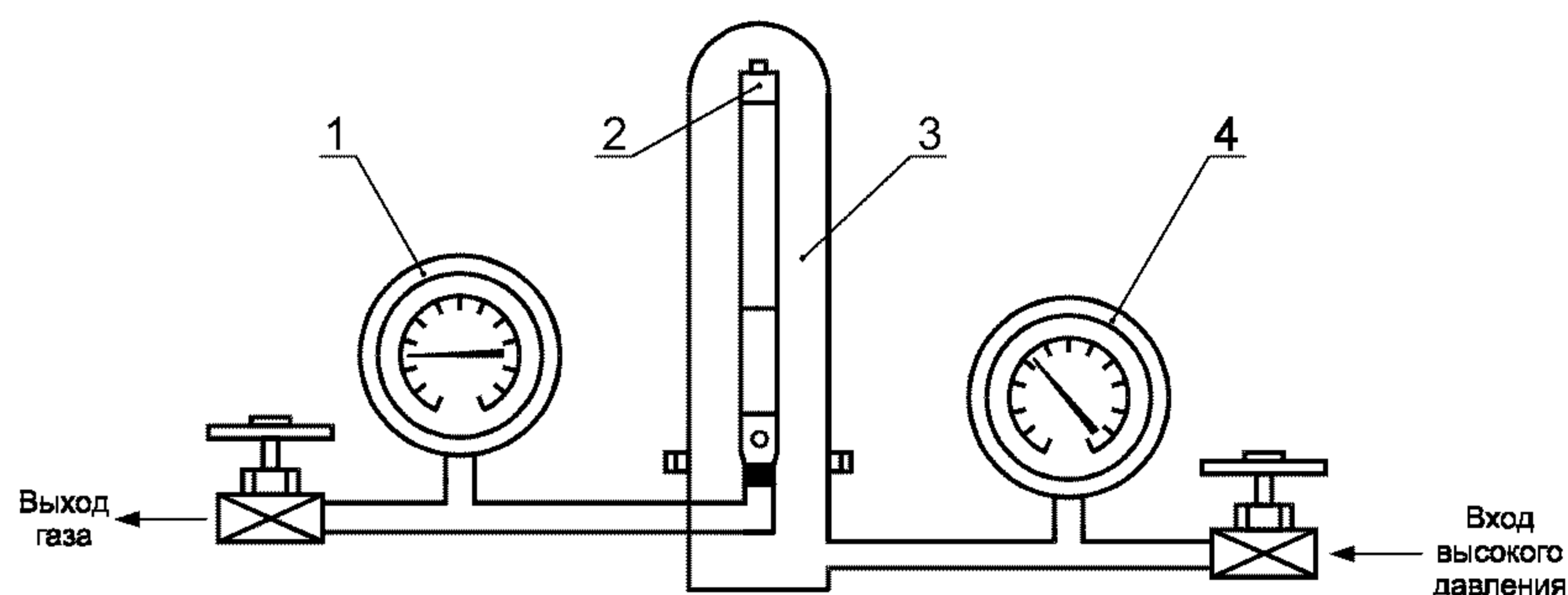
1, 4 — манометры; 2 — газлифтный клапан; 3 — камера давления
