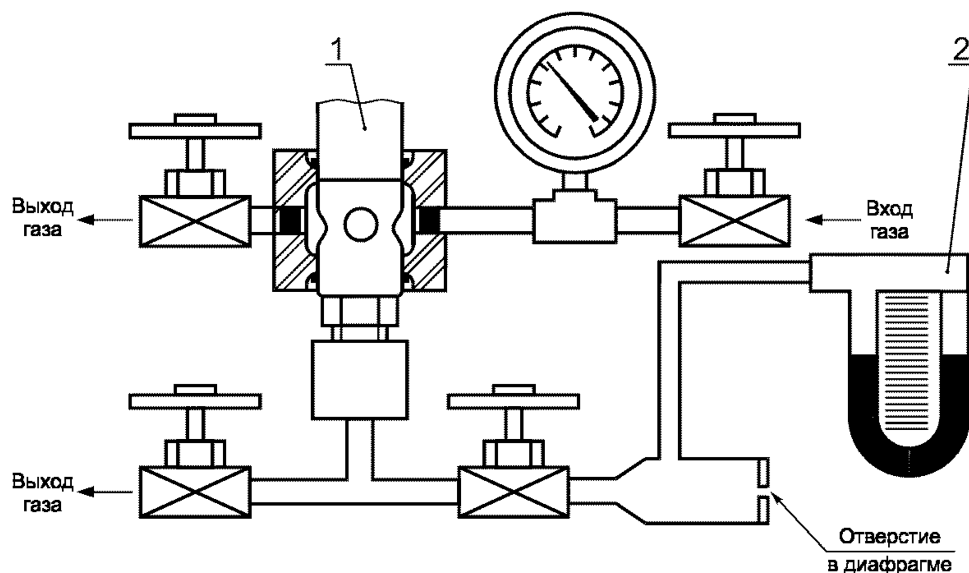
1 — газлифтный клапан; 2 — манометр
