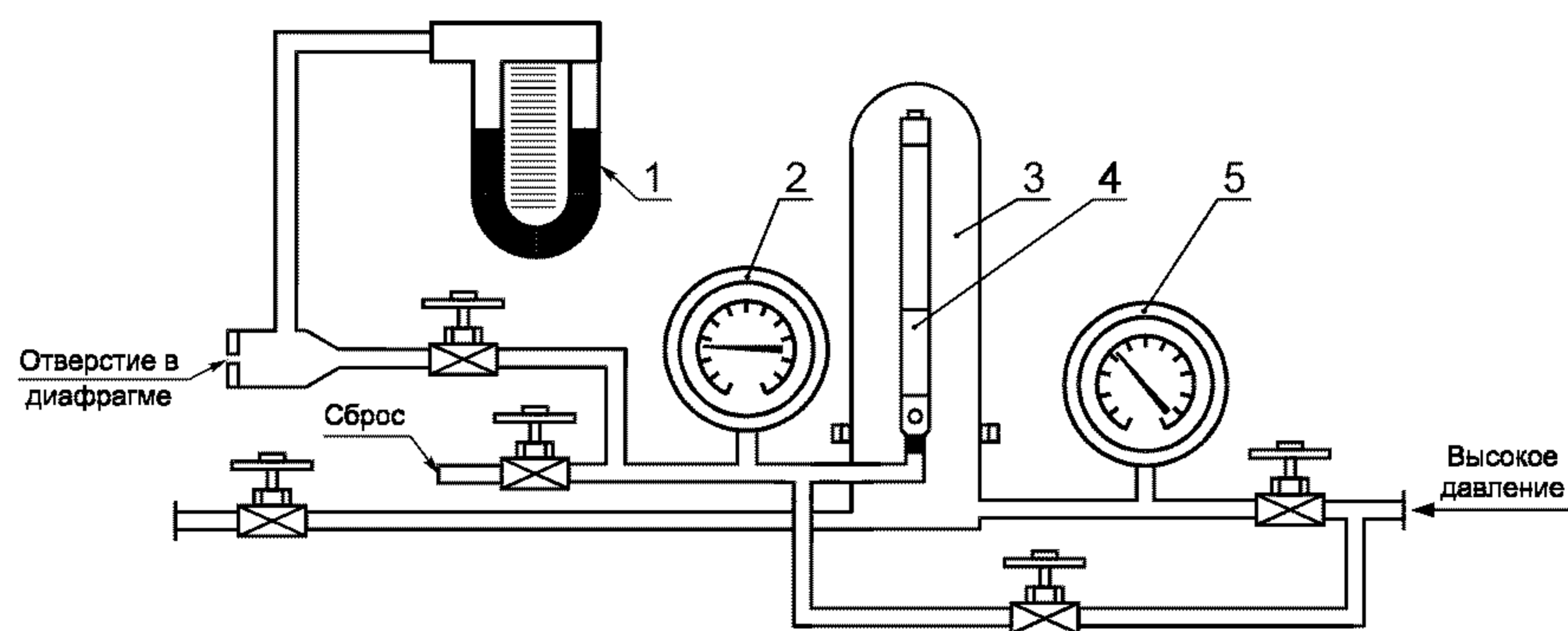
1, 2, 5 — манометры; 3 — камера давления; 4 — газлифтный клапан
