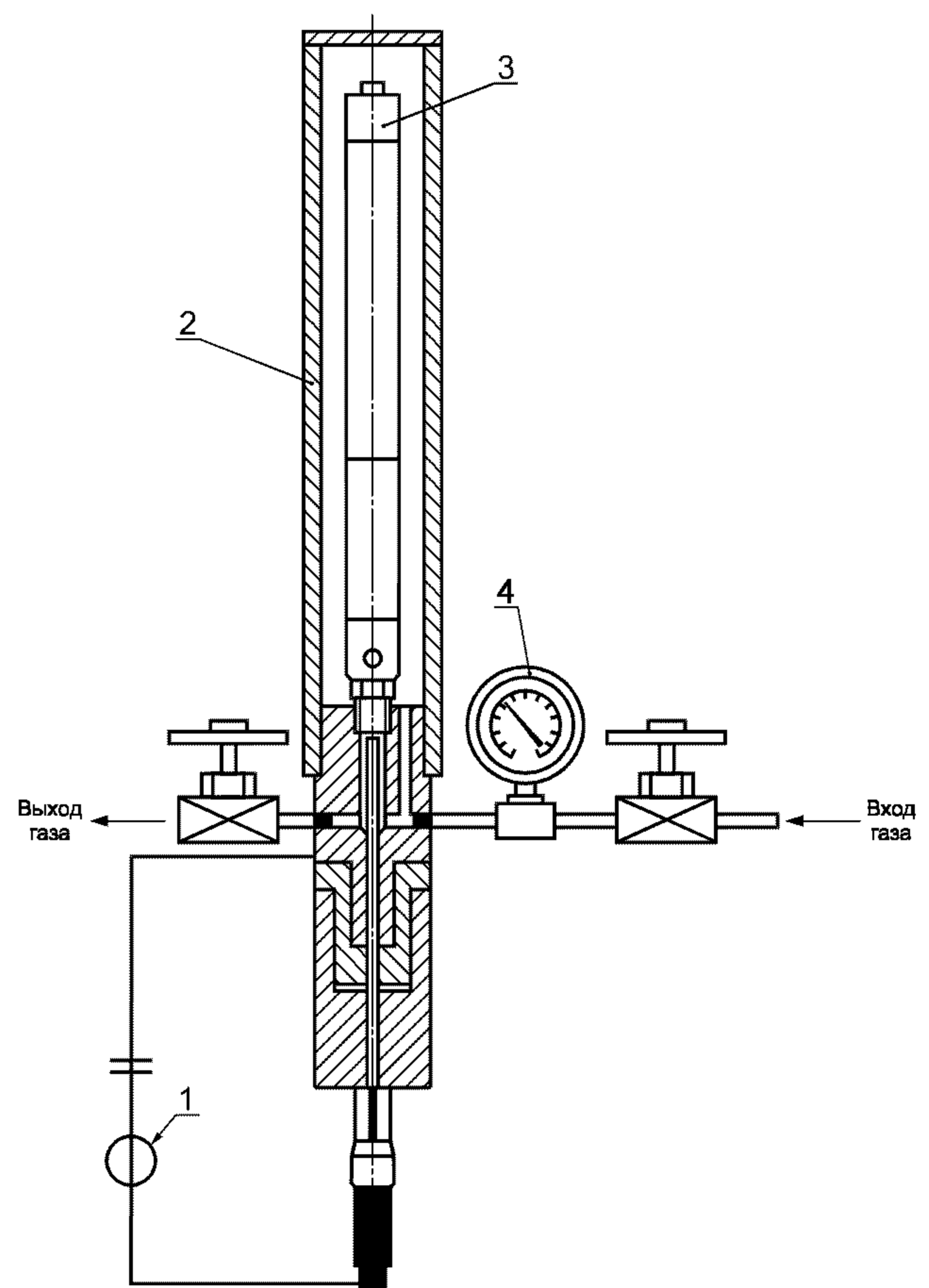
1 — омметр; 2 — камера давления; 3 — газлифтный клапан; 4 — манометр
