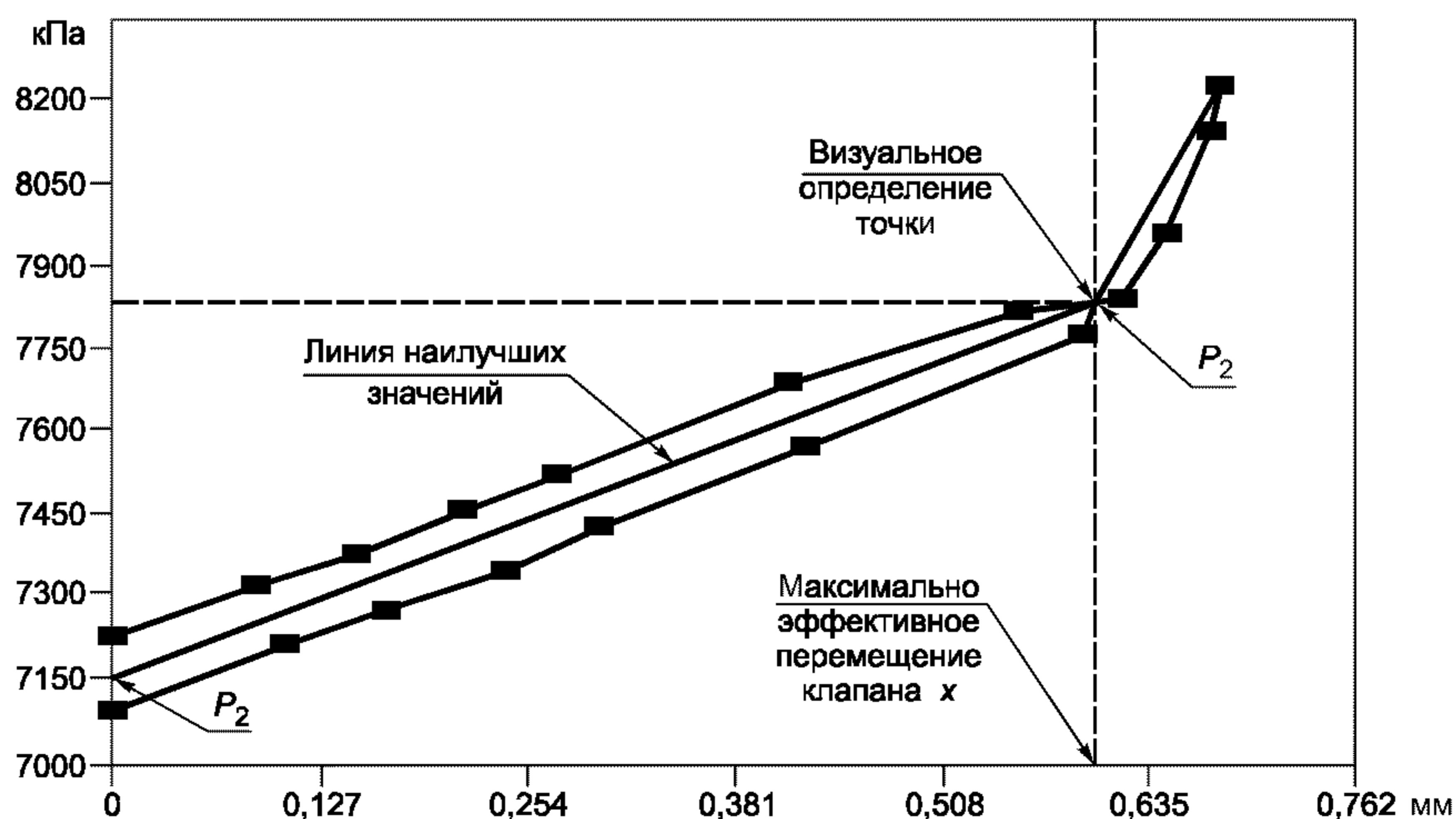
Рисунок 12 — Диаграммы перемещения штока в зависимости от коррозии клапана
