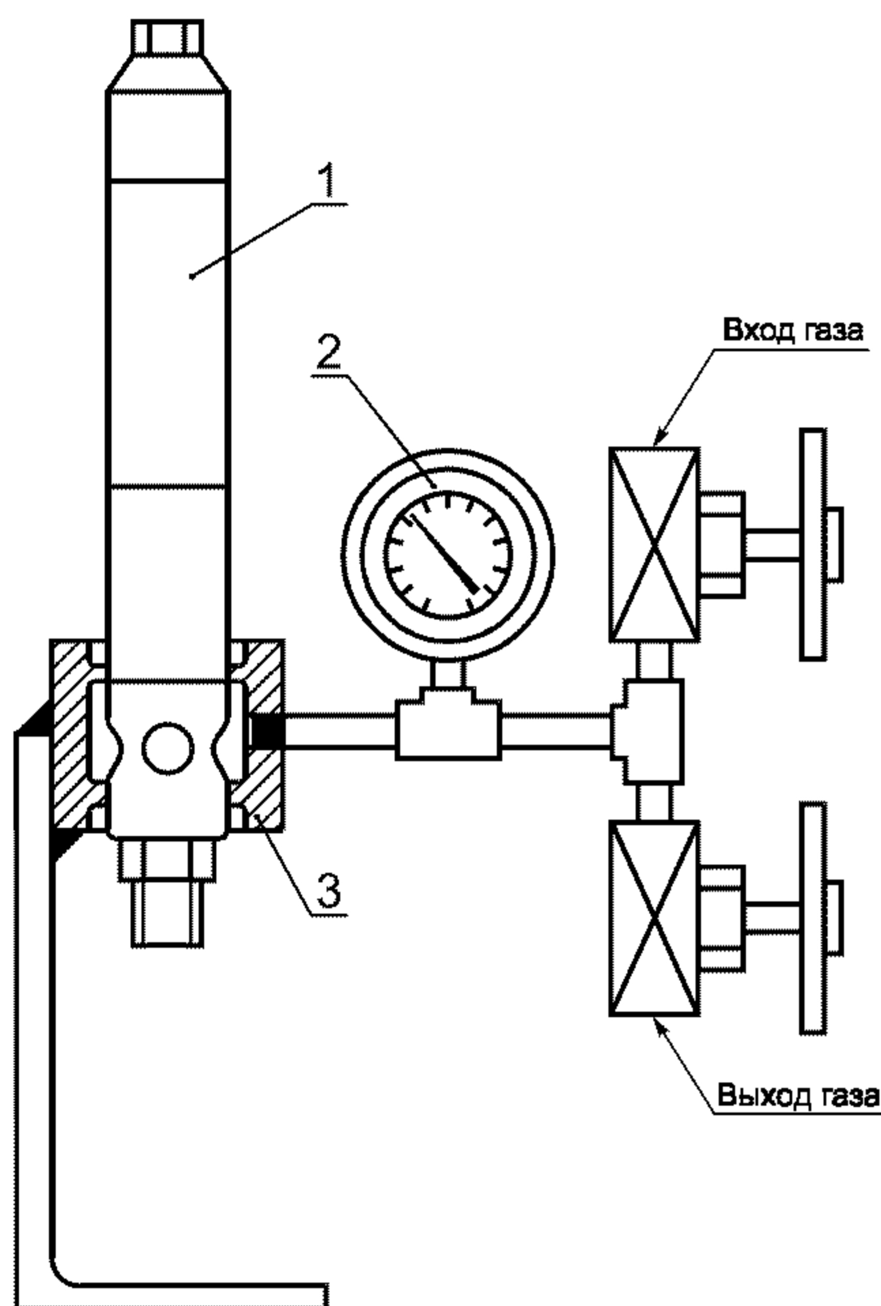
1 — испытуемый клапан; 2 — манометр; 3 — гильза
