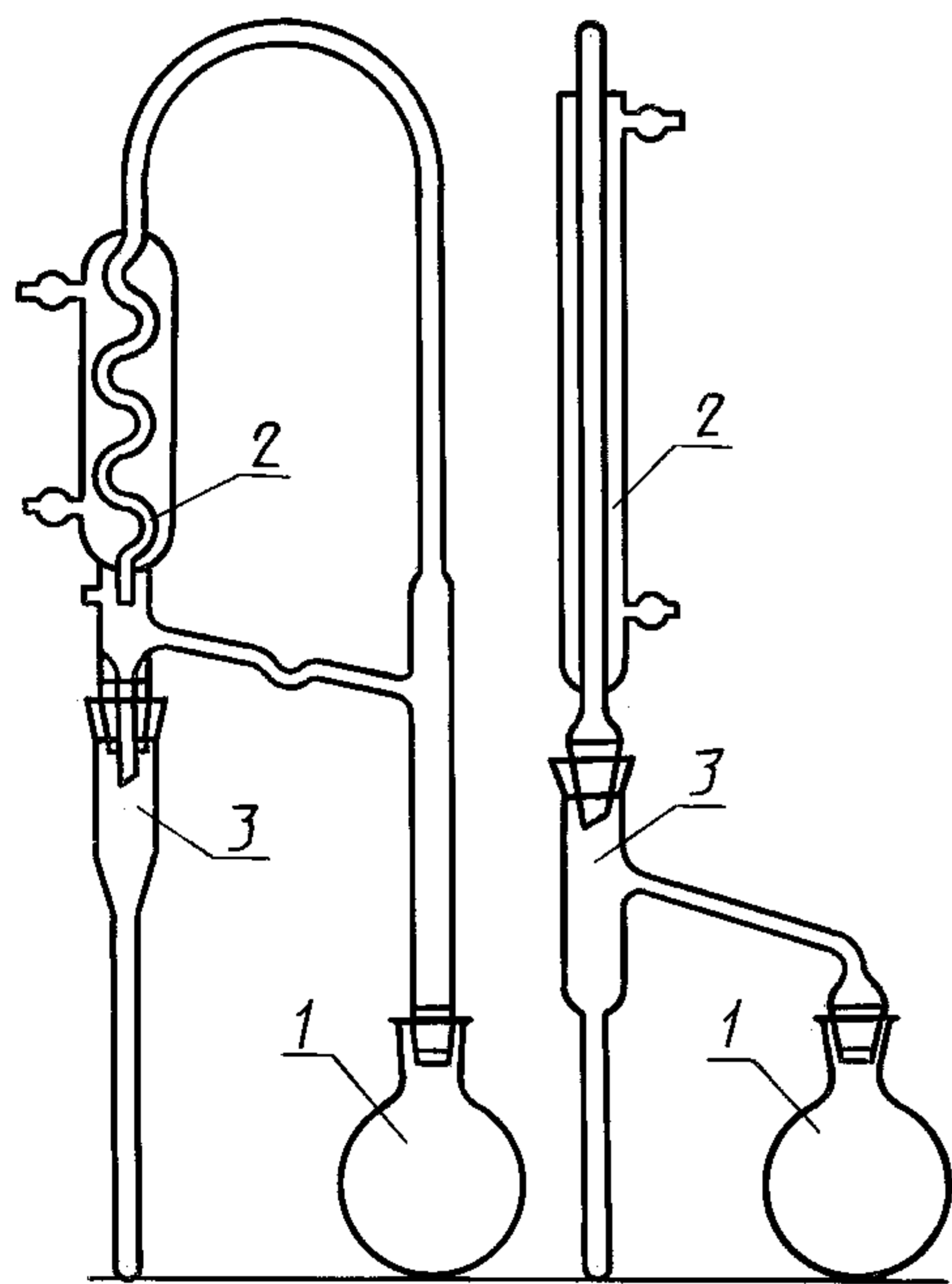
1 — колба для перегонки; 2 — холодильник; 3 — приемник
