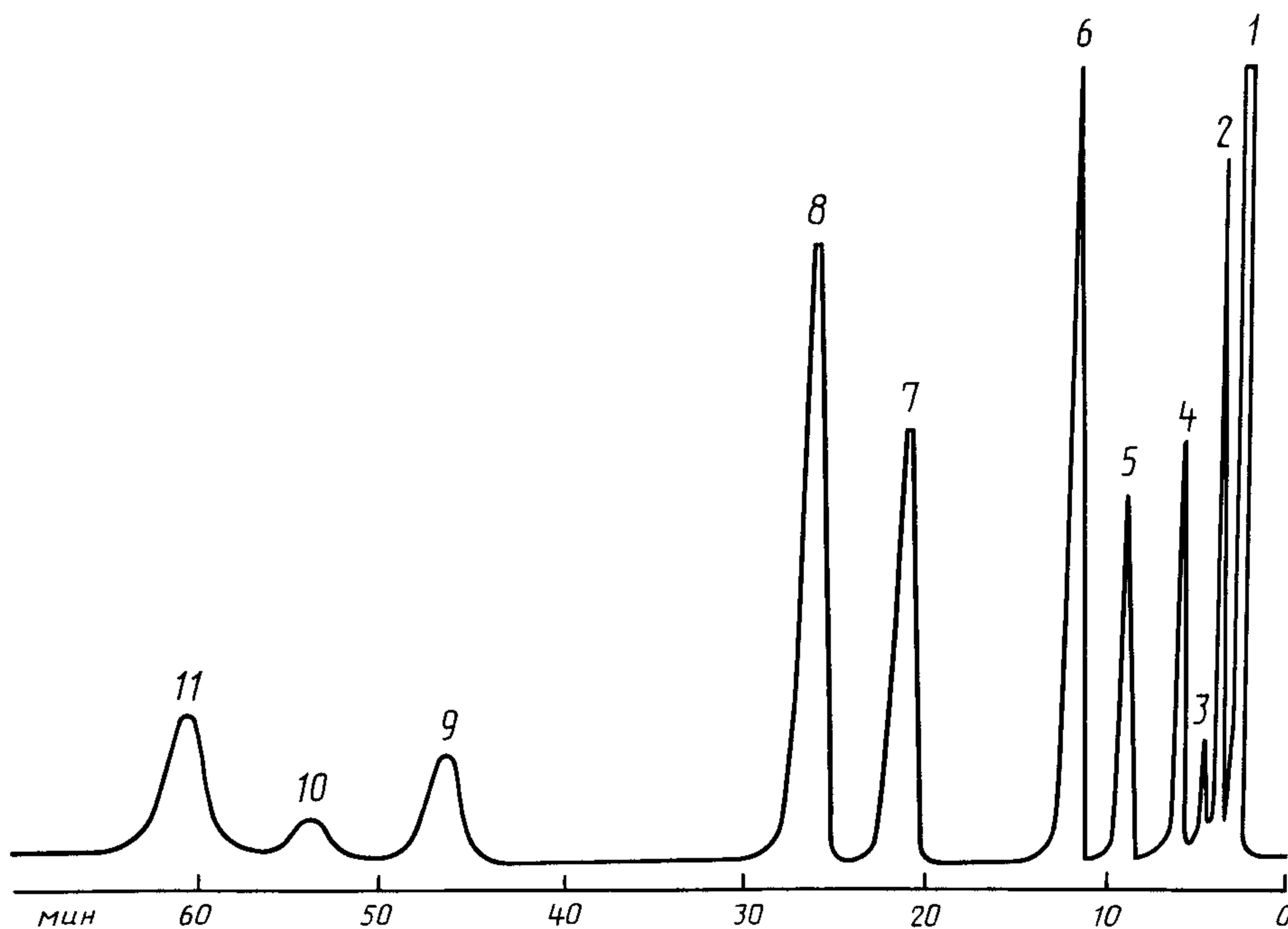
1 — метан+неуглеводородные газы; 2 — этан; 3 — диоксид углерода; 4 — пропан; 5 — i -бутан; 6 — n -бутан; 7 — i -пентан; 8 — n -пентан; 9 — 2-метилпентан+2,3-диметилбутан; 10 — 3-метилпентан; 11 — n -гексан
