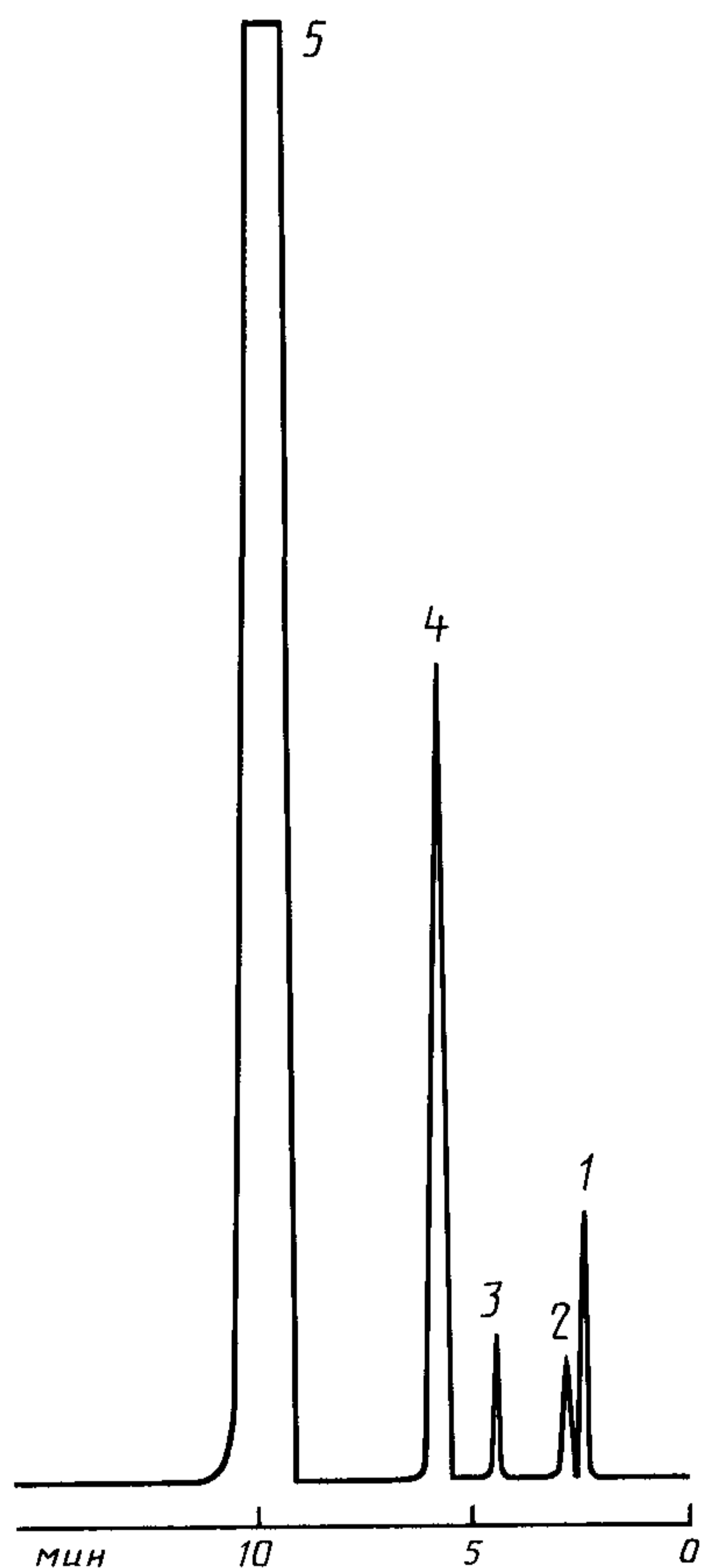
1 — гелий; 2 — водород; 3 — кислород; 4 — азот; 5 — метан
