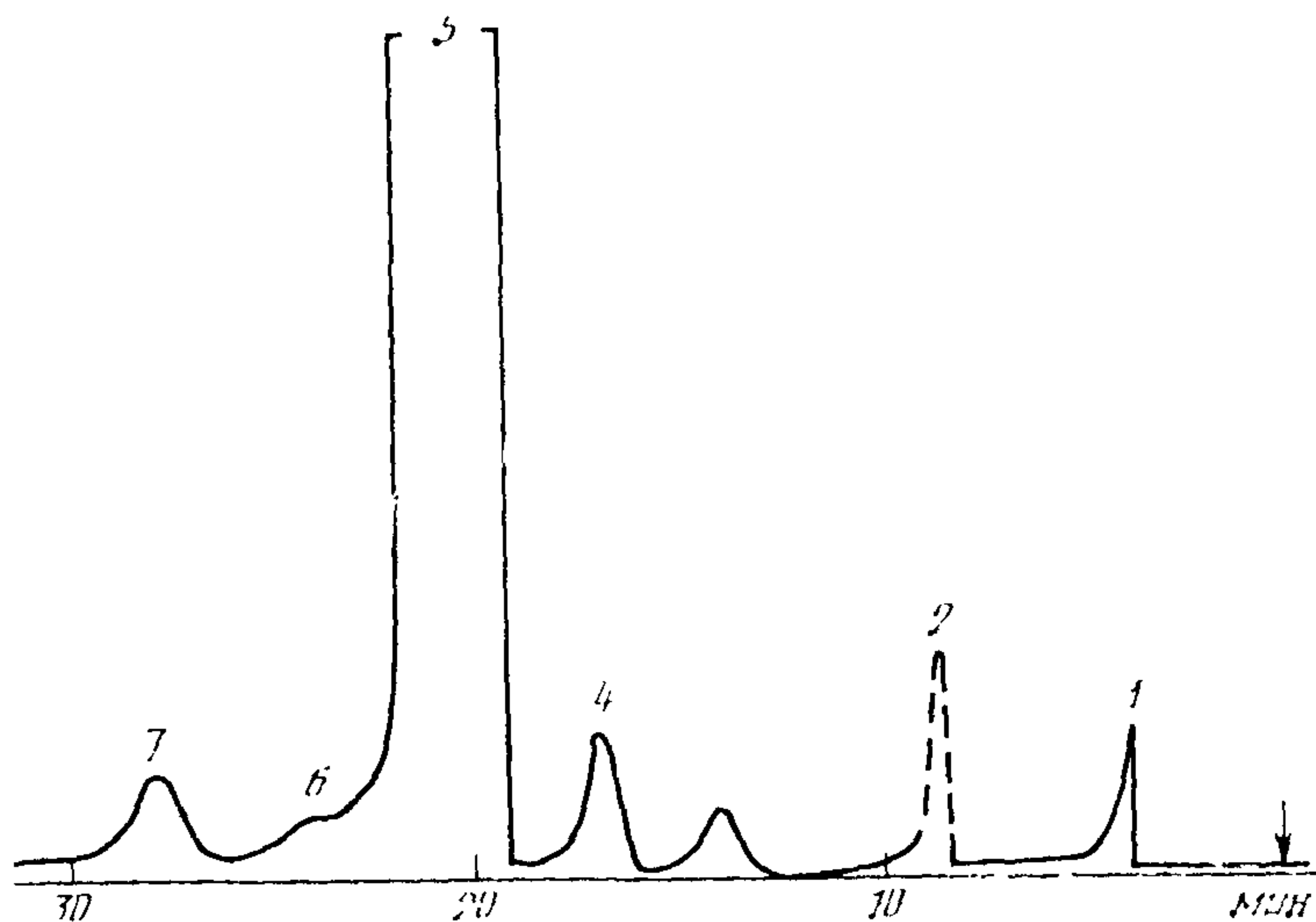
Типовая хроматограмма o -крезола
