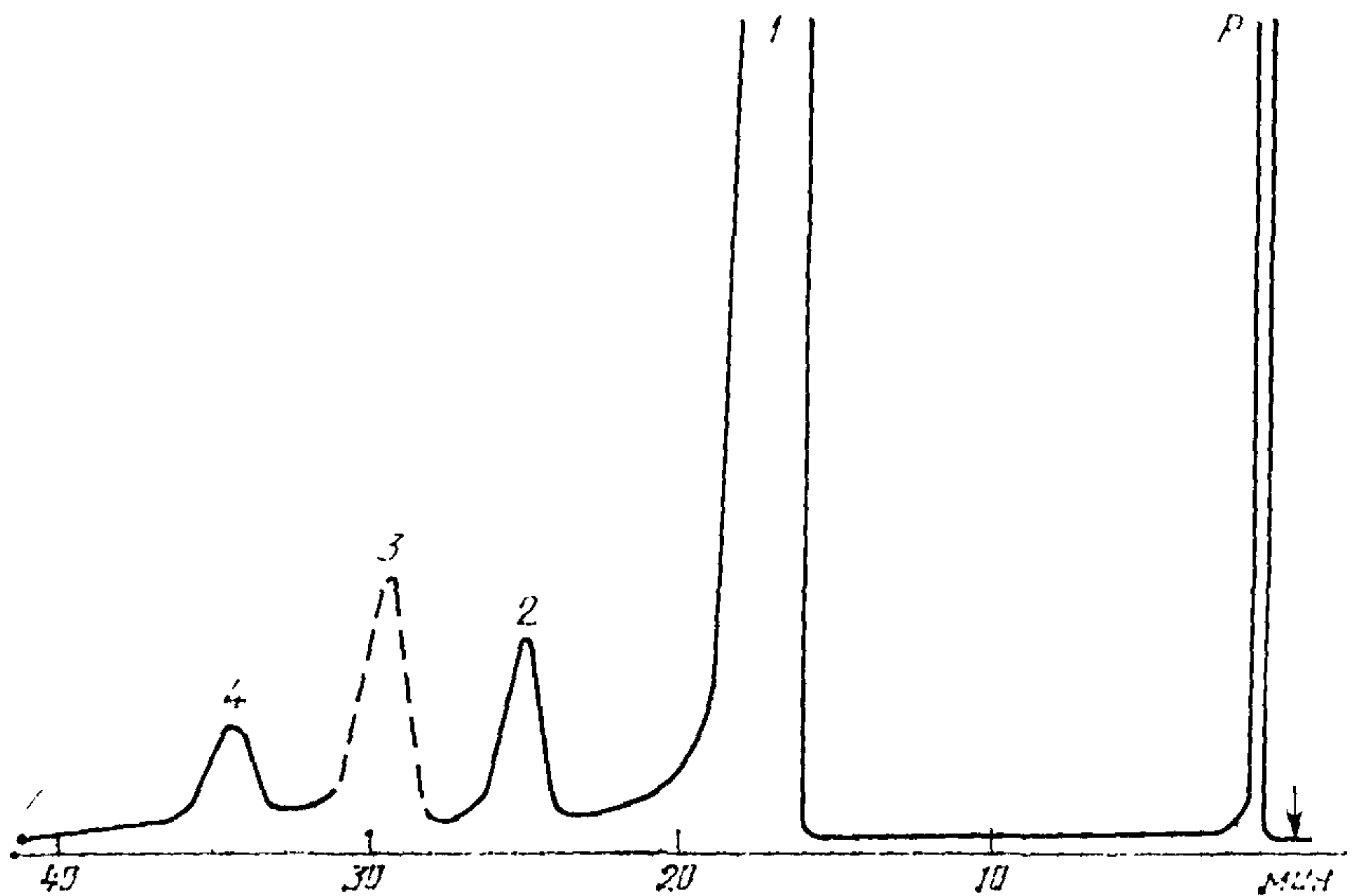
Типовая хроматограмма фенола
