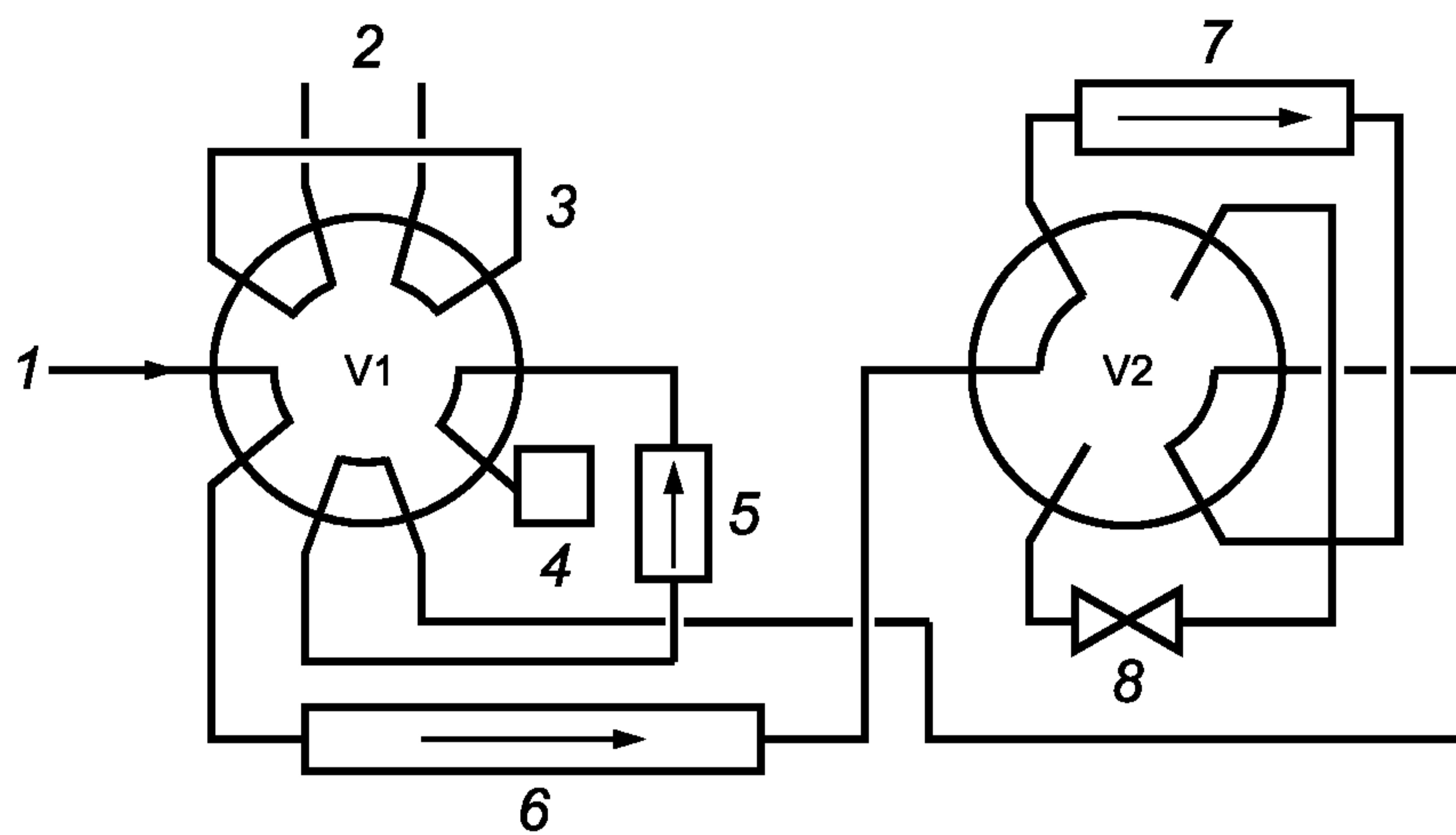
a — Кран 1 (V1) в положении 1 и кран 2 (V2) в положении 1
