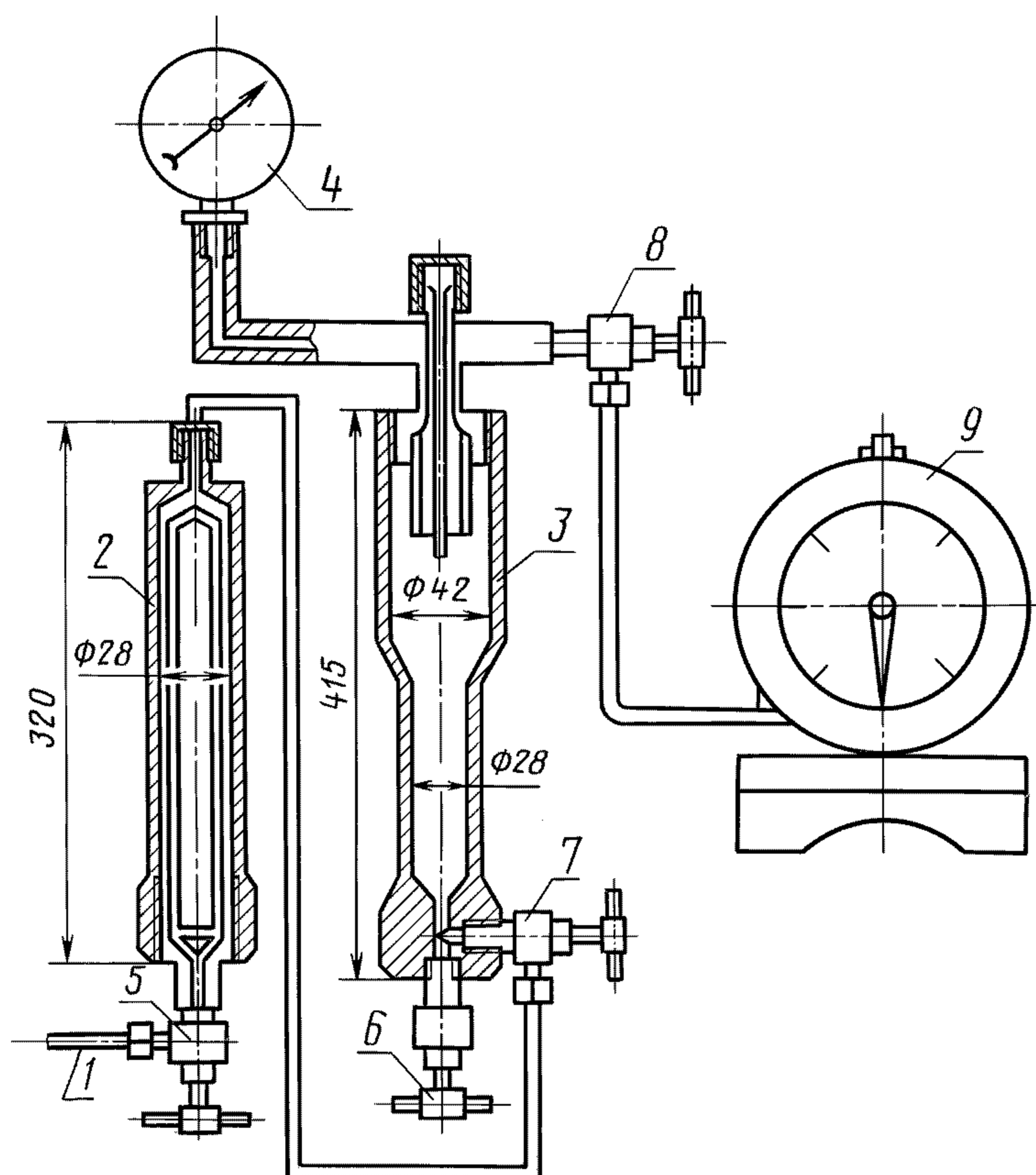
1 — вход газа; 2 — фильтр-патрон; 3 — абсорбционный сосуд; 4 — манометр; 5, 6, 7, 8 — запорные вентили; 9 — газовый счетчик
