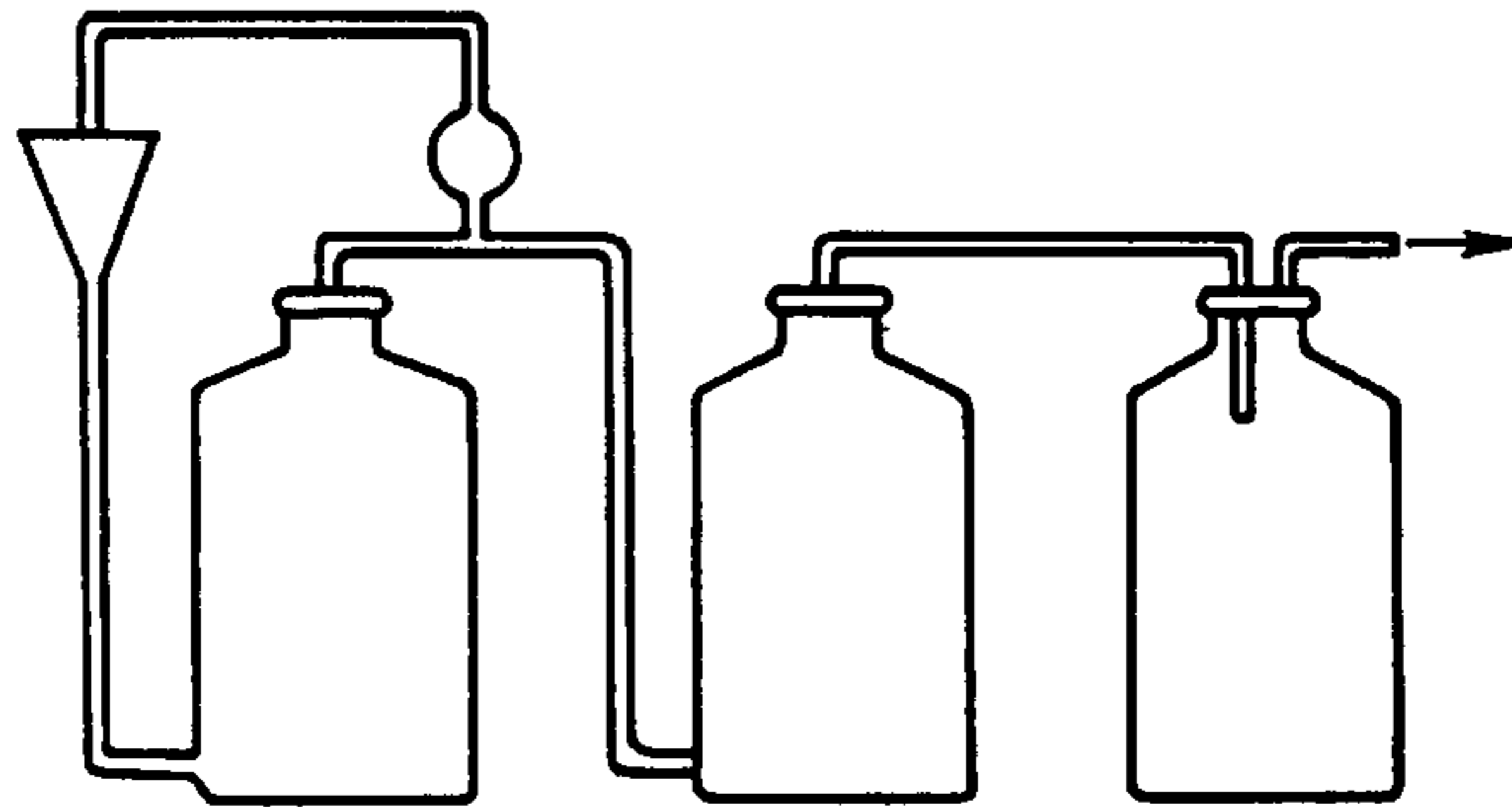
Установка для удаления ртути из сточных растворов
