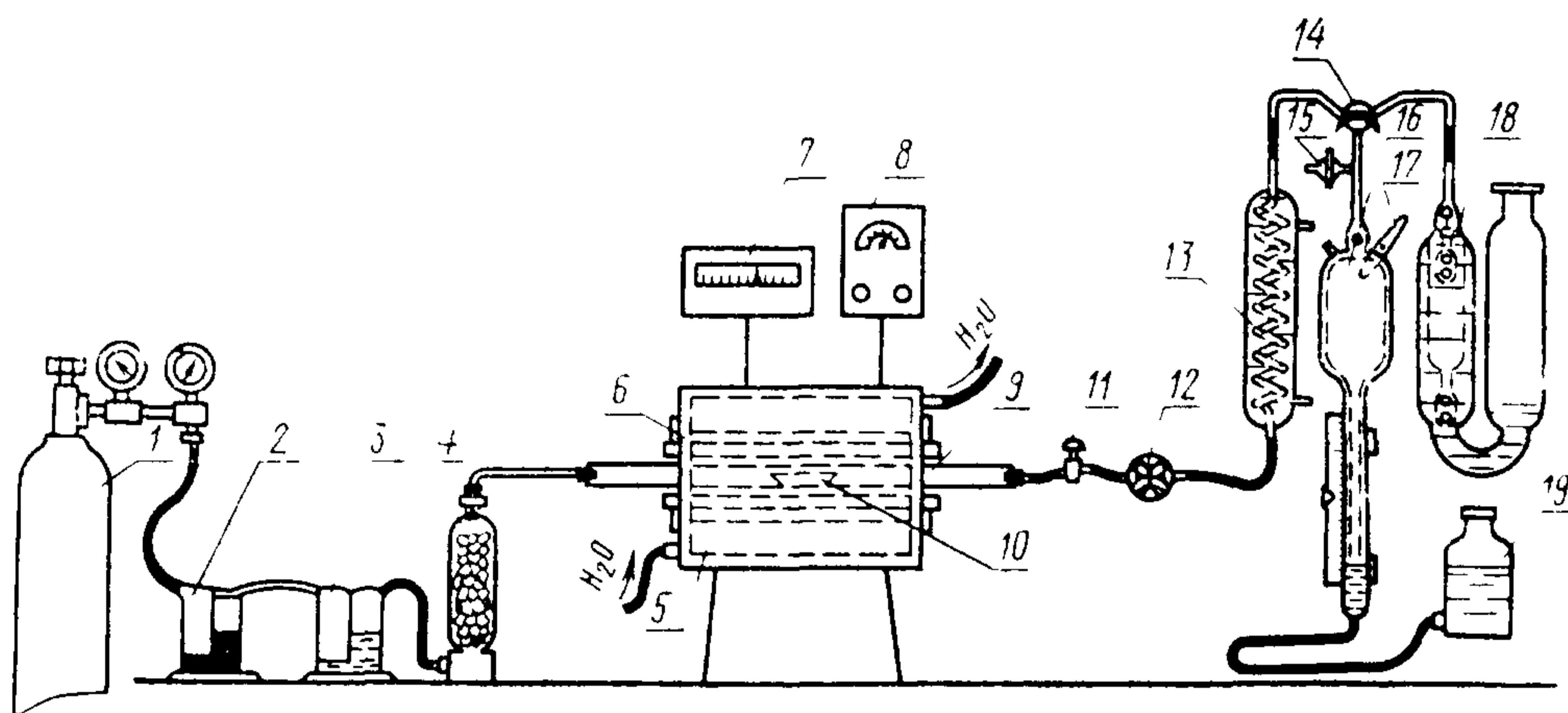
Установка для газообъемного определения содержания углерода
