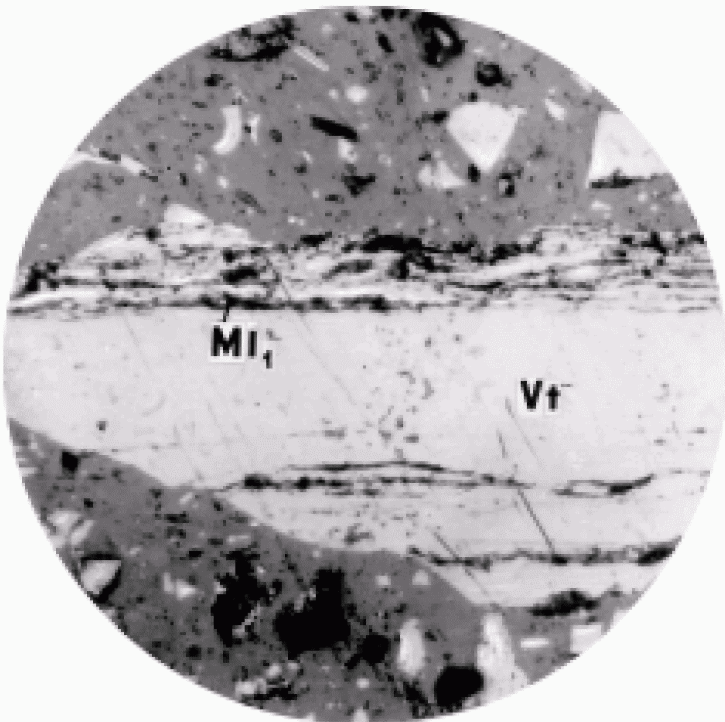
Сросток микролитотипа 1-й группы ( V_t ) + + аргиллит ( MI_1 )
