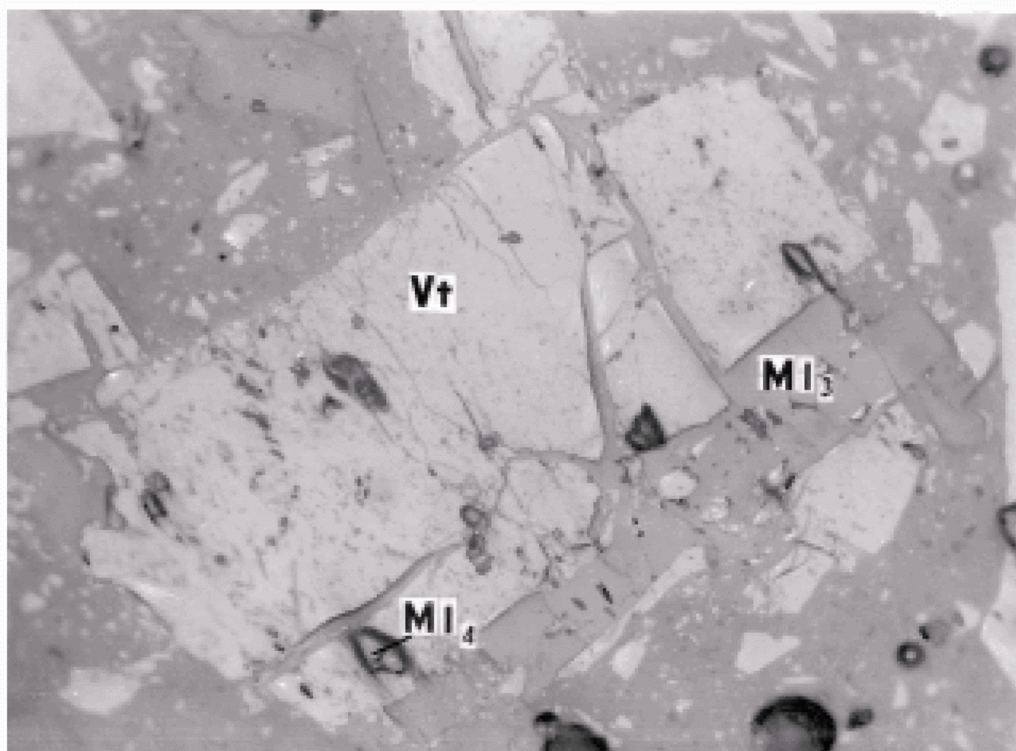
Сросток микролитотипа 1-й группы ( V_t ) + сидерит ( Ml_3 ) + кварц ( Ml_4 )
