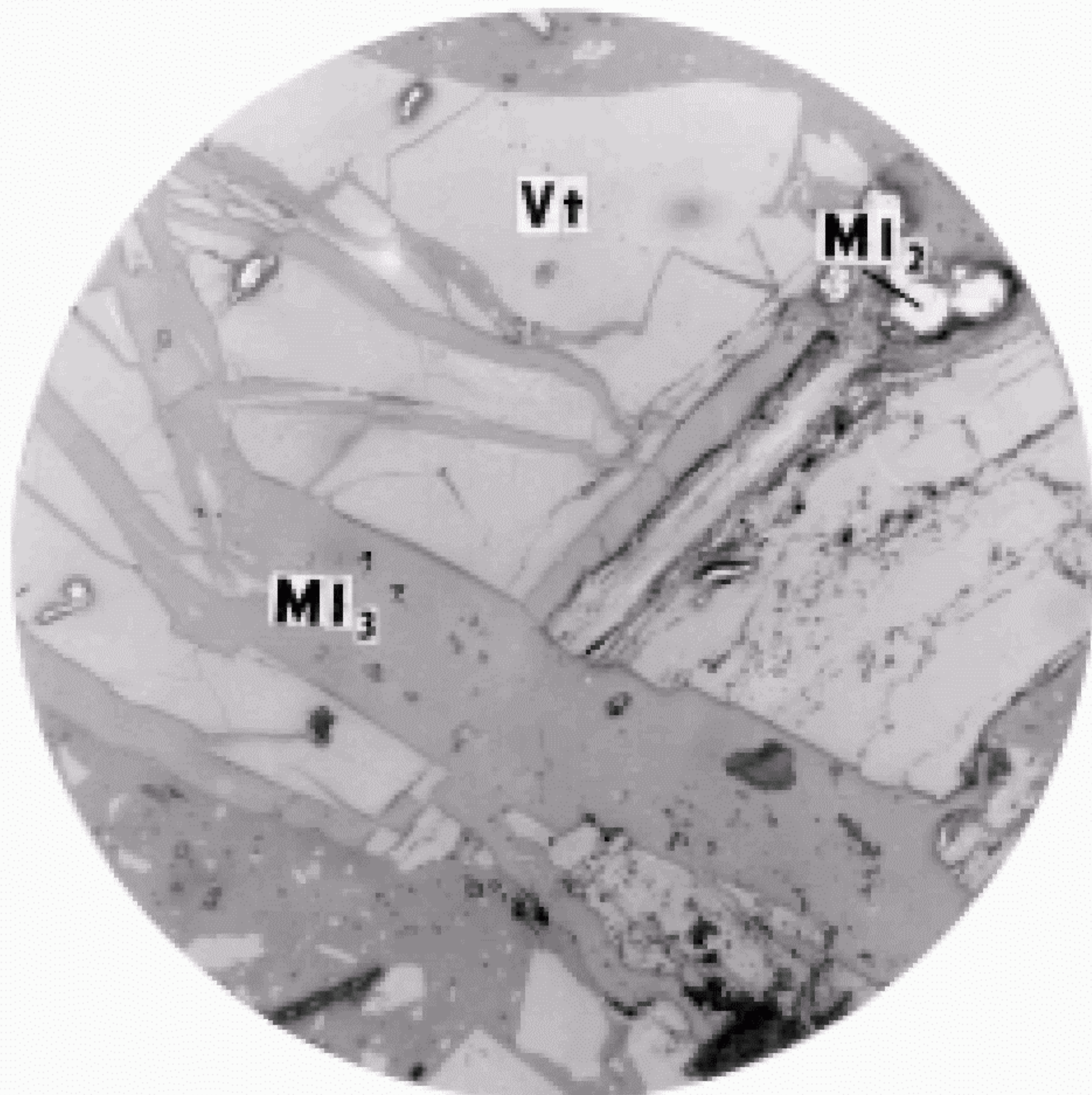
Сросток микролитотипа 1-й группы ( V_t ) + пирит ( Ml_2 ) + кальцит ( Ml_3 )
