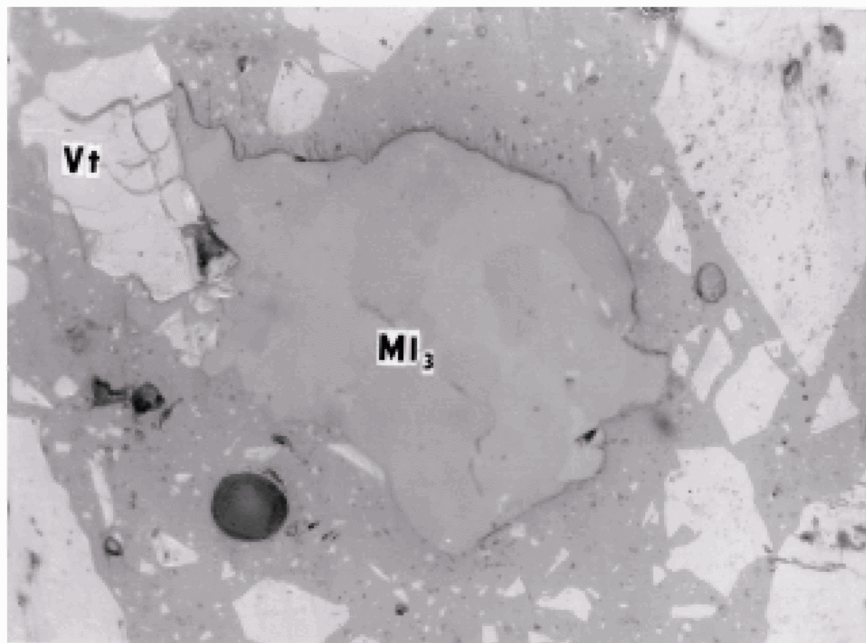
Сросток микролитотипа 1-й группы ( V_f ) + сидерит ( MI_3 )
