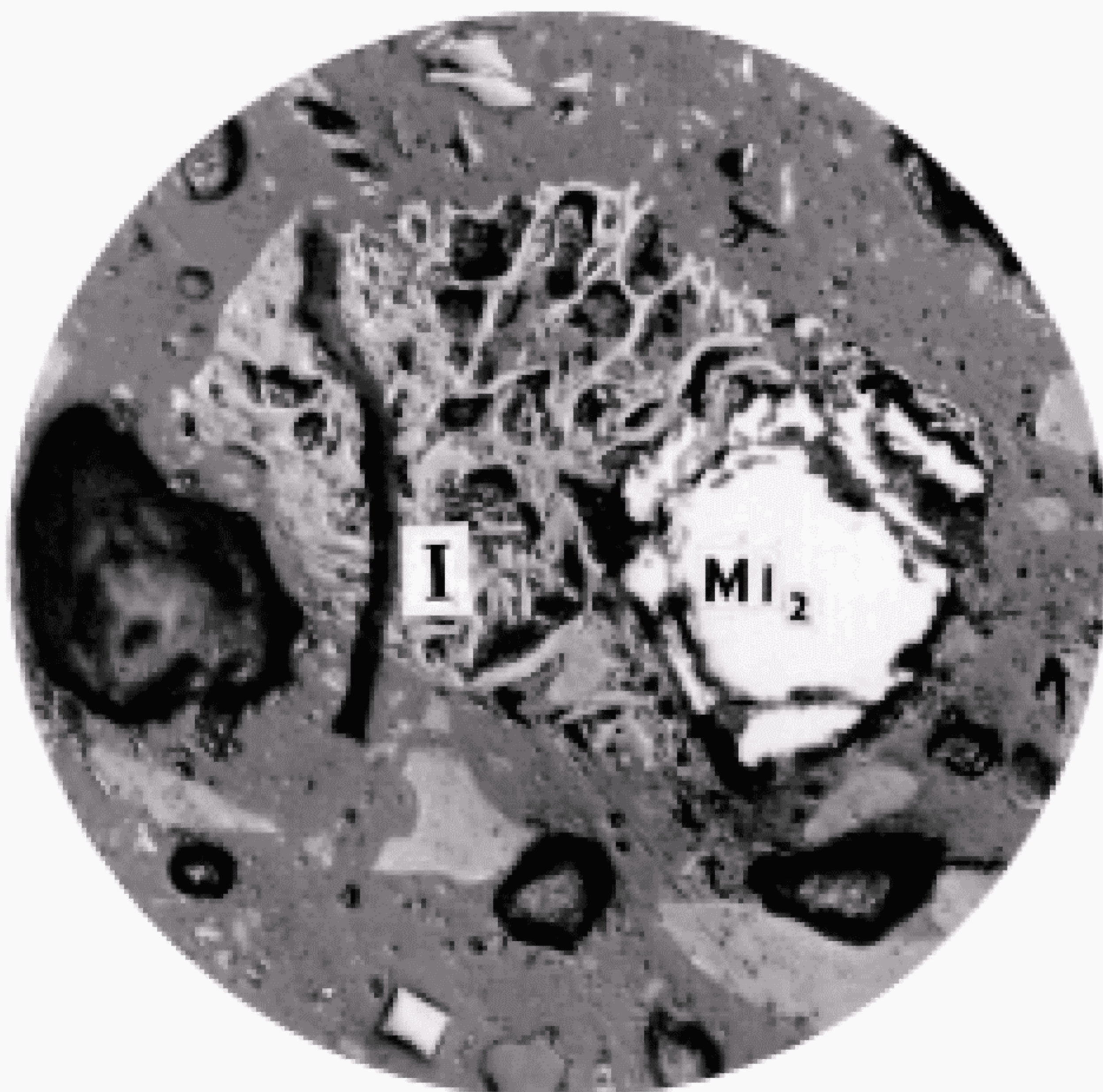
Сросток микролитотипа 3-й группы ( F ) + + пирит ( MI_2 )
