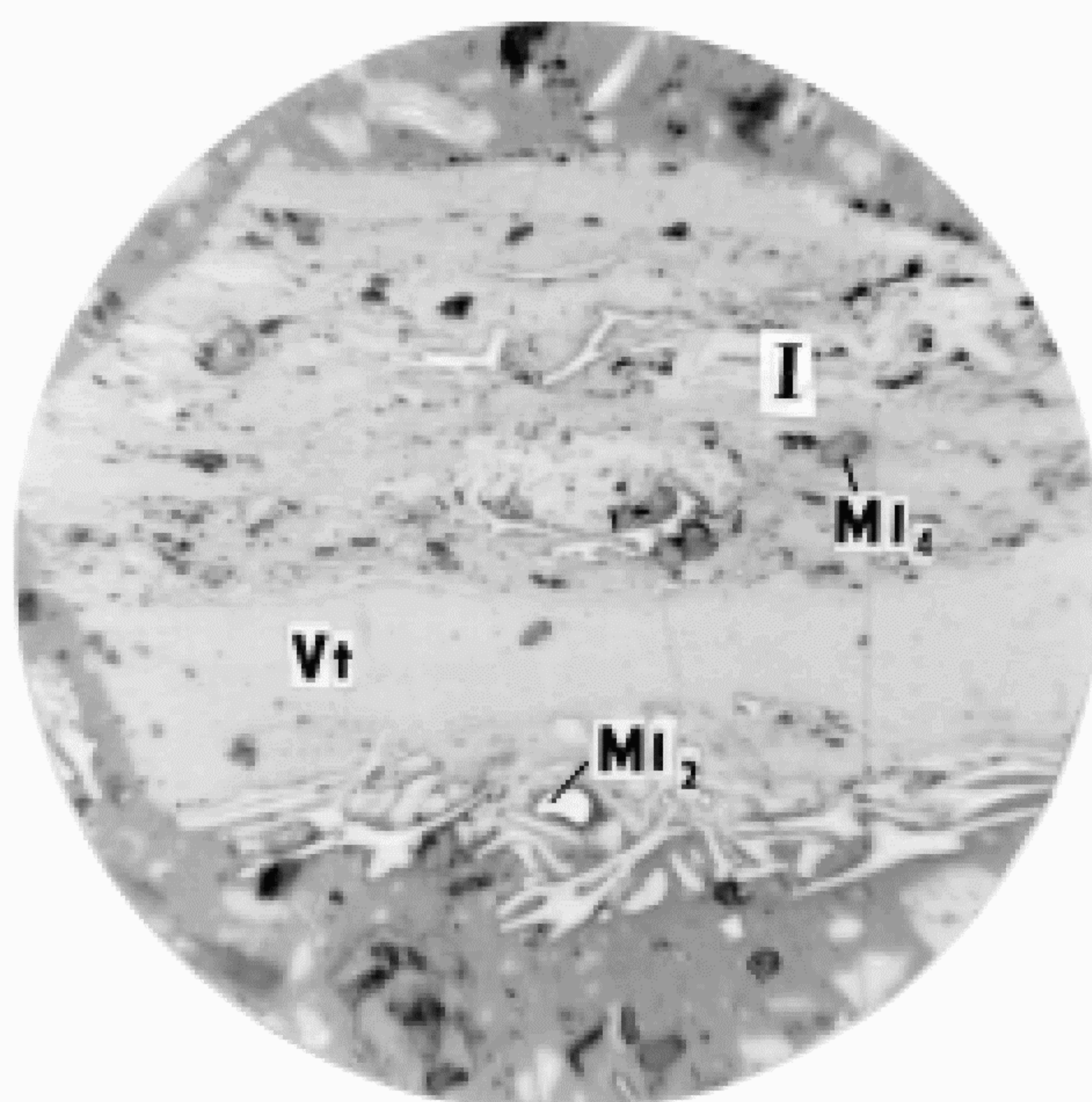
Сросток микролитотипа 2-й группы (V 1 + F) + + кварц (MI 4 ) + пирит (MI 2 )
