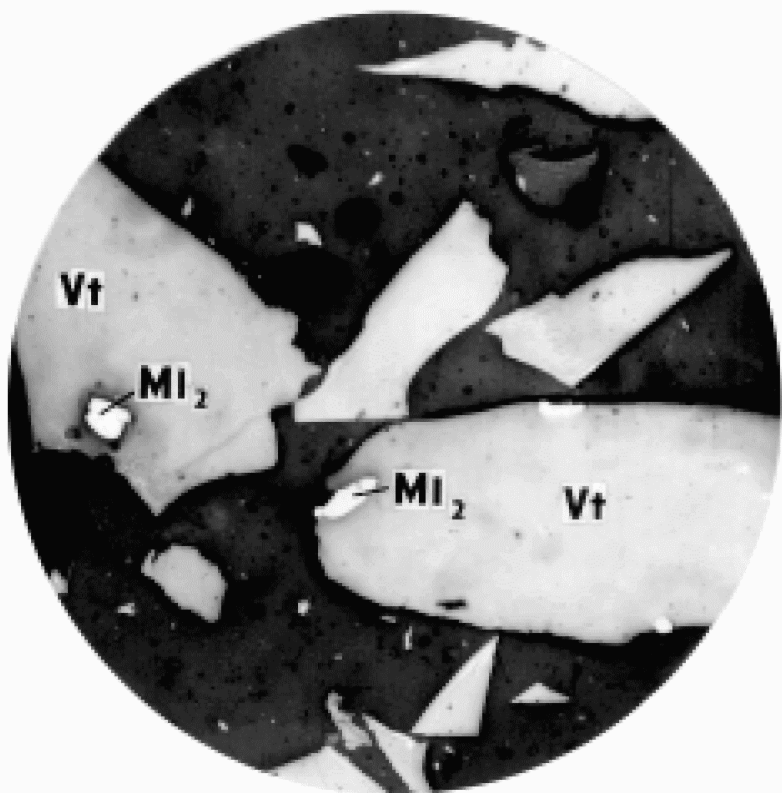
Сростки микролитотипов 1-й группы (V 1 ) + + пирит (MI 2 )
