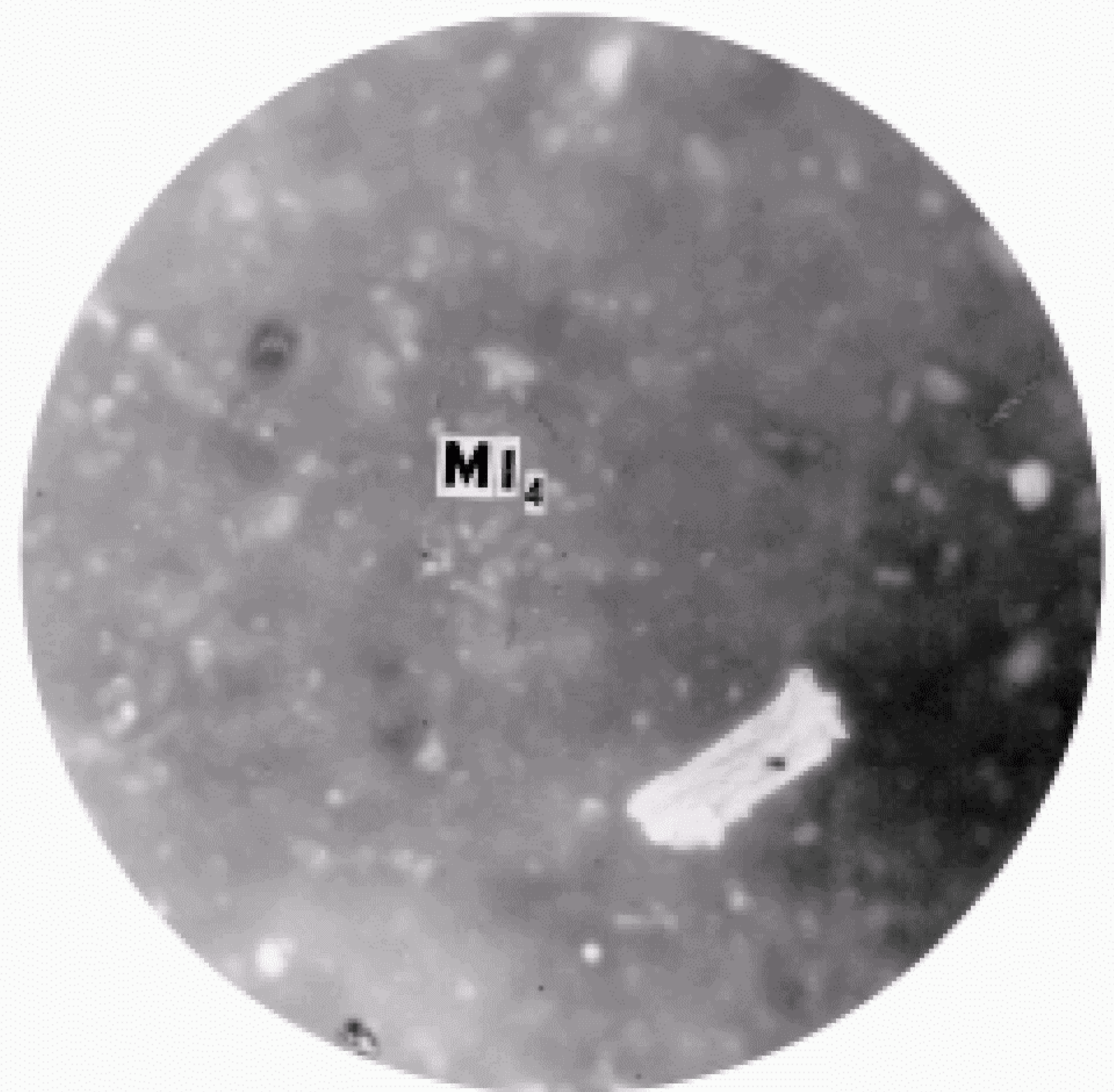
Известняк (M1 4 ) (увеличение 200)
