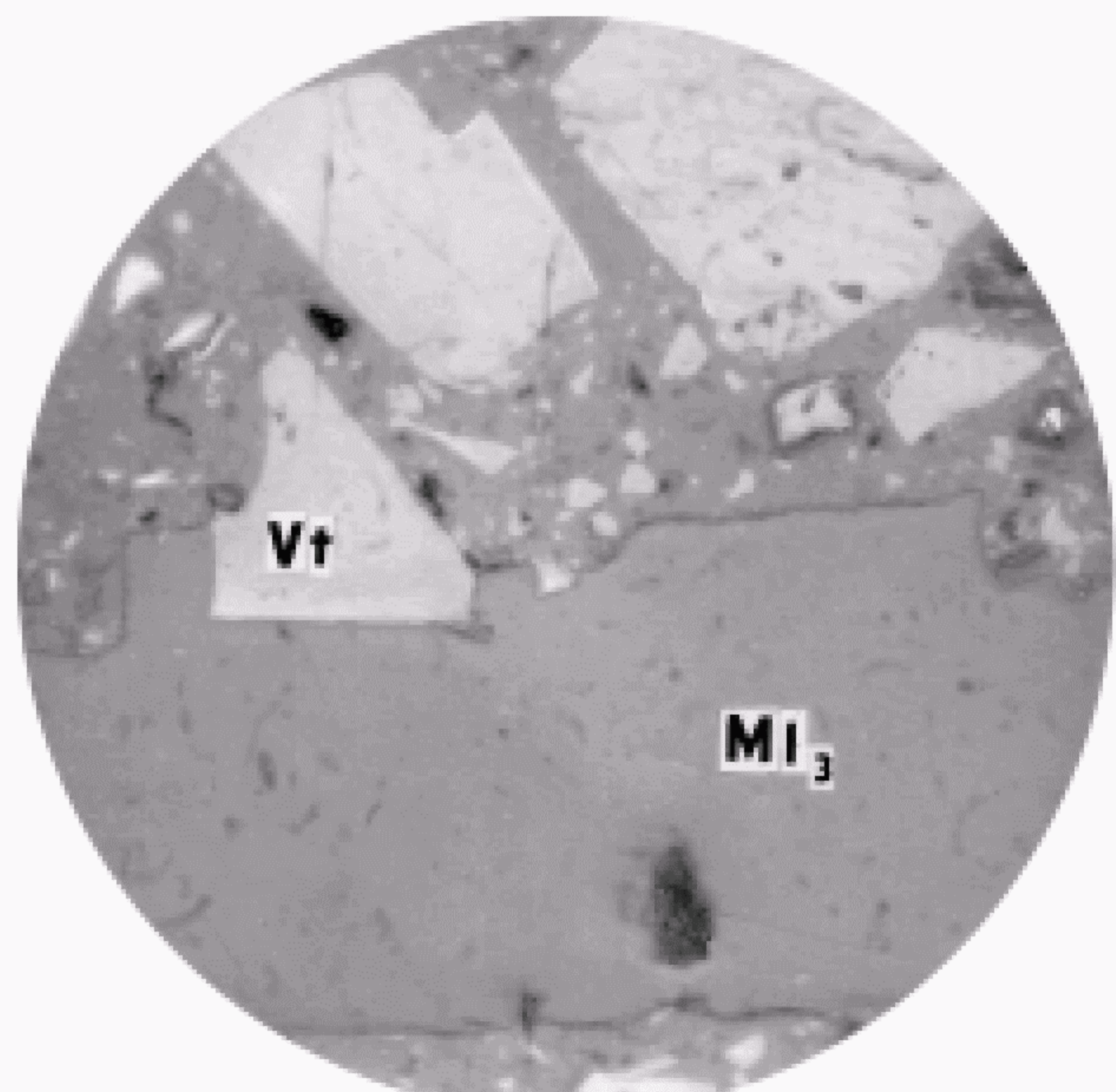
Сросток микролитотипа 1-й группы ( V_t ) + + кальцит ( MI_3 )
