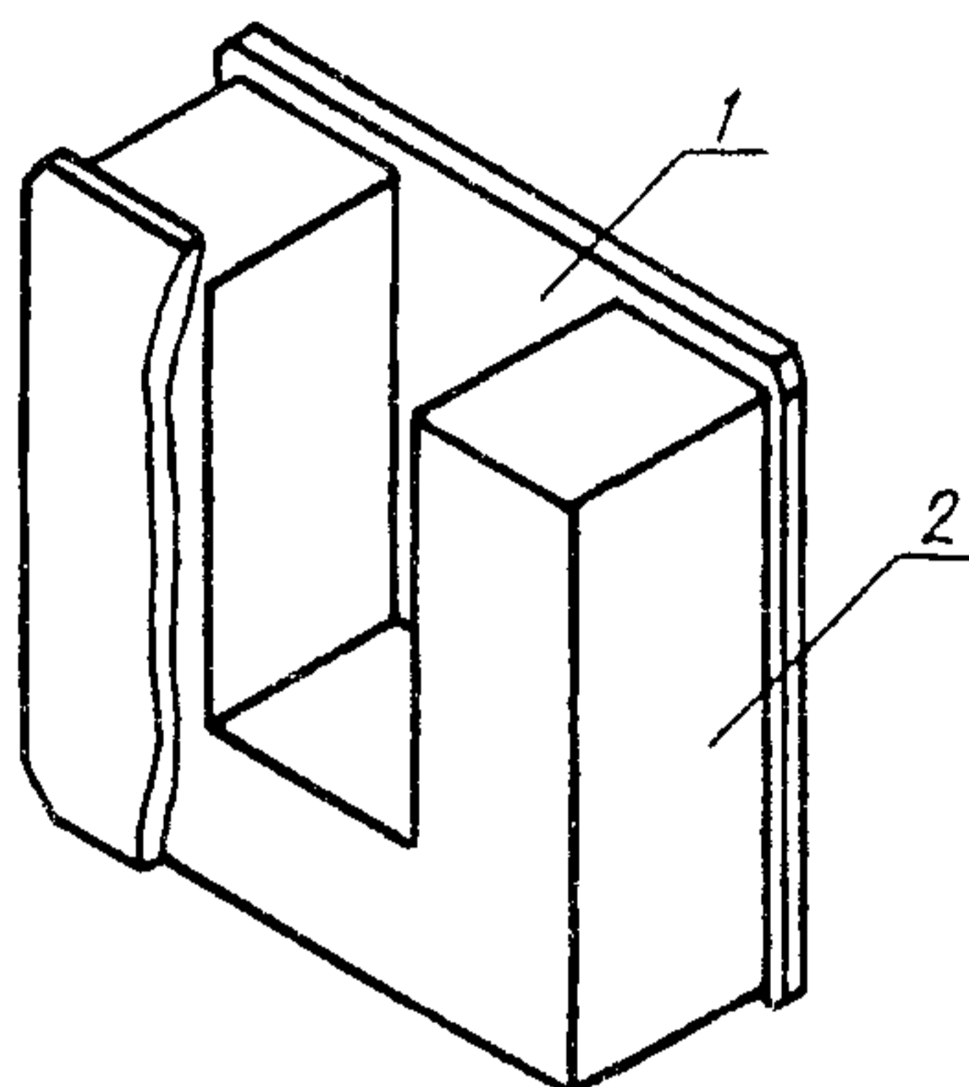
Форма № 1 для заливки образца
