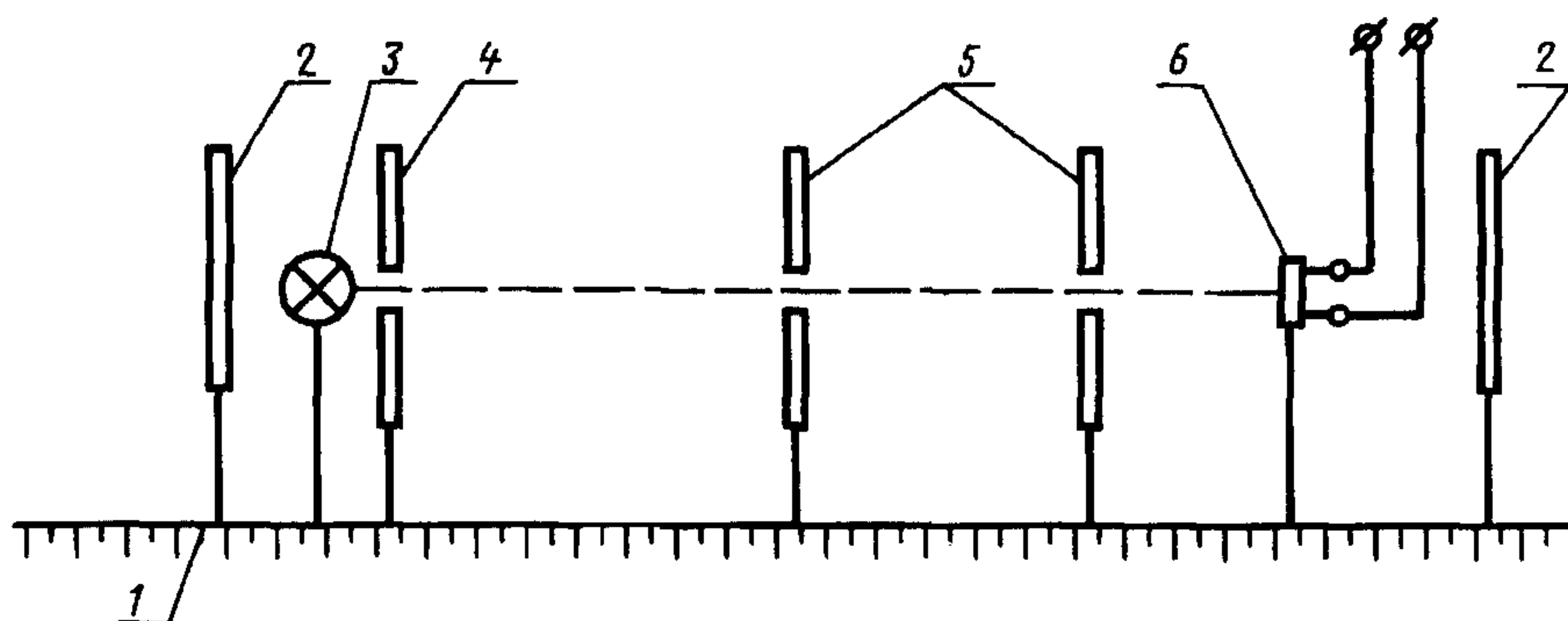
Схема градуировки светоизмерительной аппаратуры
