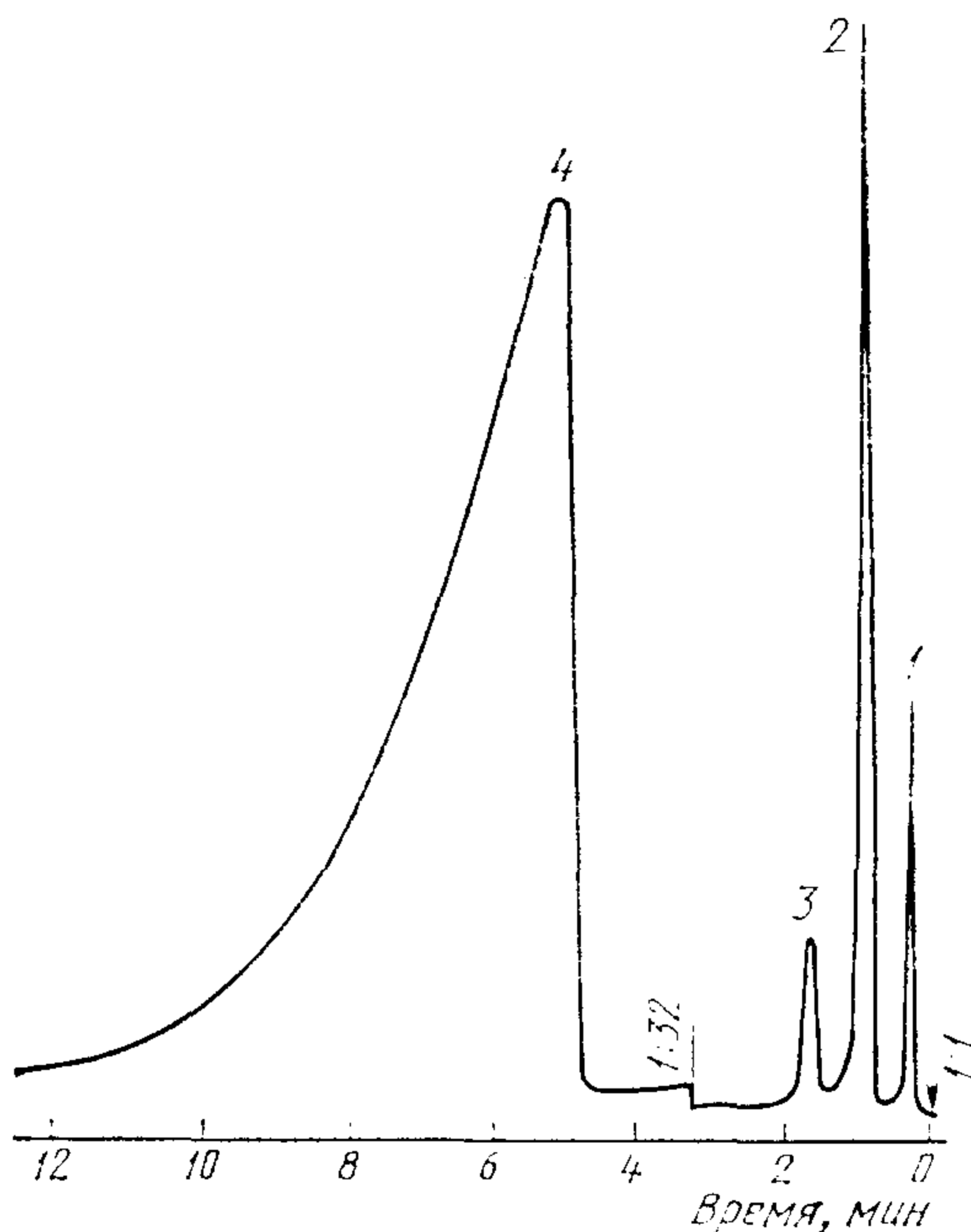
Типовая хроматограмма анализа ацетона
