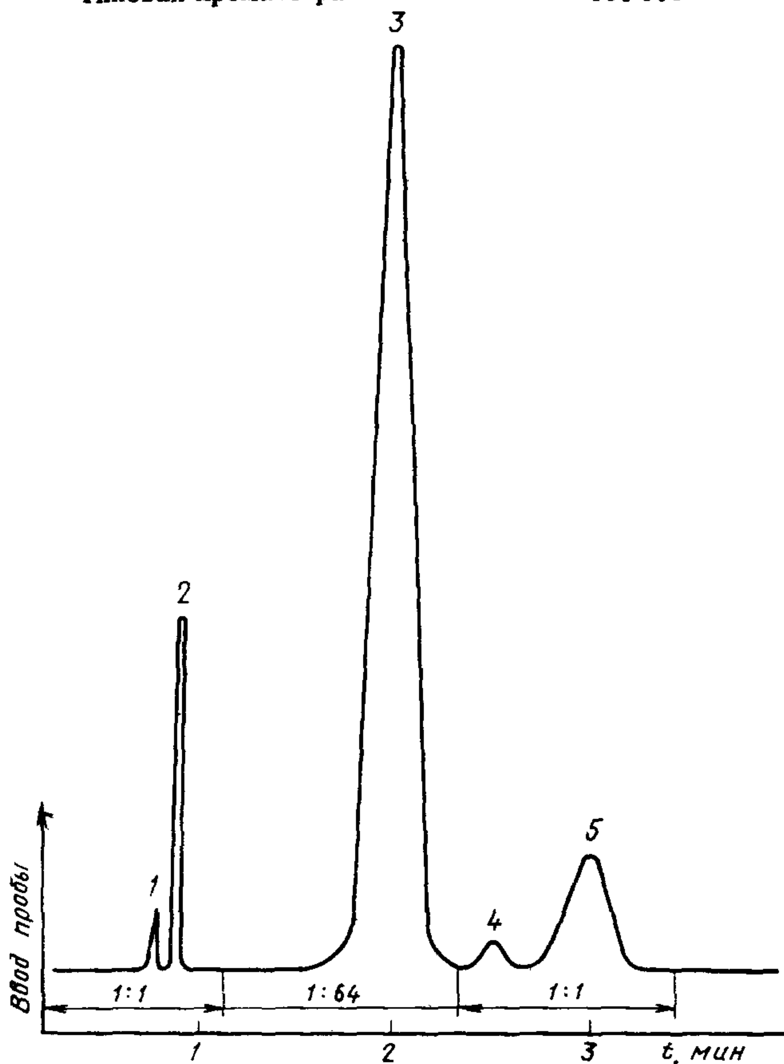
Типовая хроматограмма технического фурфурола
