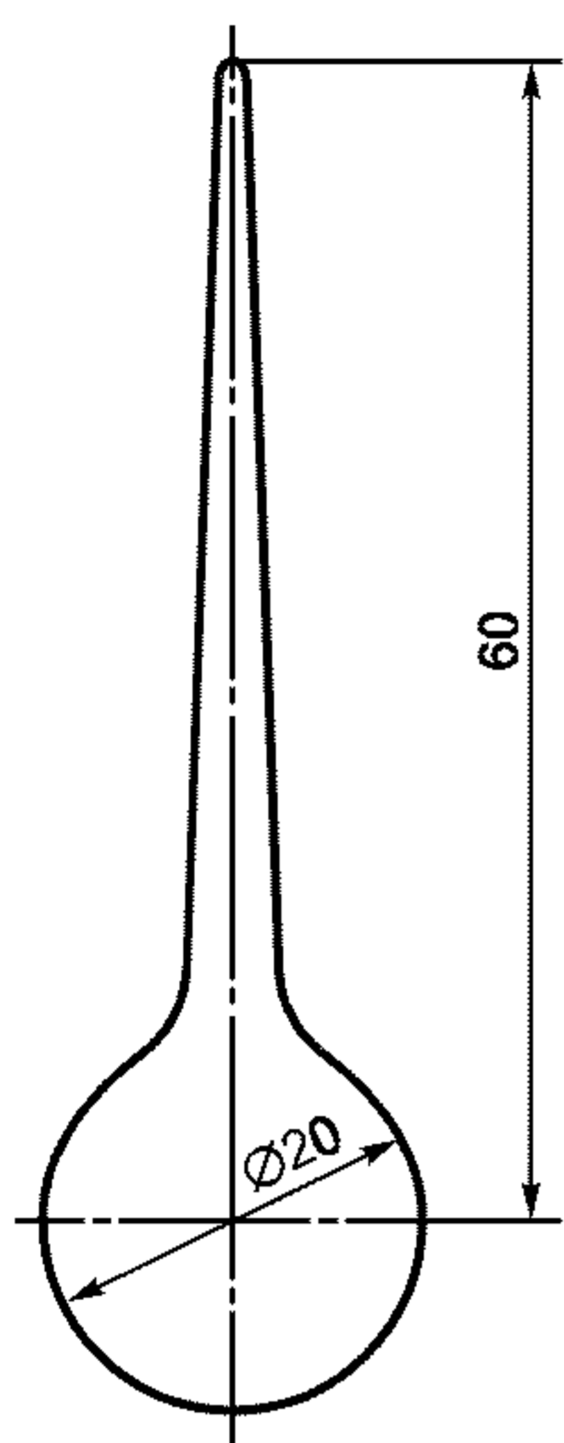
Рисунок 1 — Ампула стеклянная сферическая
