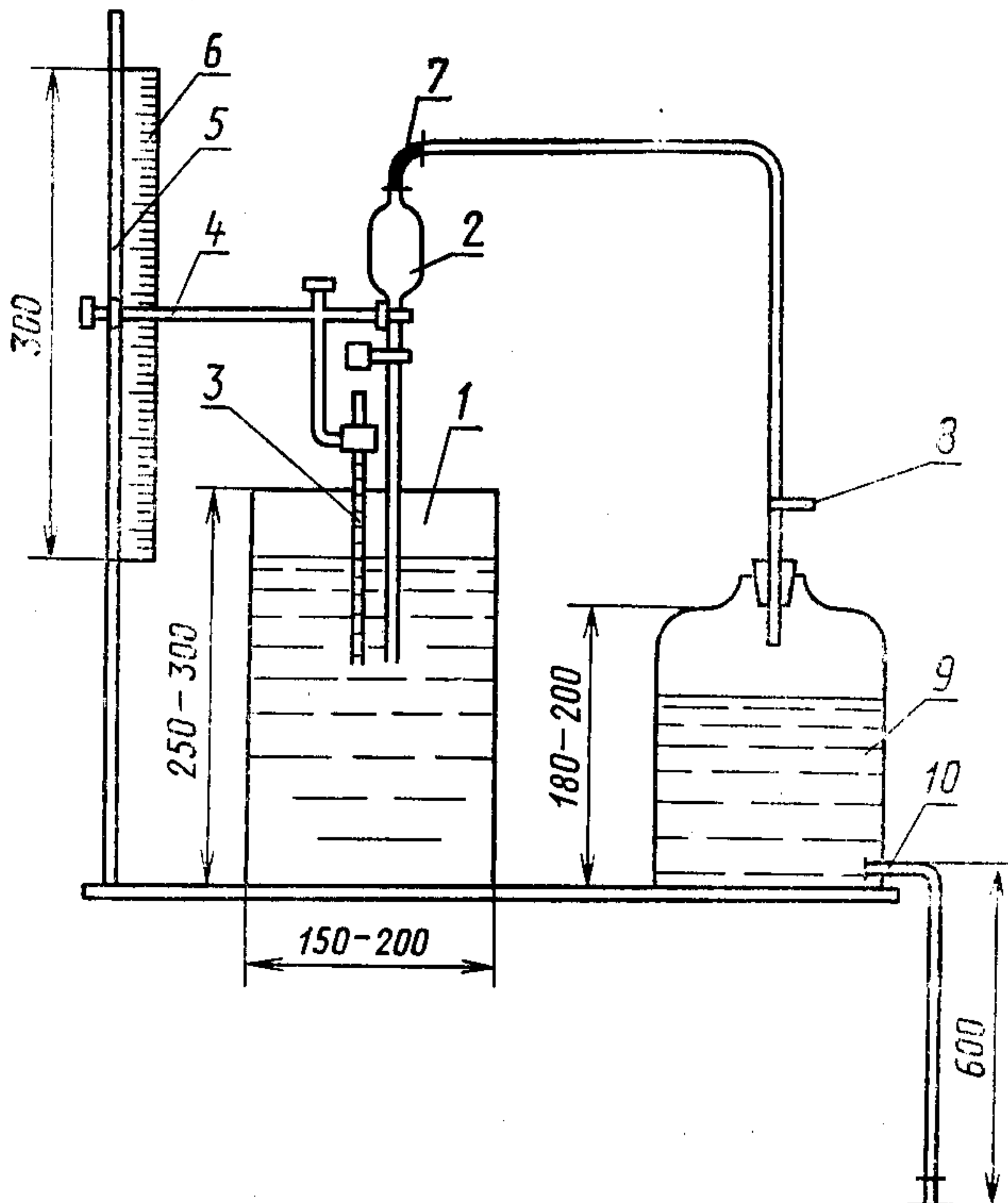
Установка для определения фракционного состава
