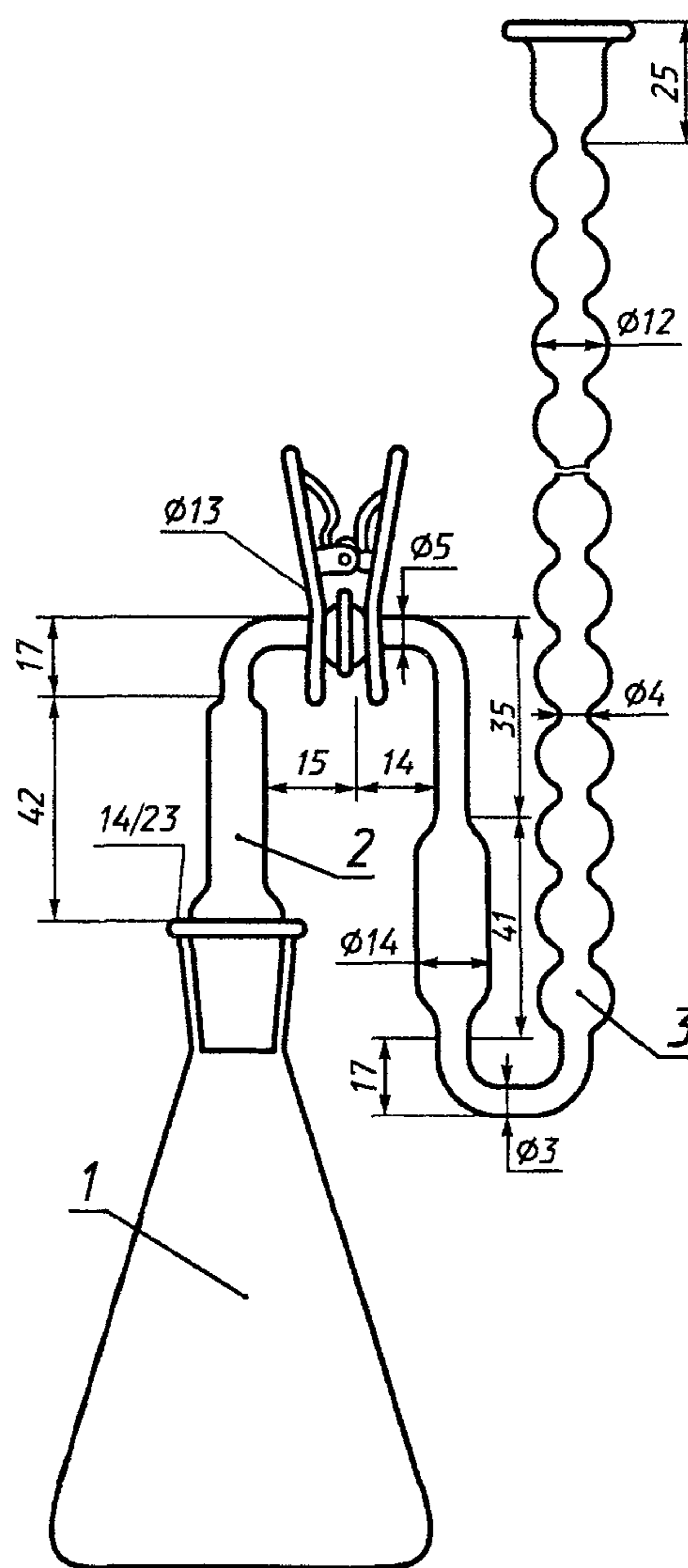
1 — коническая колба; 2 — соединительная трубка; 3 — абсорбер
