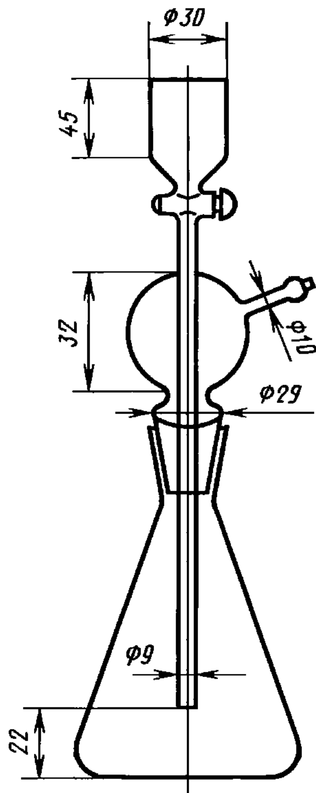
Прибор для растворения металлического олова
