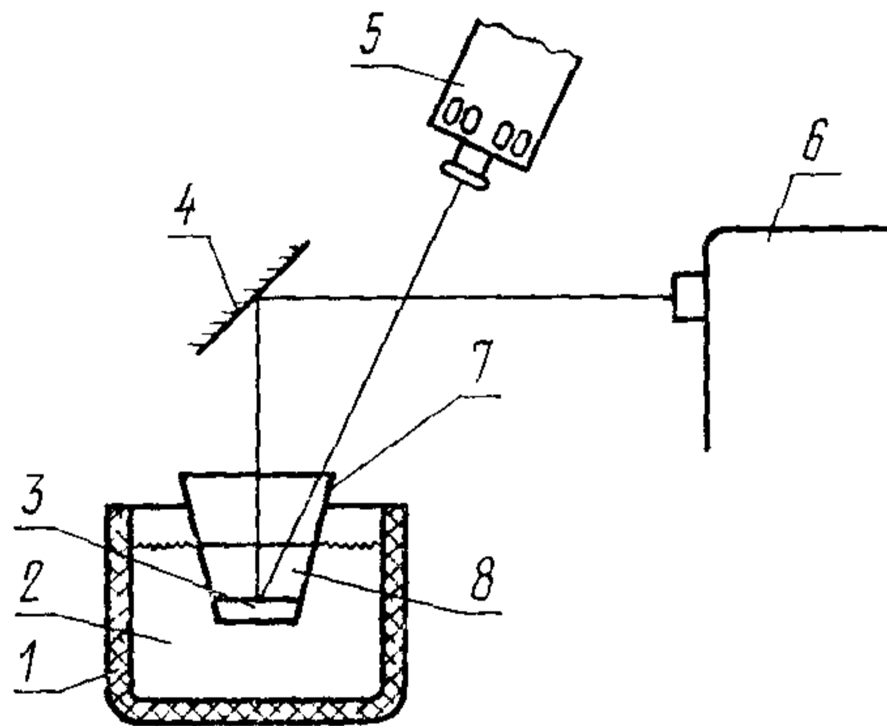
1—панопластовая чашка, 2—жидкий азот, 3—анализуемый раствор, 4—зеркало; 5—осветитель, 6—монохроматор; 7—платиновый тигель; 8—жидкий азот.
